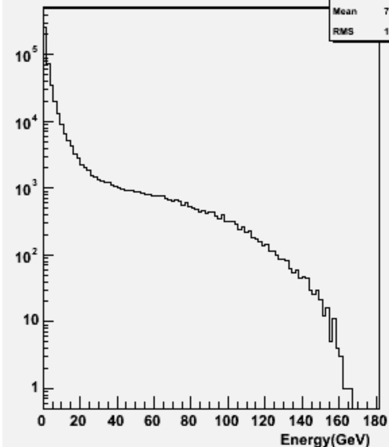
Start point R : w100813 e2e2n1e1sc_o
