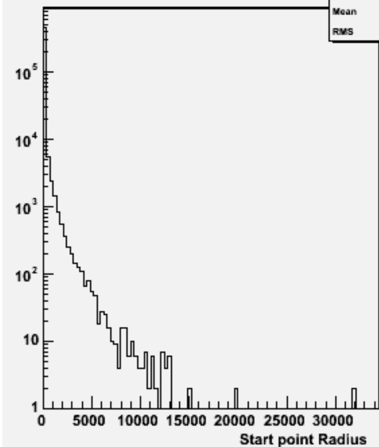
Start point R : w100813 e2e2n1e1sc_o
