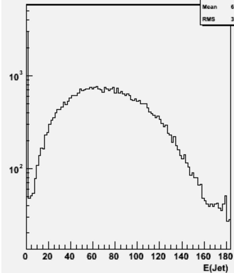
Jet energies(All jets)w100813 e2e2n1e1sc_o
