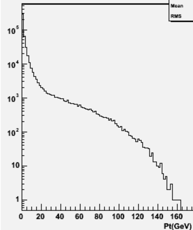
Start point Z : w100813 e2e2n1e1sc_o
