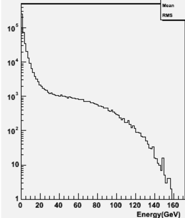
Particle Energy : w100812 e2e2n1e1sc_o
