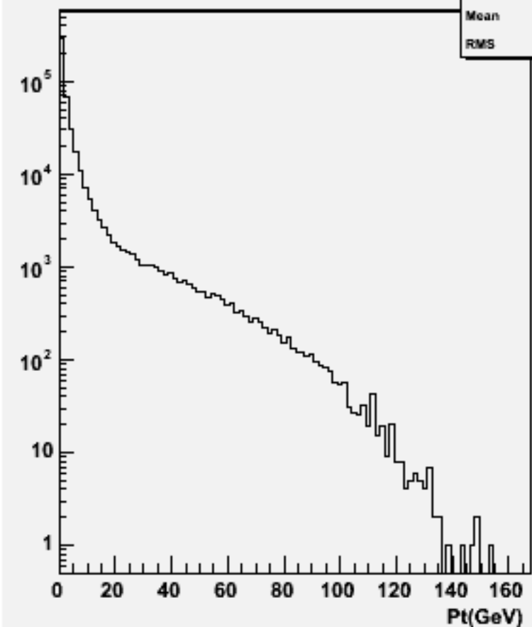
Particle Pt : w100812 e2e2n1e1sc_o
