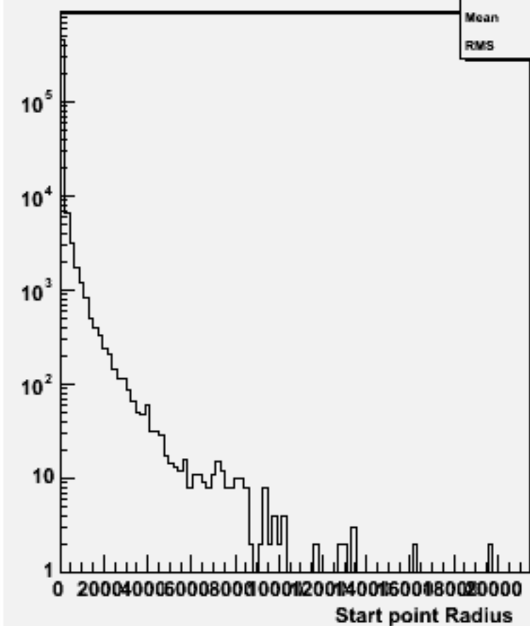
Start point R : w100812 e2e2n1e1sc_o
