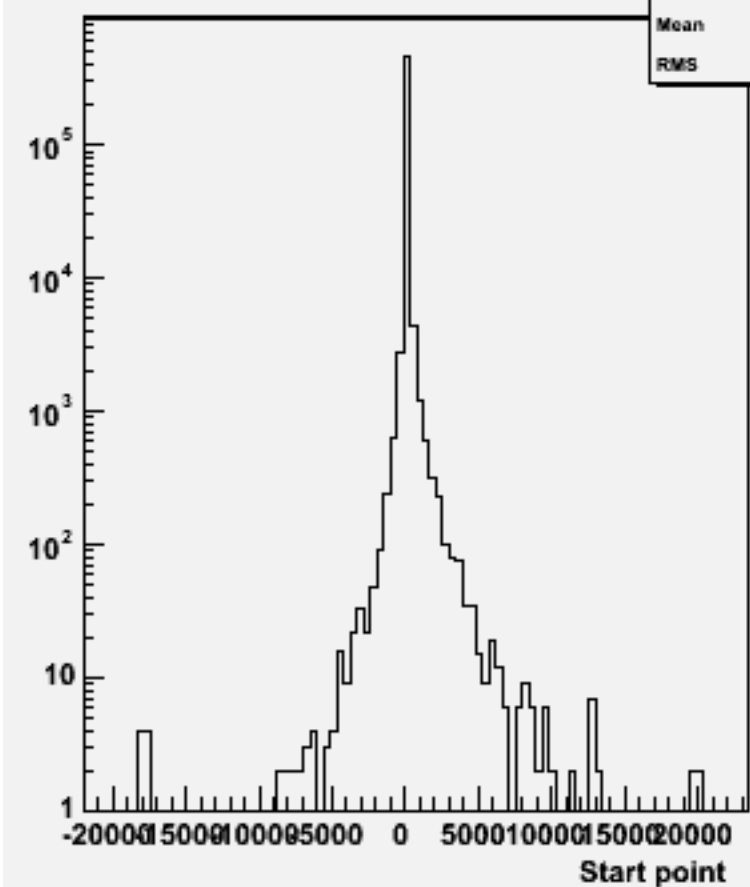
Start point Z : w100812 e2e2n1e1sc_o
