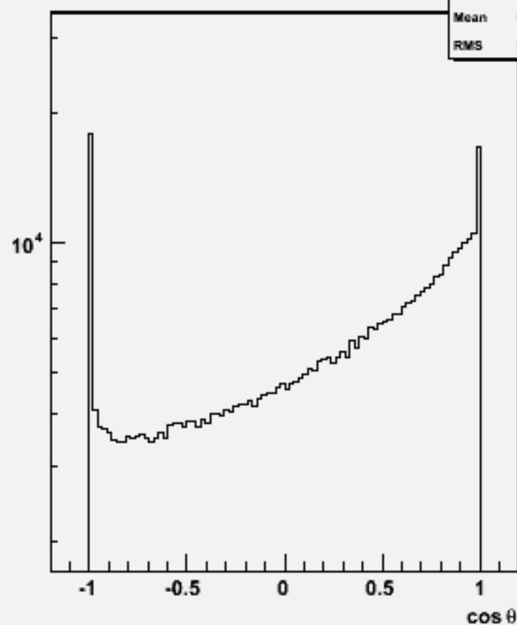
Particle cosθ : w100812 e2e2n1e1sc_o
