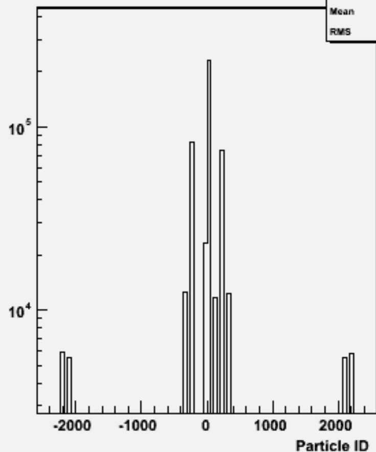
Particle ID : w100811 e2e2n1e1sc_o
