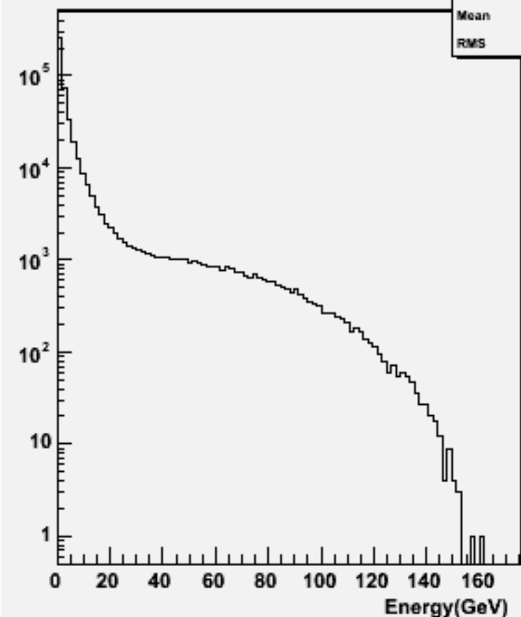
Particle Energy : w100811 e2e2n1e1sc_o
