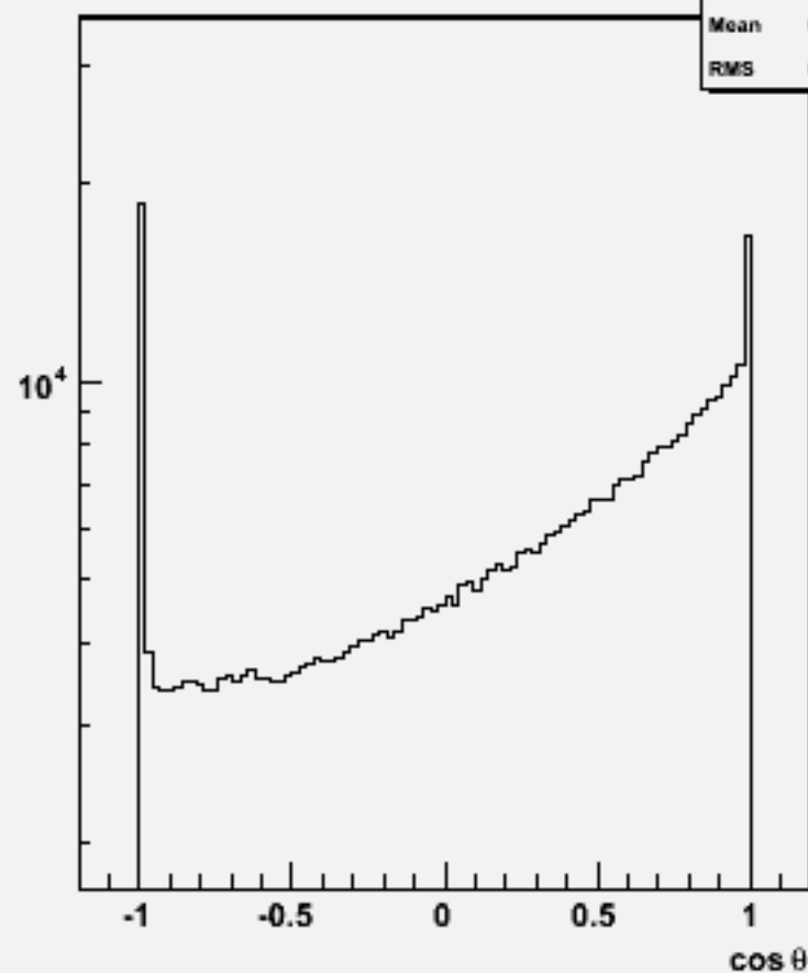
Particle cosθ : w100811 e2e2n1e1sc_o
