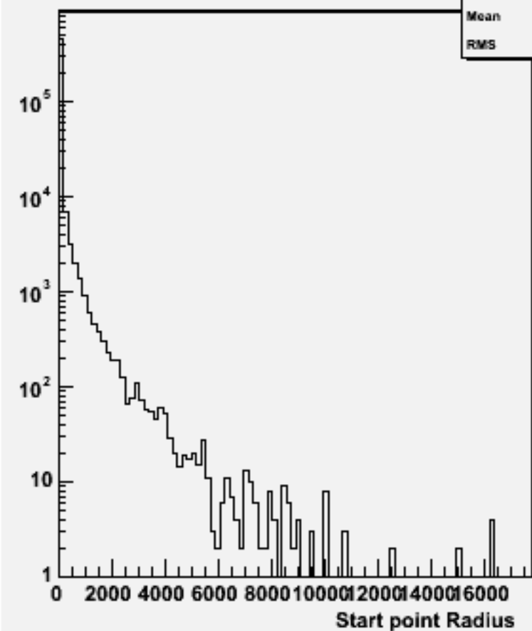
Start point R : w100811 e2e2n1e1sc_o
