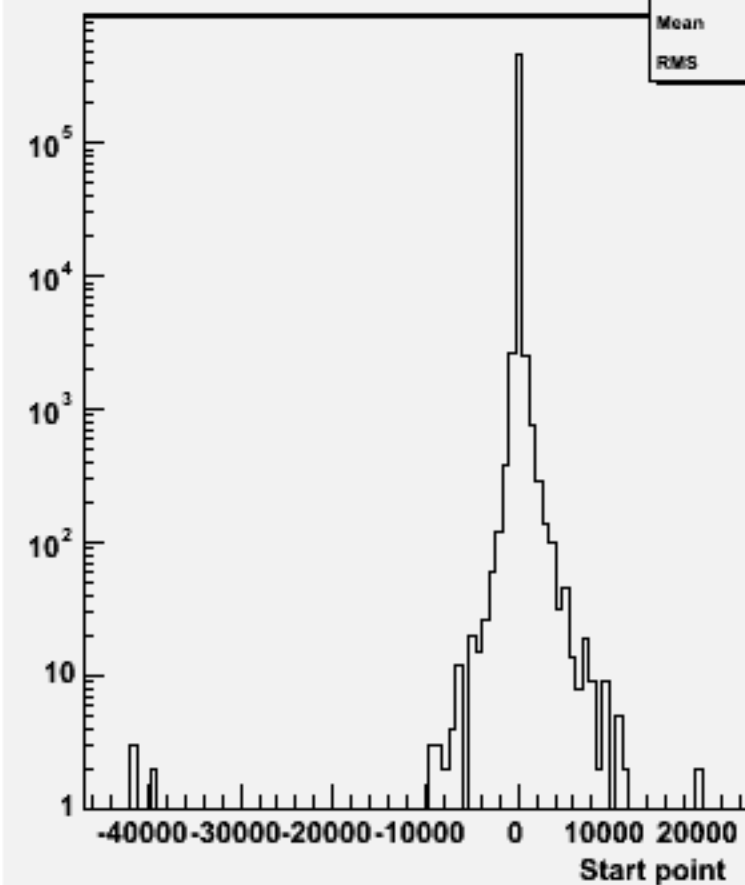
Start point Z : w100811 e2e2n1e1sc_o
