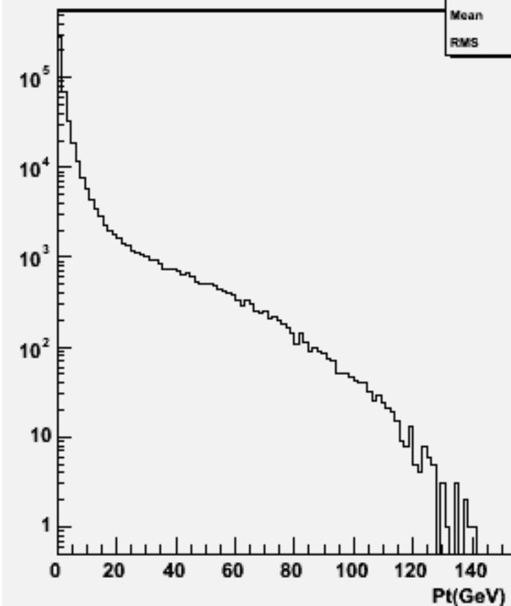
Particle Pt : w100811 e2e2n1e1sc_o
