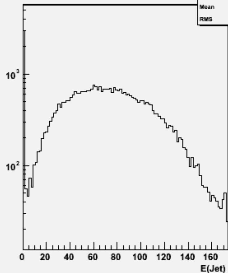
Jet energies(All jets)w100809 e2e2n1e1du_o
