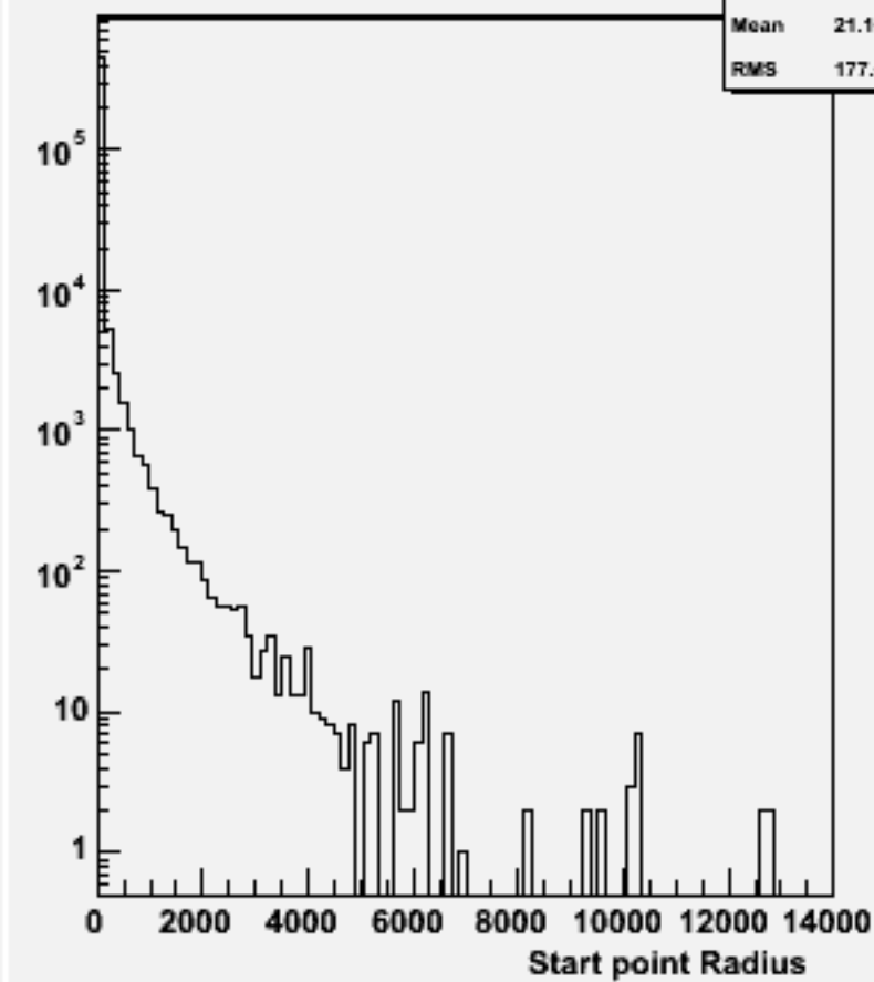
Start point R : w100809 e2e2n1e1du_o
