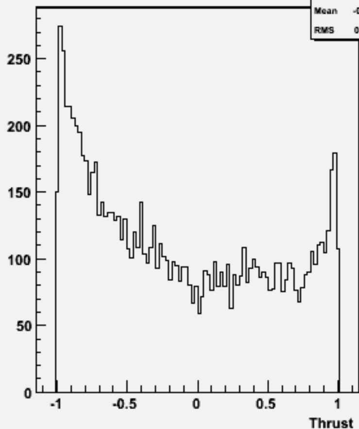
cos \Theta (thrust) w100809 e2e2n1e1du_o
