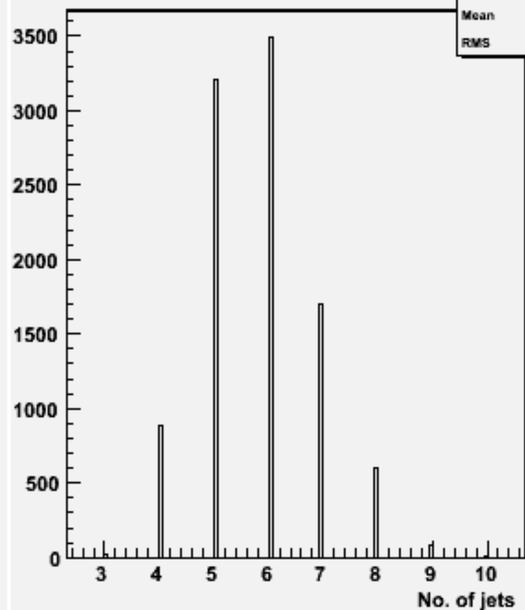
No. jets (ycut=0.001) : w100809 e2e2n1e1du_o
