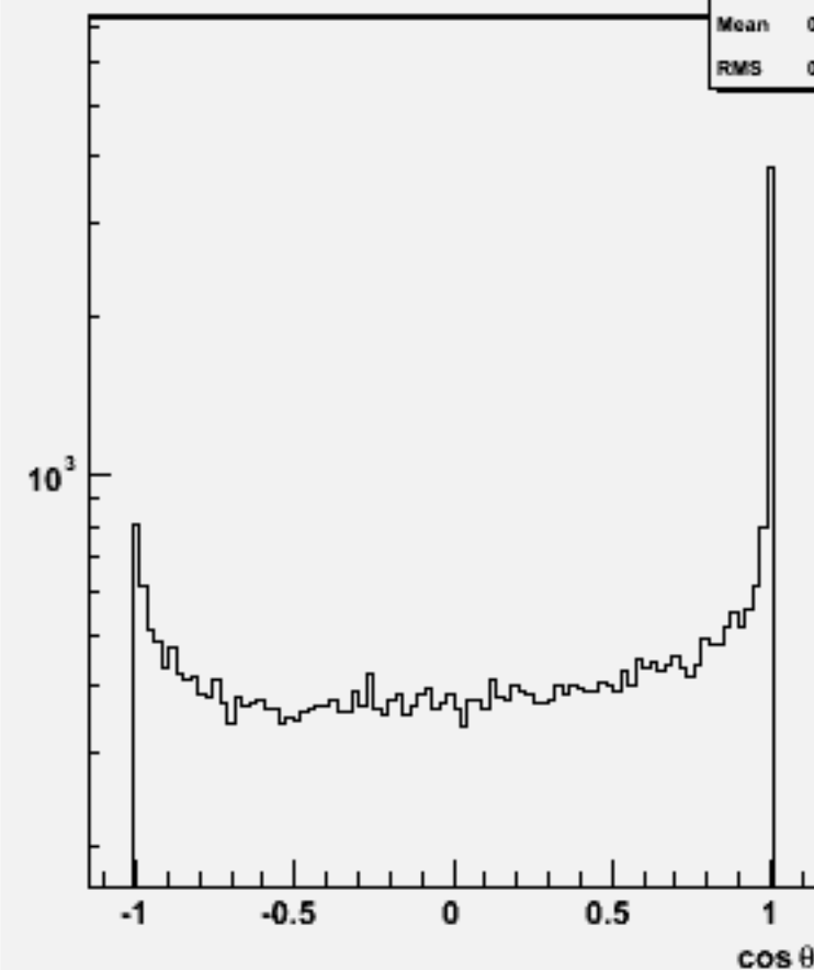
Jet cos \theta (All jets)w100809 e2e2n1e1du_o
