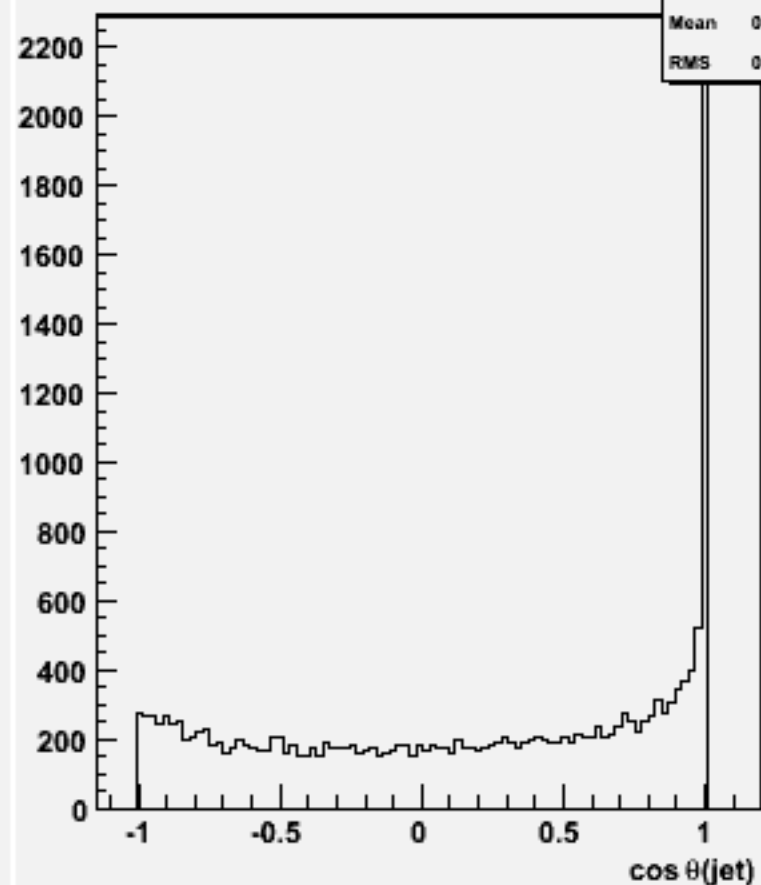
cos \theta for 2-jets :w100809 e2e2n1e1du_o
