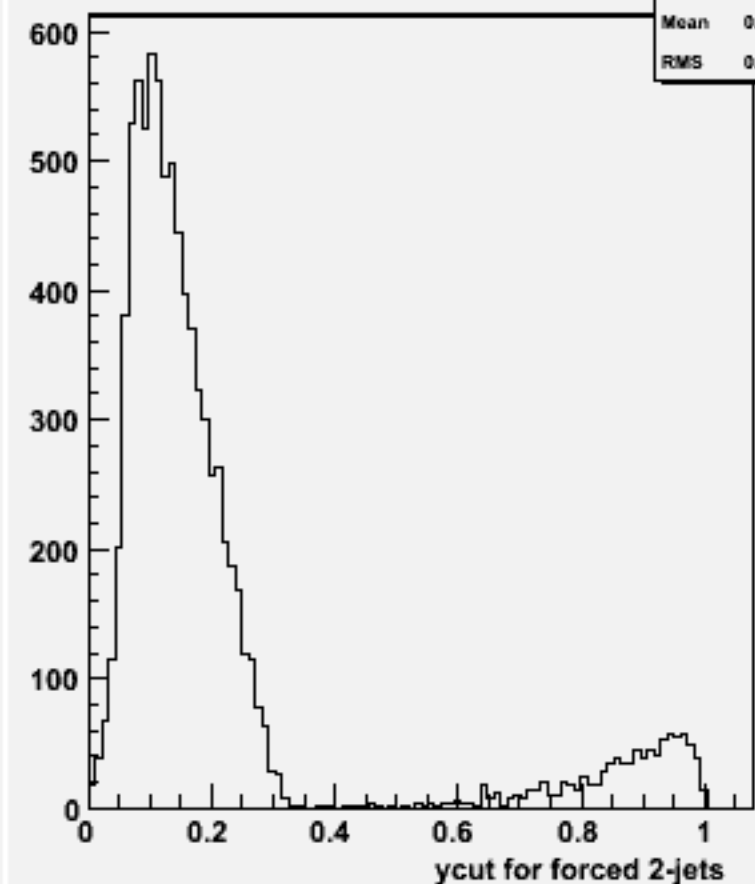
Ycut for 2-jets :w100809 e2e2n1e1du_o
