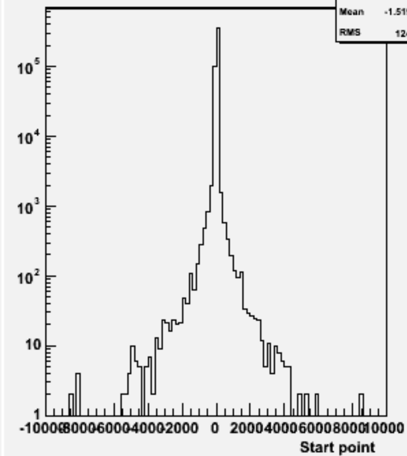
Start point Z : w100809 e2e2n1e1du_o
