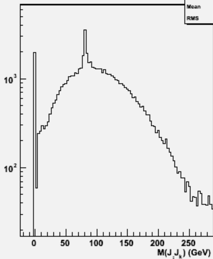
2jets mass(All comb)w100809 e2e2n1e1du_o
