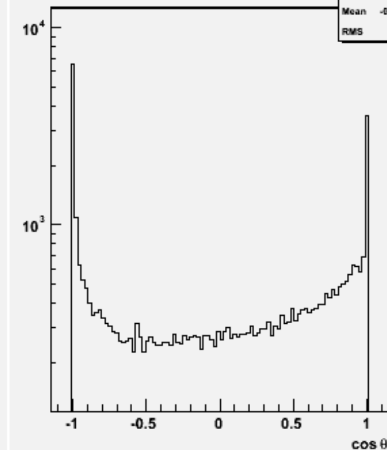
Jet cos \theta (All jets)w100807 e2e2n1e1du_o
