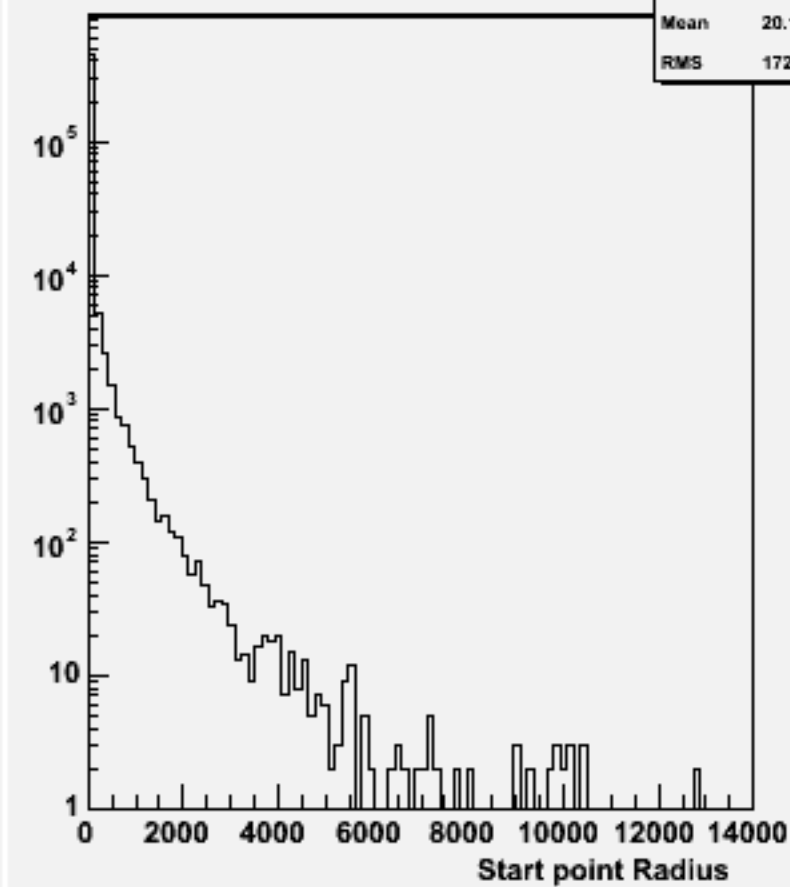
Start point R : w100807 e2e2n1e1du_o
