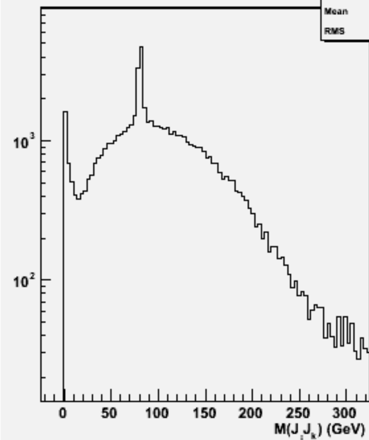
2jets mass(All comb)w100807 e2e2n1e1du_o
