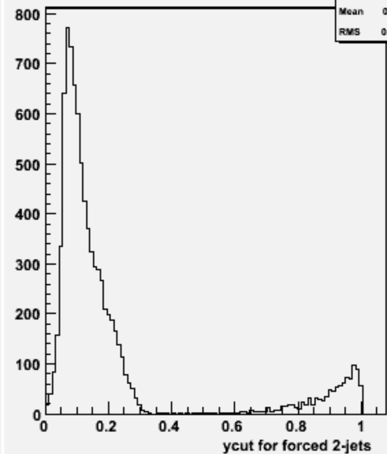
Ycut for 2-jets :w100807 e2e2n1e1du_o
