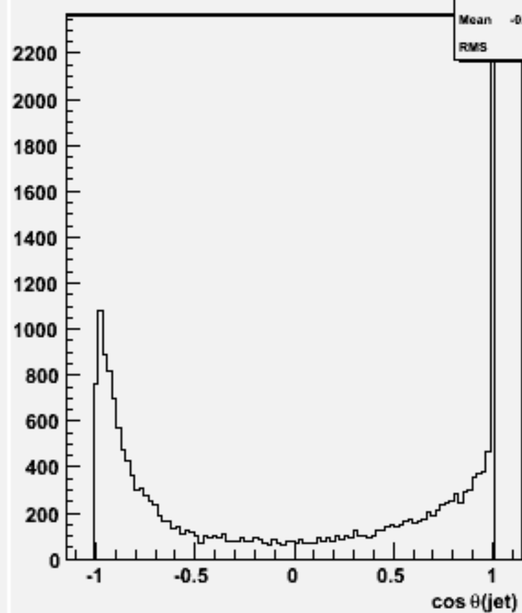
cos \theta for 2-jets :w100807 e2e2n1e1du_o
