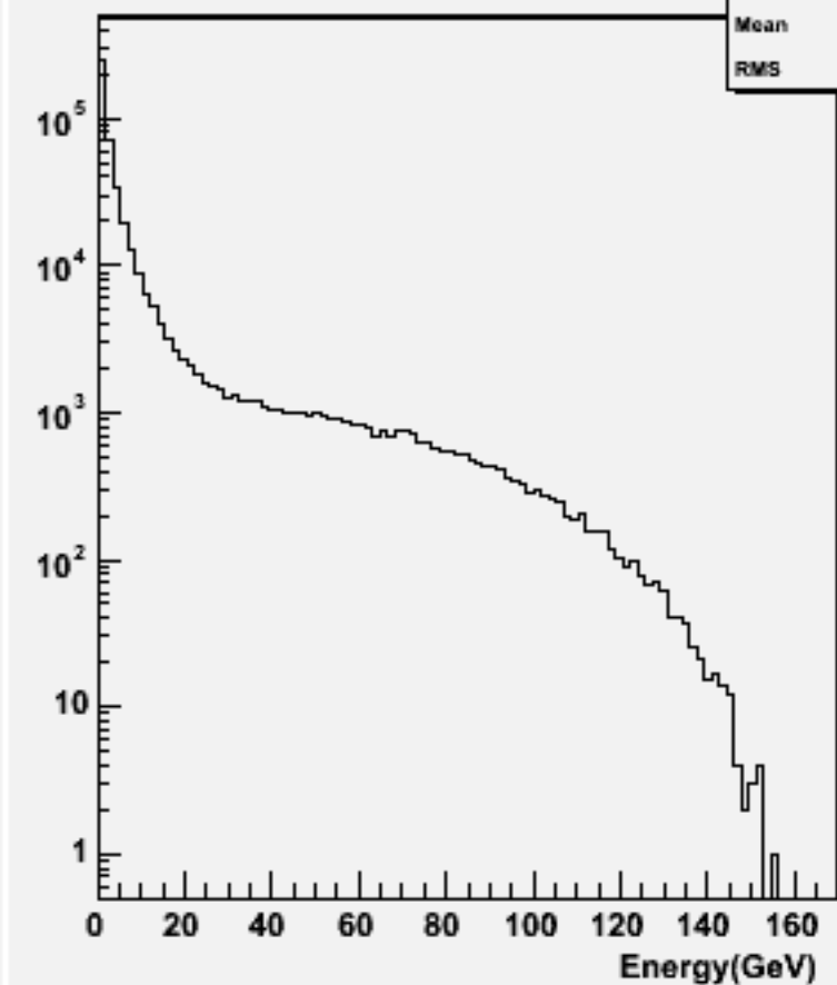
Start point R : w100807 e2e2n1e1du_o
