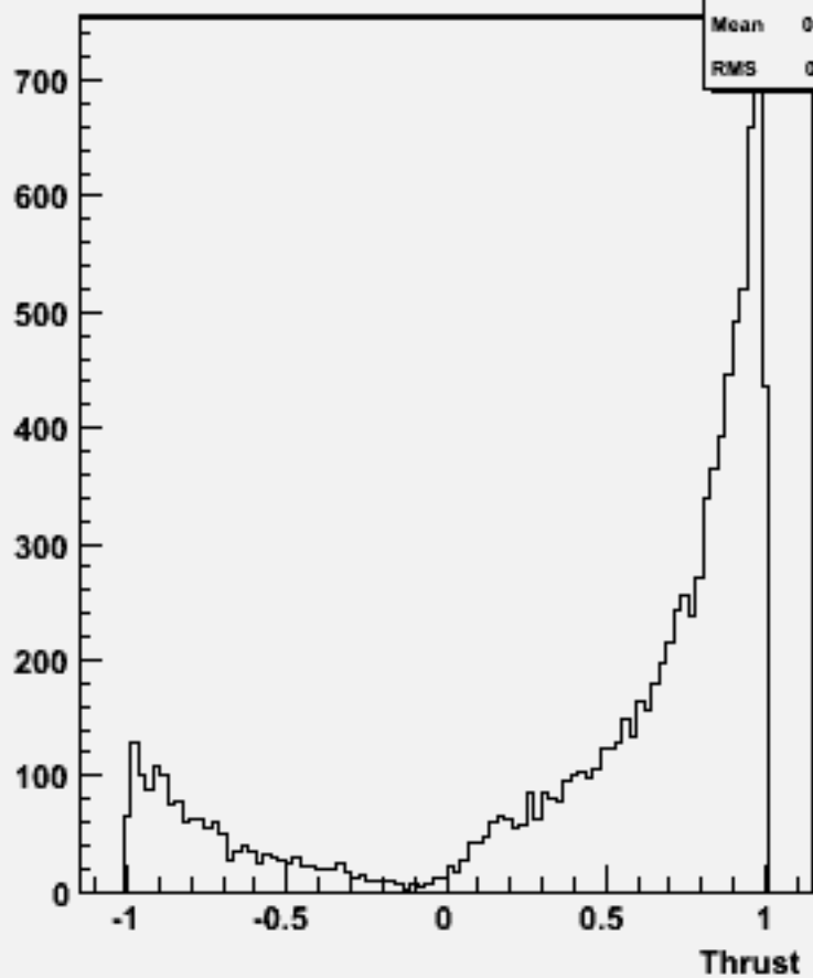
cos \Theta (thrust) w100807 e2e2n1e1du_o
