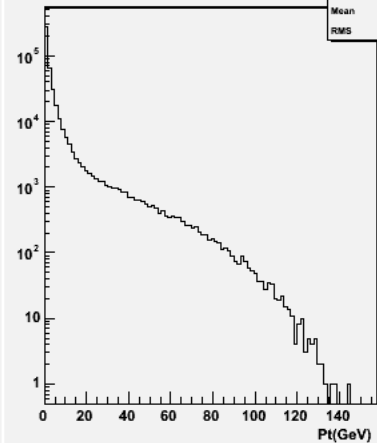
Start point Z : w100807 e2e2n1e1du_o
