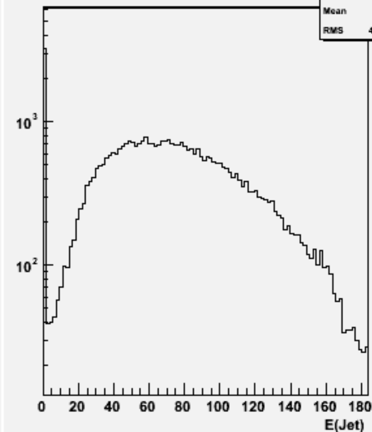
Jet energies(All jets)w100807 e2e2n1e1du_o
