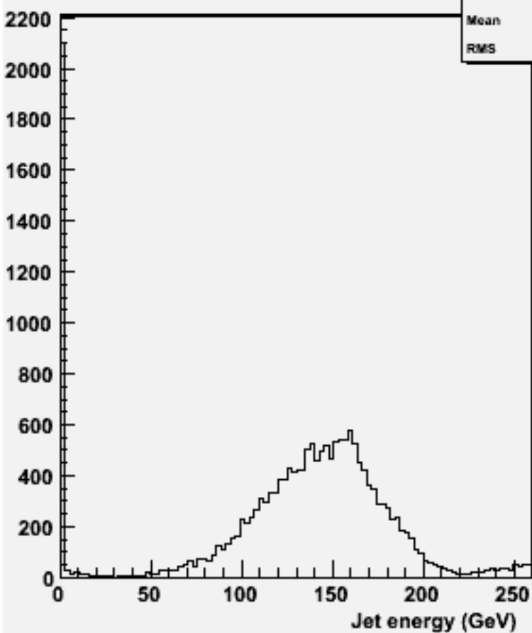
energy for 2-jets :w100807 e2e2n1e1du_o
