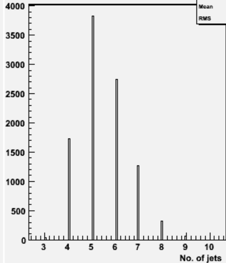
No. jets (ycut=0.001) : w100807 e2e2n1e1du_o
