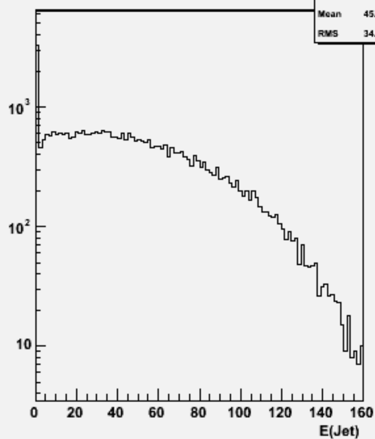
Jet energies(All jets)w100805 e2e2n1e1e3n3_o
