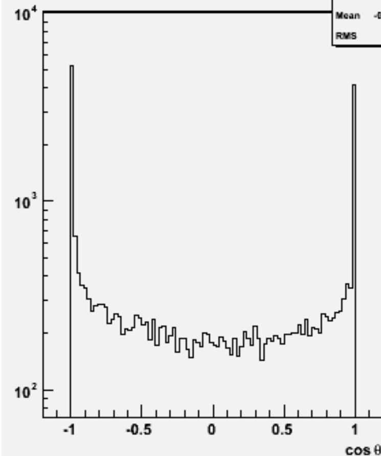
Jet cos \theta (All jets)w100804 e2e2n1e1e3n3_o
