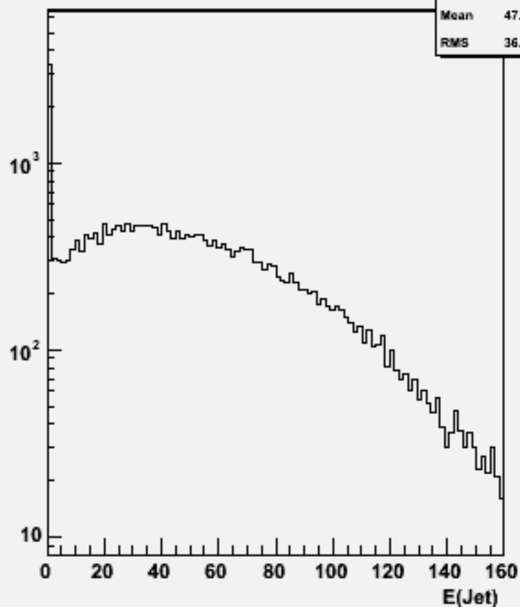
Jet energies(All jets)w100804 e2e2n1e1e3n3_o
