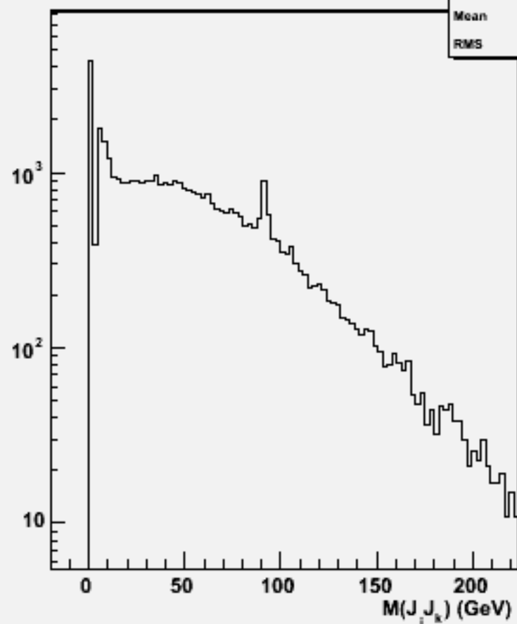
2jets mass(All comb)w100804 e2e2n1e1e3n3_o
