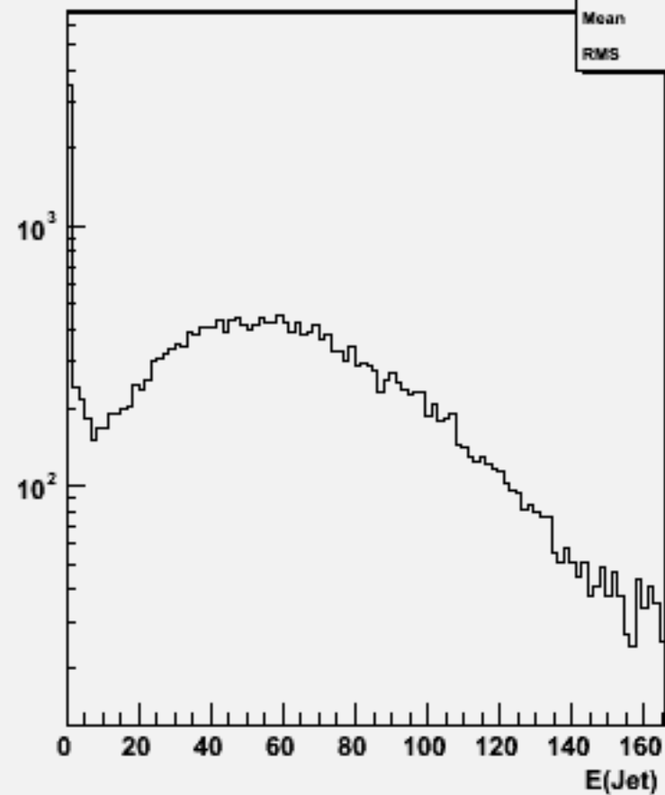
Jet energies(All jets)w100796 e2e2n1e1e1n1_o
