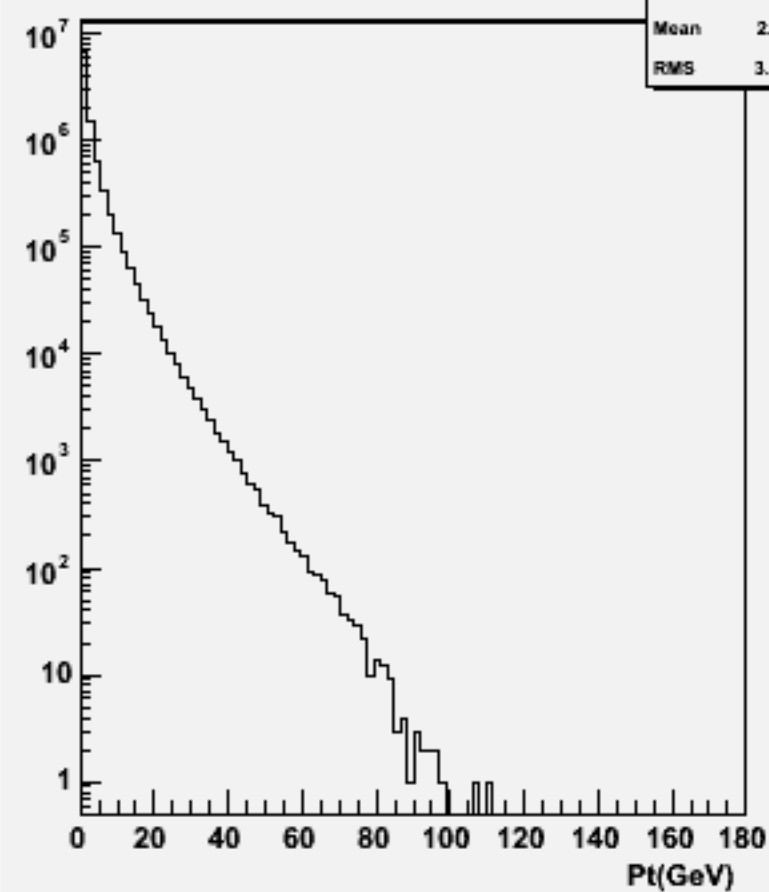
Particle Pt : w100794 e1e1cssc_o
