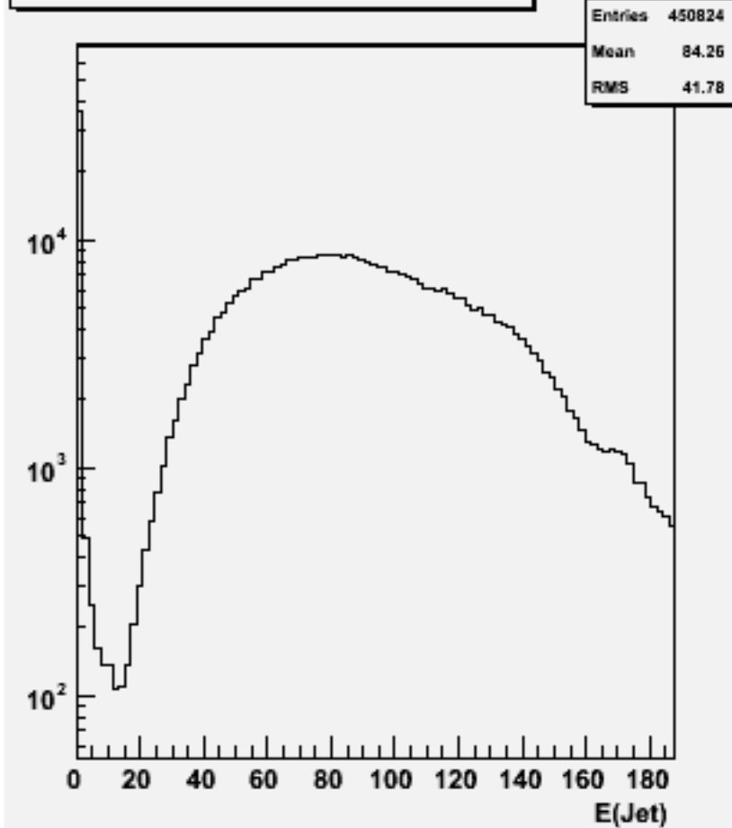
Jet energies(All jets)w100794 e1e1cssc_o
