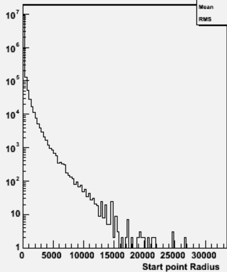
Start point R : w100794 e1e1cssc_o
