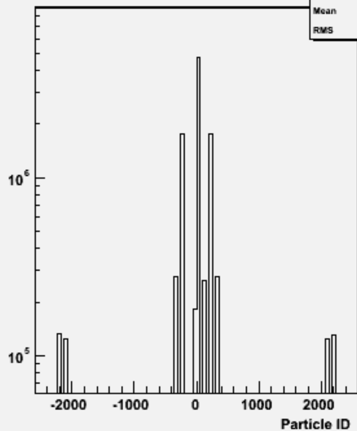
Particle ID : w100794 e1e1cssc_o
