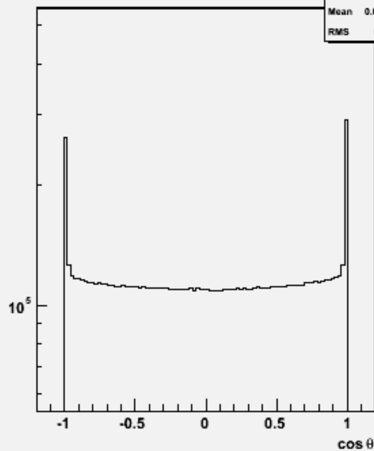
Particle cos \theta : w100794 e1e1cssc_o
