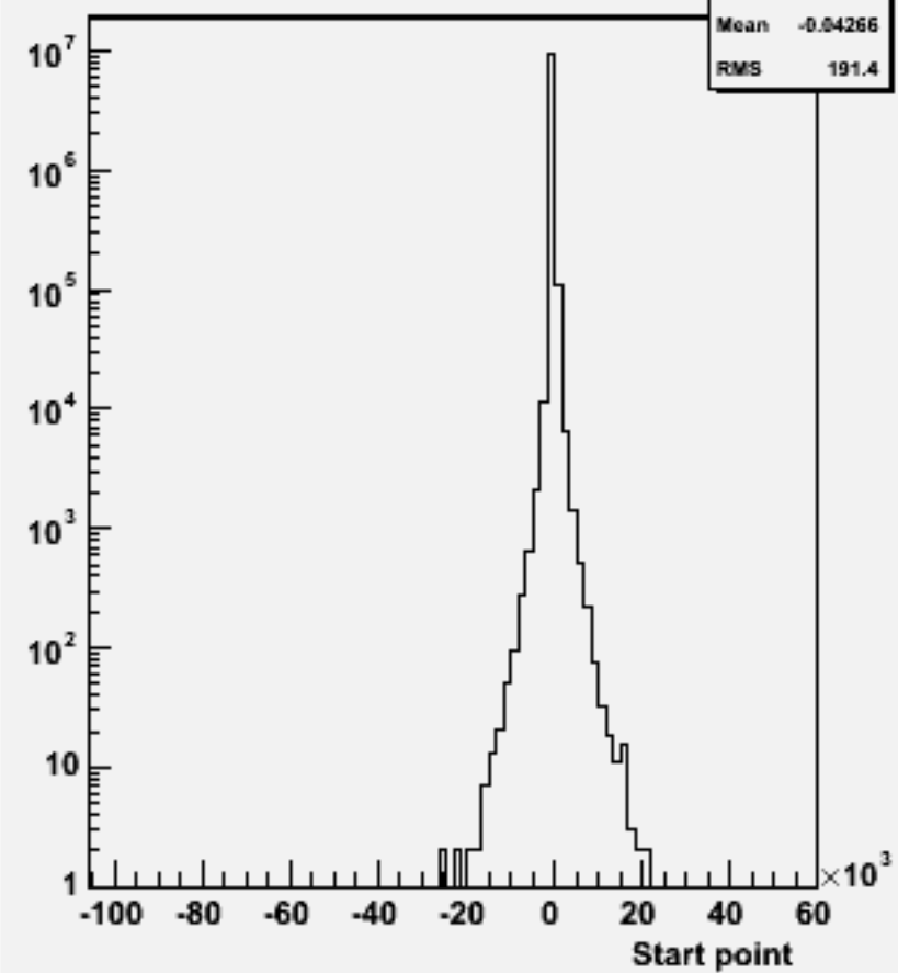
Start point Z : w100794 e1e1cssc_o
