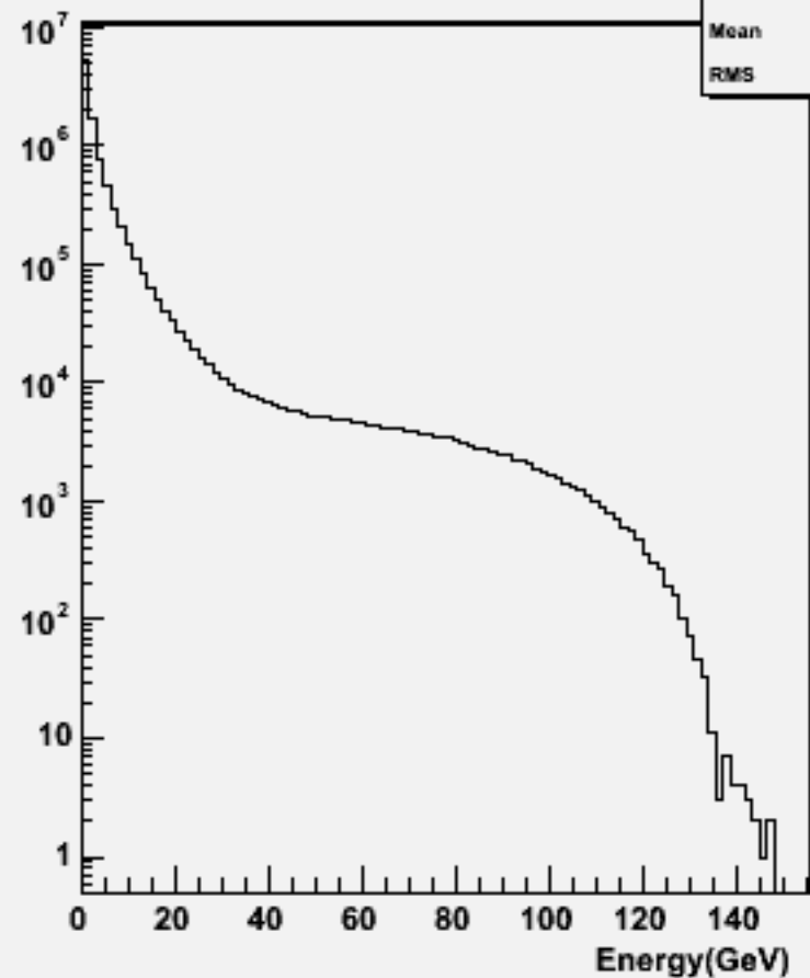
Particle Energy : w100794 e1e1cssc_o
