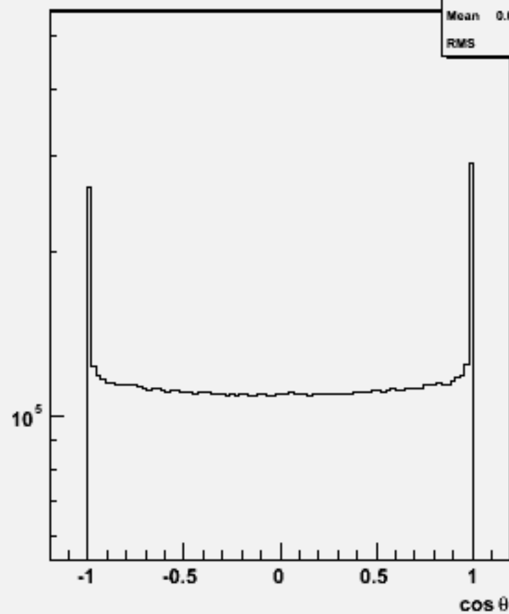
Particle cos \theta : w100793 e1e1cssc_o
