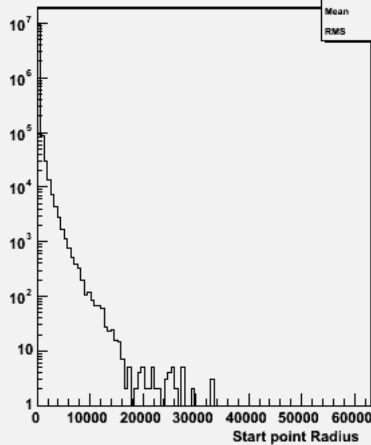
Start point R : w100793 e1e1cssc_o
