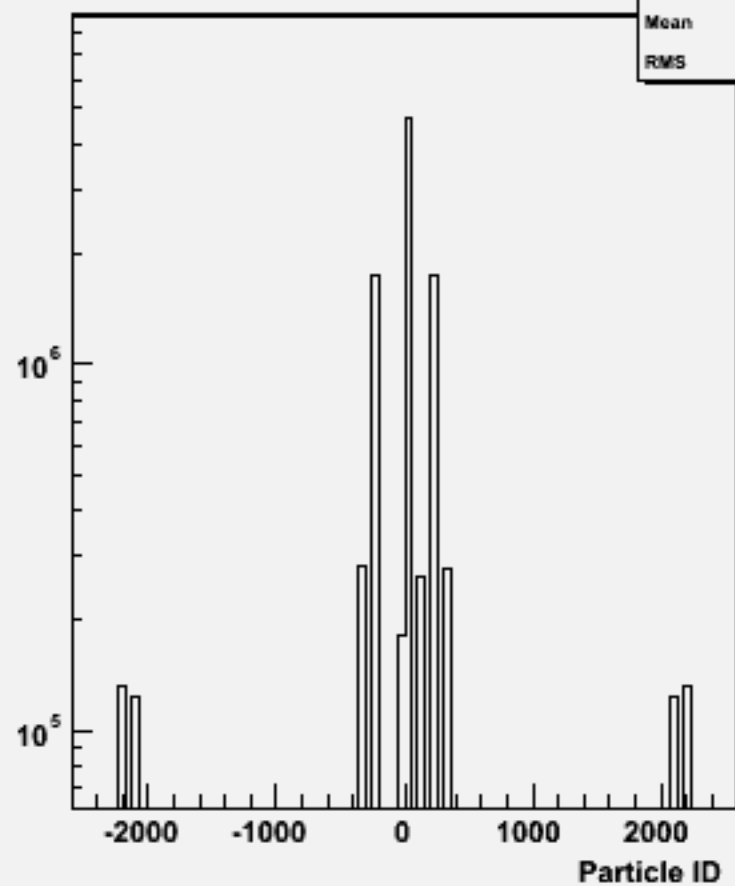
Particle ID : w100793 e1e1cssc_o
