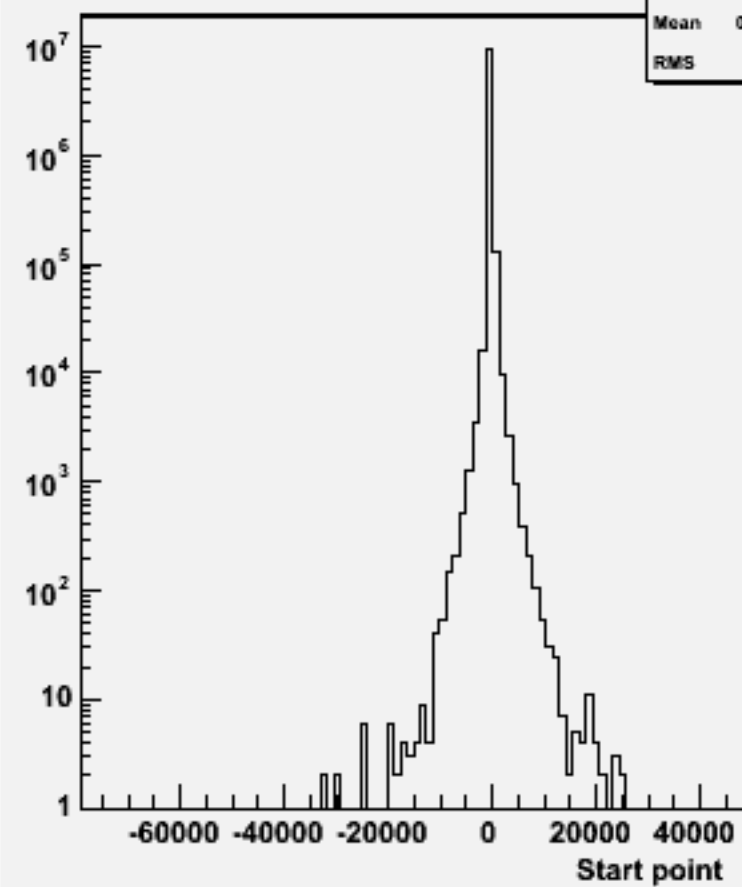
Start point Z : w100793 e1e1cssc_o
