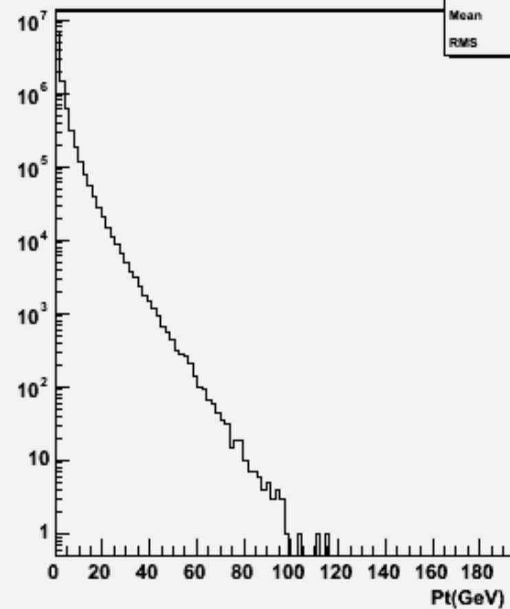
Particle Pt : w100793 e1e1cssc_o
