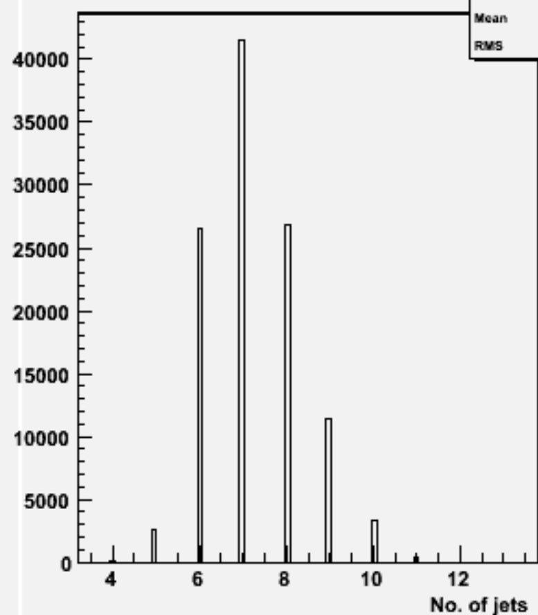
No. jets (ycut=0.001) : w100793 e1e1cssc_o
