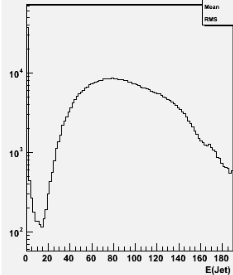
Jet energies(All jets)w100793 e1e1cssc_o
