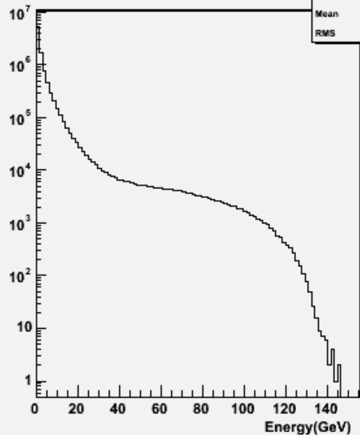
Particle Energy : w100793 e1e1cssc_o
