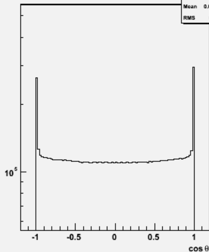
Particle cos \theta : w100790 e1e1csdu_o
