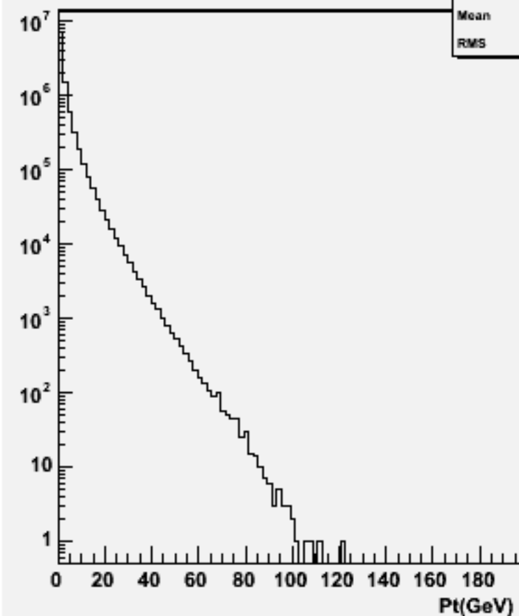
Particle Pt : w100790 e1e1csdu_o
