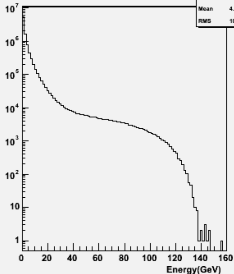
Particle Energy : w100790 e1e1csdu_o
