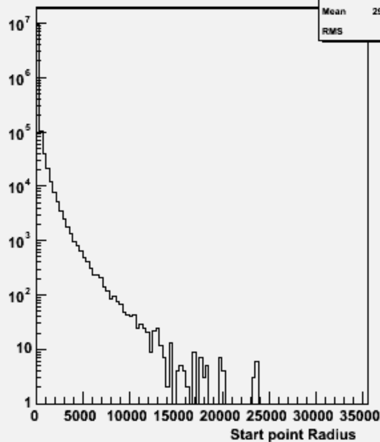
Start point R : w100790 e1e1csdu_o
