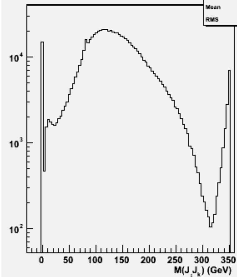
2jets mass(All comb)w100790 e1e1csdu_o
