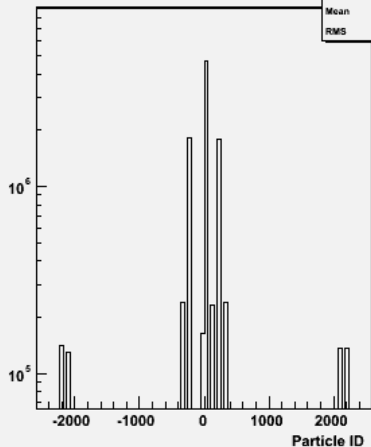
Particle ID : w100790 e1e1csdu_o
