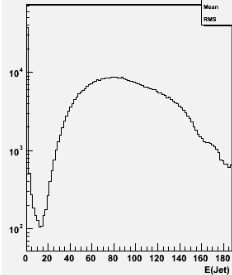
Jet energies(All jets)w100790 e1e1csdu_o
