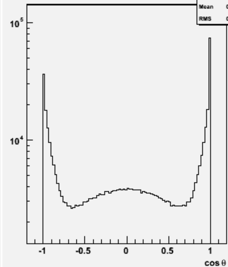
Jet cosθ (All jets)w100790 e1e1csdu_o
