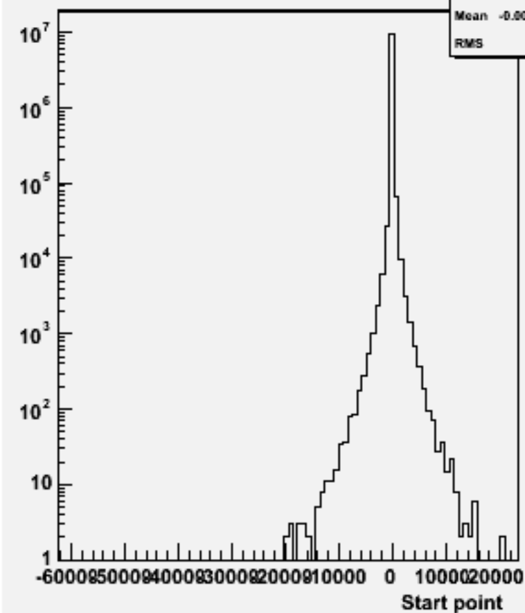
Start point Z : w100790 e1e1csdu_o
