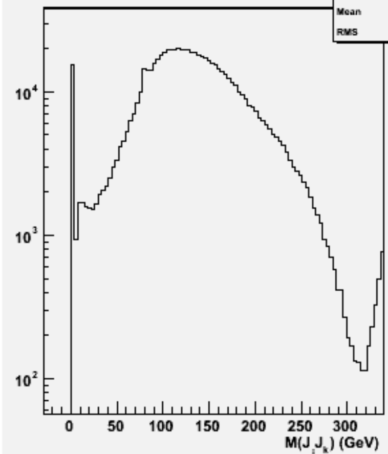
2jets mass(All comb)w100788 e1e1csdu_o
