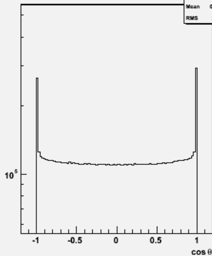
Particle cos \theta : w100788 e1e1csdu_o
