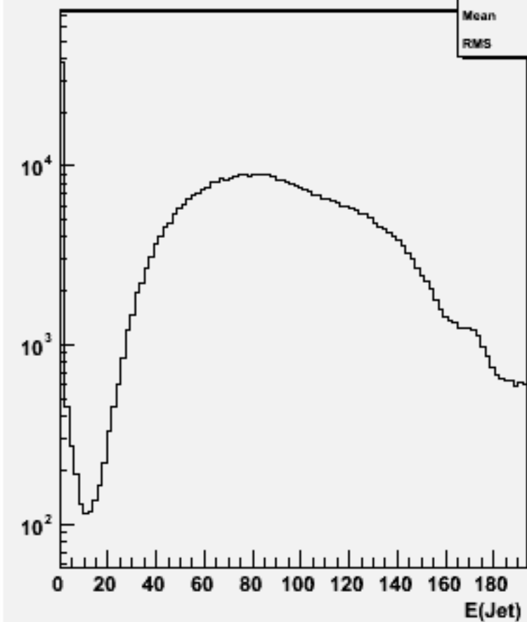
Jet energies(All jets)w100788 e1e1csdu_o
