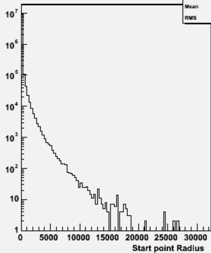
Start point R : w100788 e1e1csdu_o
