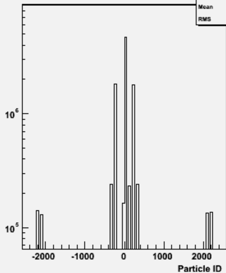
Particle ID : w100788 e1e1csdu_o
