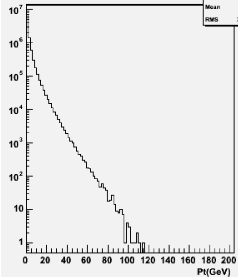
Particle Pt : w100788 e1e1csdu_o
