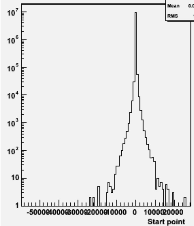
Start point Z : w100788 e1e1csdu_o
