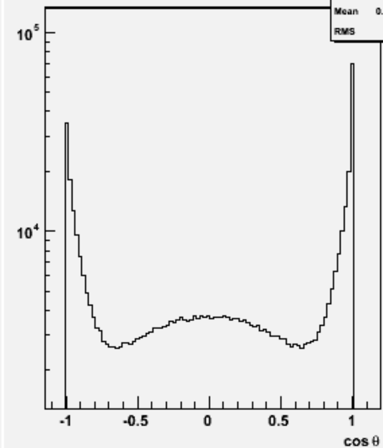
Jet cosθ (All jets)w100788 e1e1csdu_o
