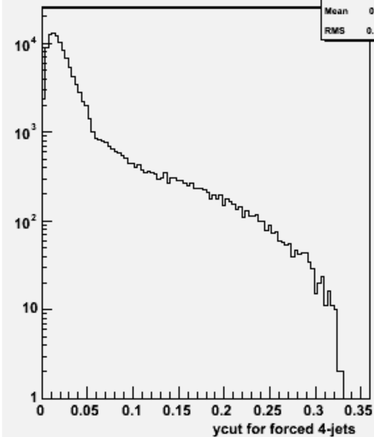
Ycut for 4-jets :w100788 e1e1csdu_o
