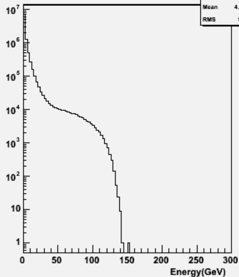
Particle Energy : w100788 e1e1csdu_o
