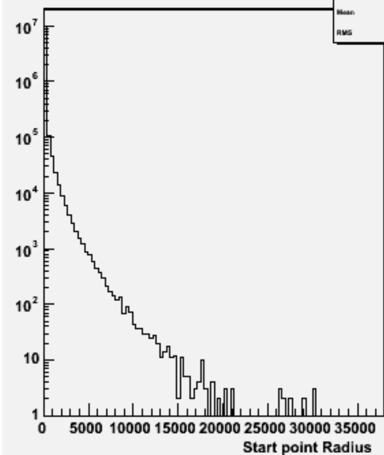
Start point R : w100783 e1e1cse3n3_o
