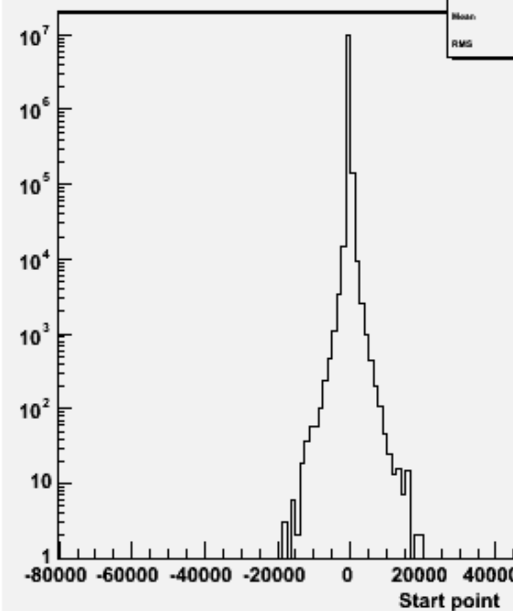
Start point Z : w100783 e1e1cse3n3_o
