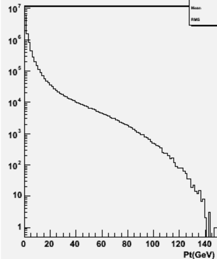
Particle Pt : w100783 e1e1cse3n3_o
