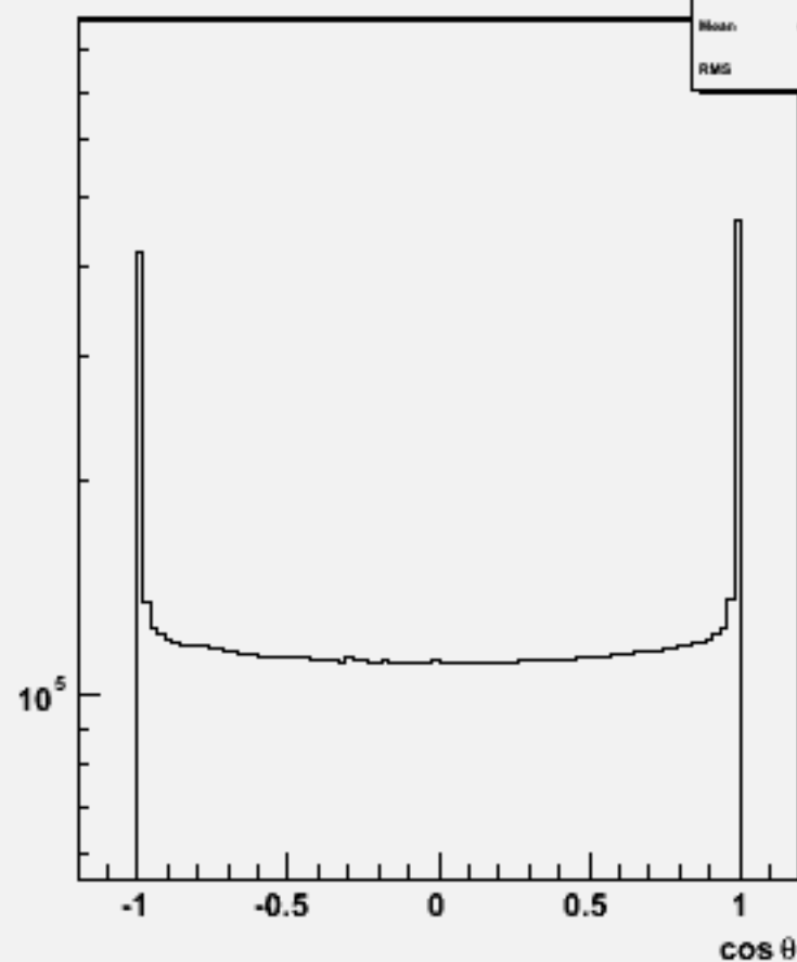
Particle \cos\theta : w100783 e1e1cse3n3_o
