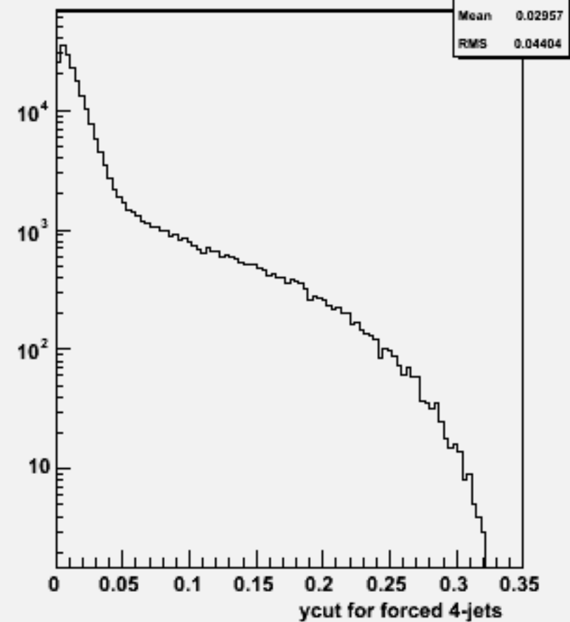
Ycut for 4-jets :w100782 e1e1cse2n2_o
