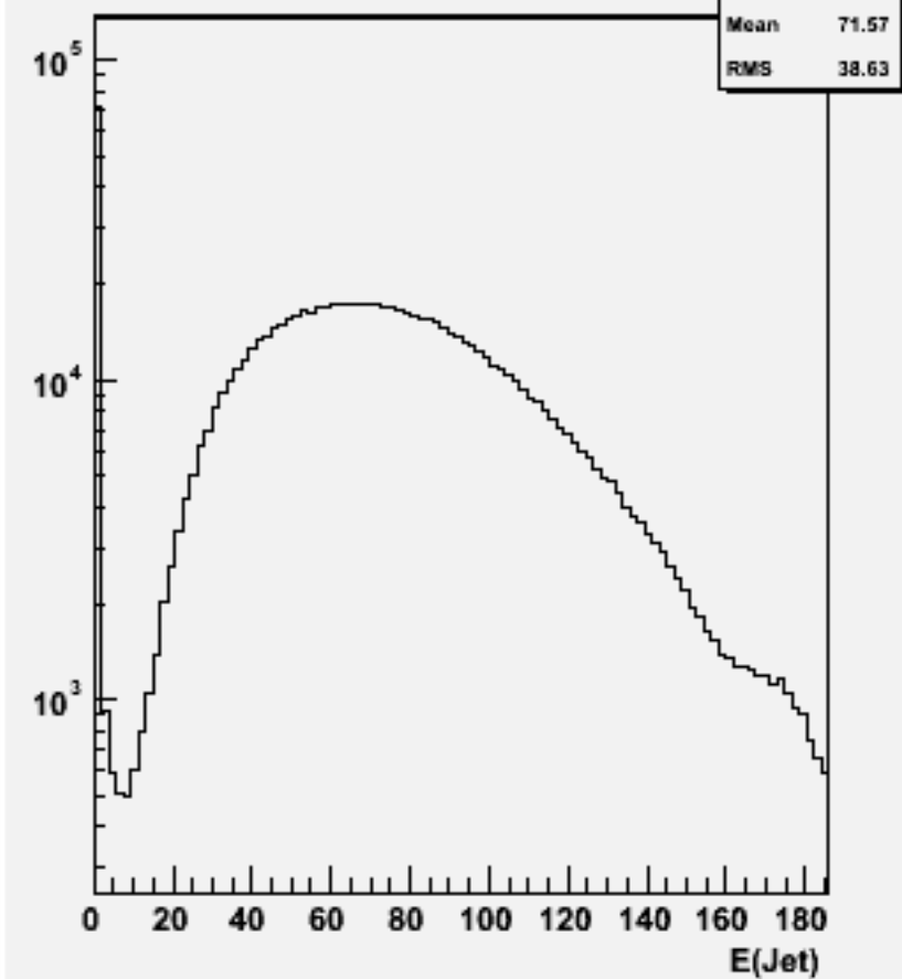
Jet energies(All jets)w100782 e1e1cse2n2_o
