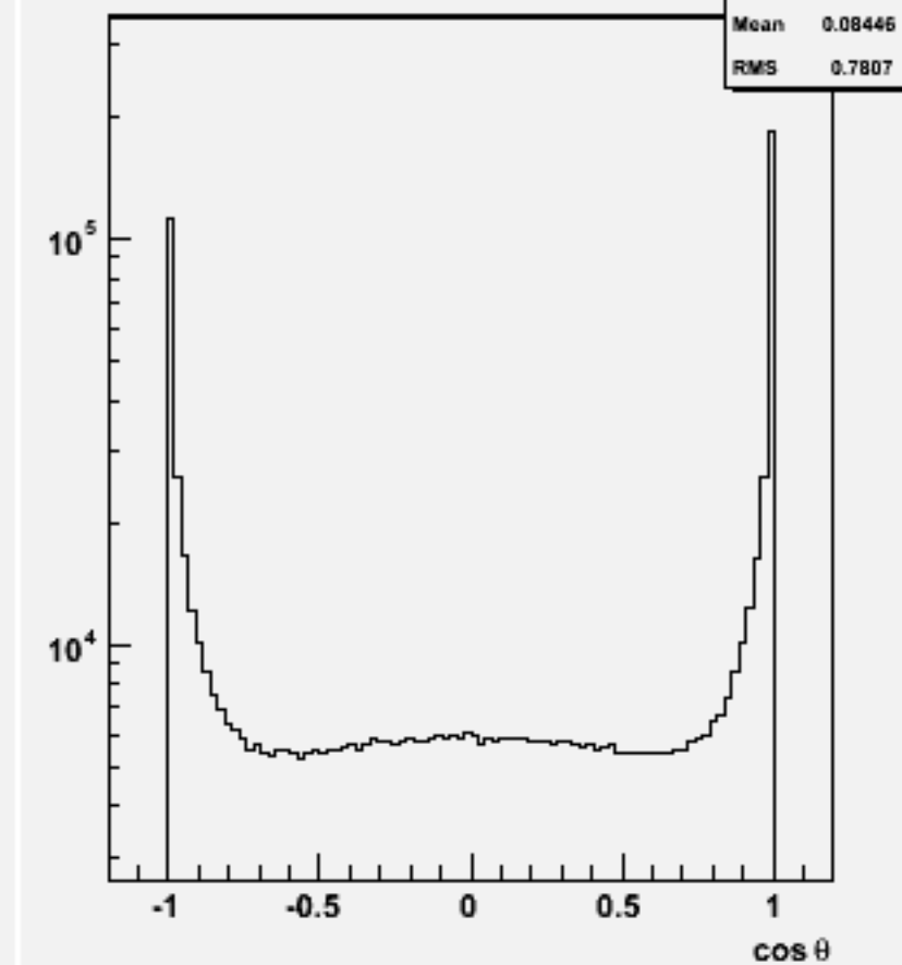
Jet cos \theta (All jets)w100782 e1e1cse2n2_o
