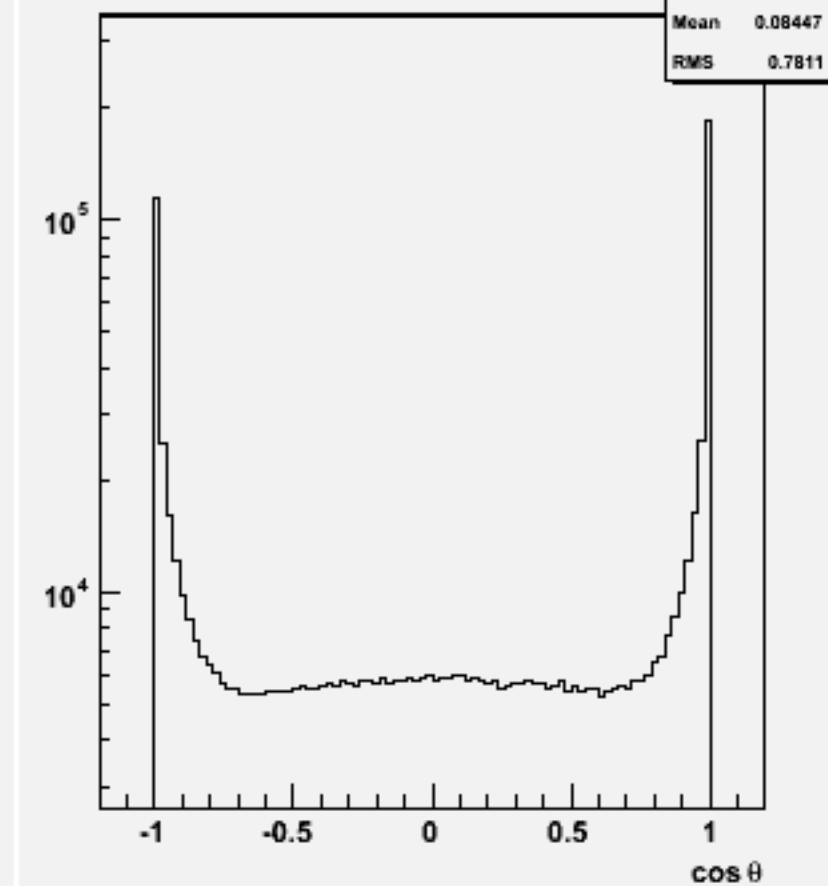
Jet cos \theta (All jets)w100781 e1e1cse2n2_o
