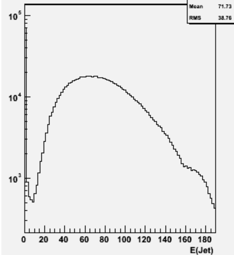
Jet energies(All jets)w100781 e1e1cse2n2_o
