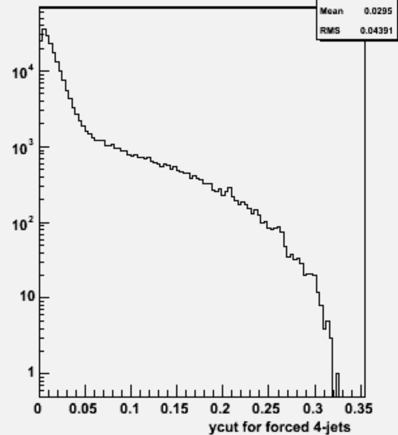
Ycut for 4-jets :w100781 e1e1cse2n2_o
