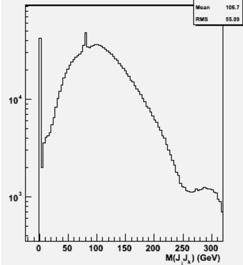
2jets mass(All comb)w100781 e1e1cse2n2_o
