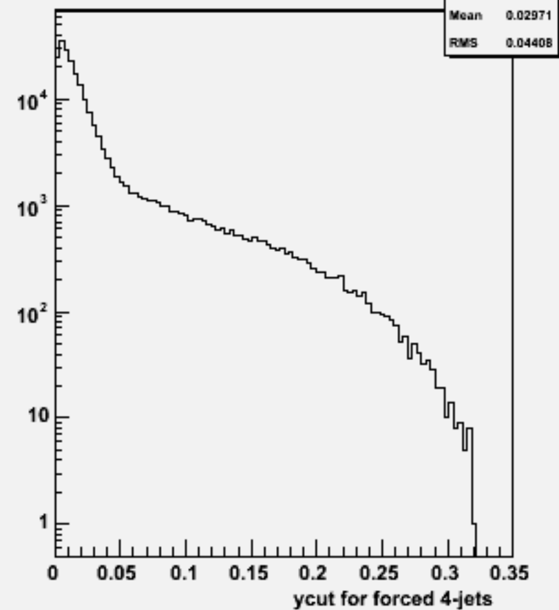
Ycut for 4-jets :w100780 e1e1cse2n2_o
