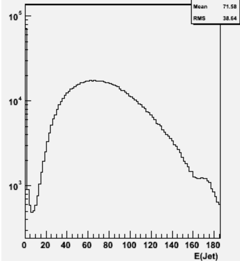
Jet energies(All jets)w100780 e1e1cse2n2_o
