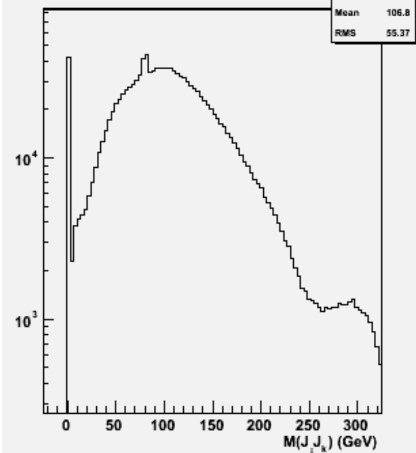
2jets mass(All comb)w100780 e1e1cse2n2_o
