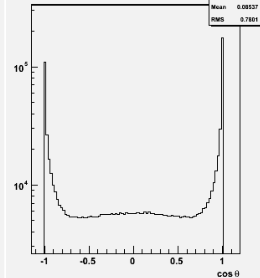
Jet cos \theta (All jets)w100780 e1e1cse2n2_o
