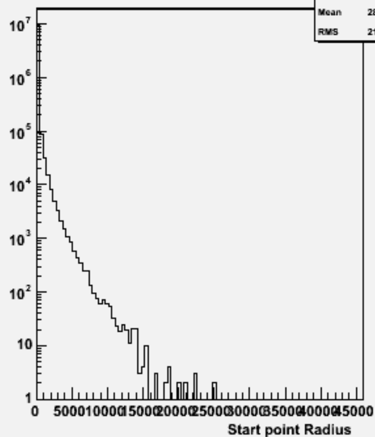
Start point R : w100774 e1e1udsc_o
