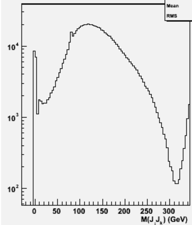
2jets mass(All comb)w100774 e1e1udsc_o
