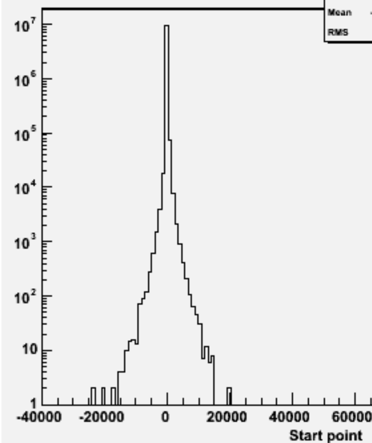
Start point Z : w100774 e1e1udsc_o
