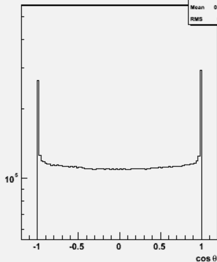
Particle cos \theta : w100774 e1e1udsc_o
