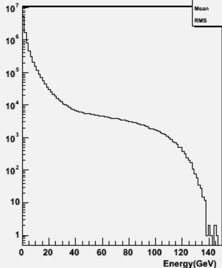
Particle Energy : w100774 e1e1udsc_o
