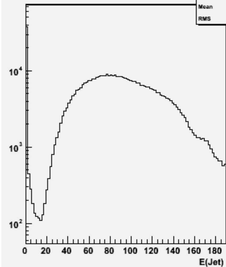
Jet energies(All jets)w100774 e1e1udsc_o
