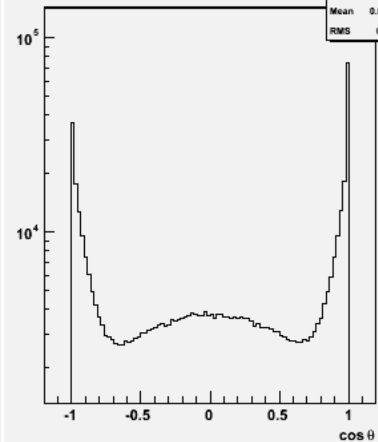
Jet cosθ (All jets)w100774 e1e1udsc_o
