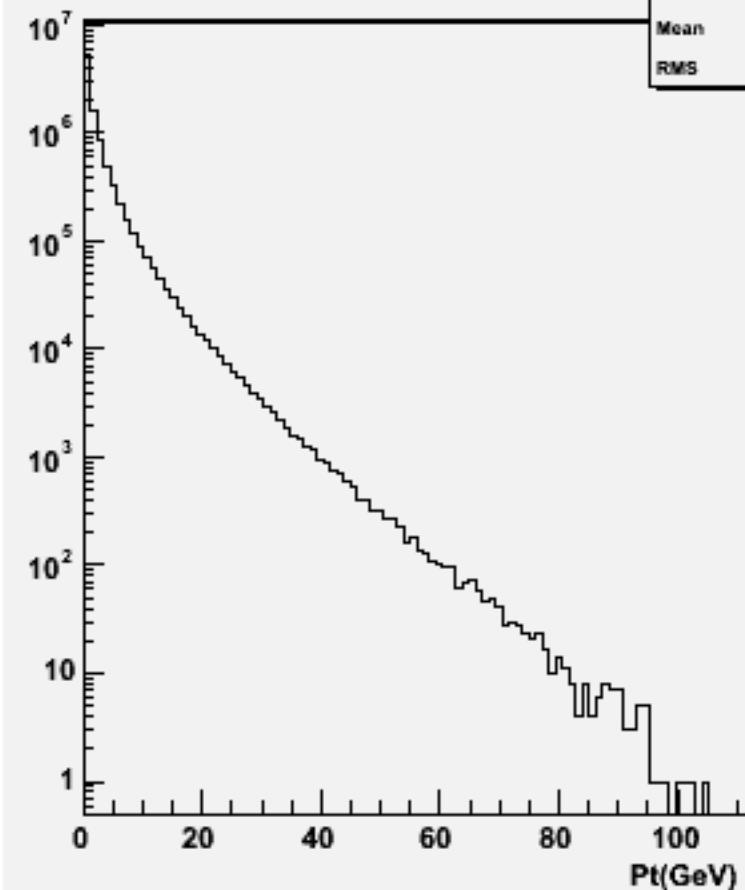
Particle Pt : w100774 e1e1udsc_o
