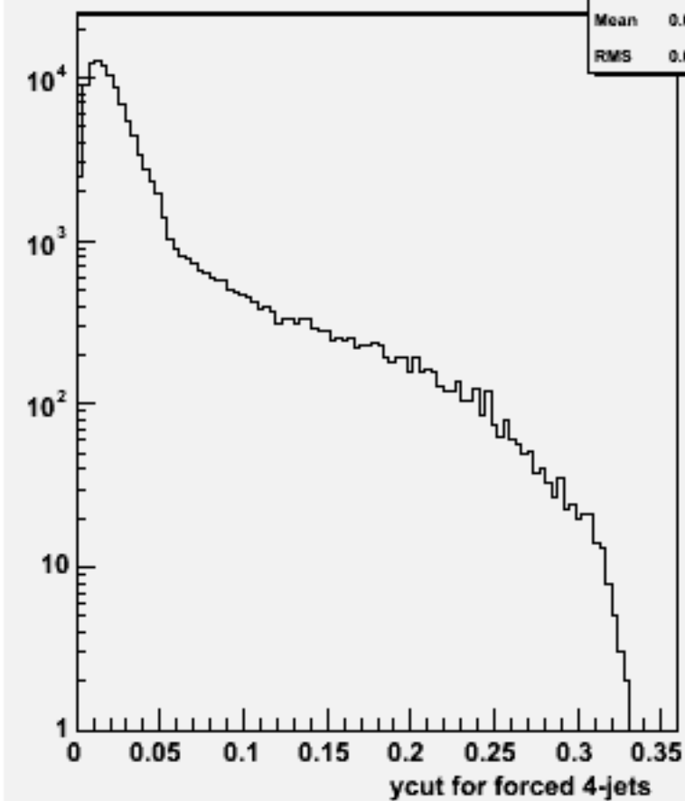
Ycut for 4-jets :w100774 e1e1udsc_o
