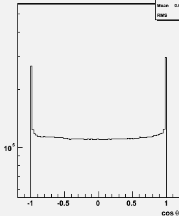
Particle cos \theta : w100773 e1e1udsc_o
