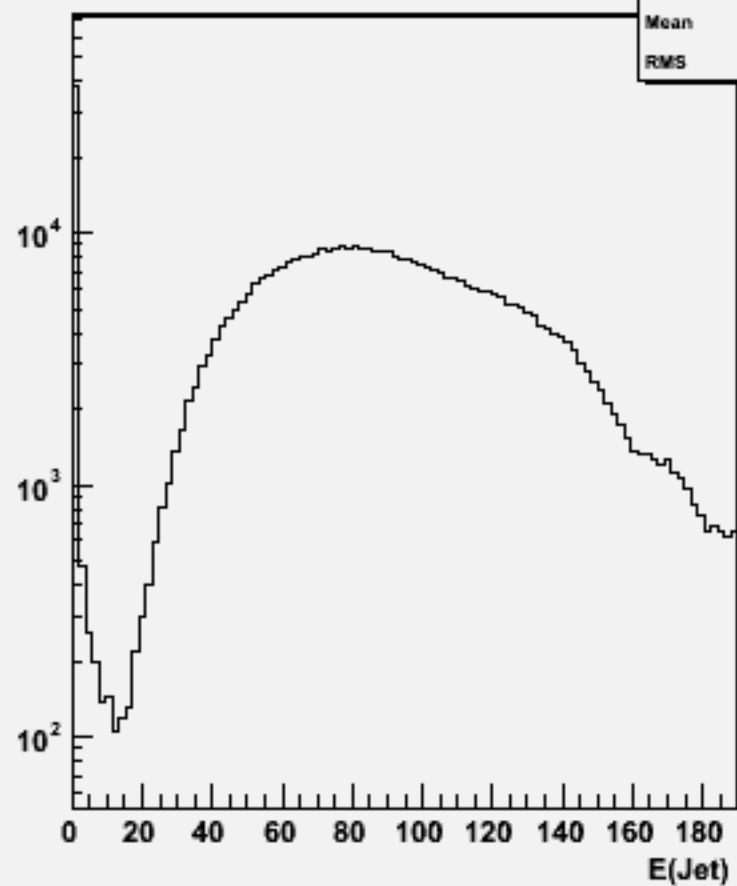
Jet energies(All jets)w100773 e1e1udsc_o
