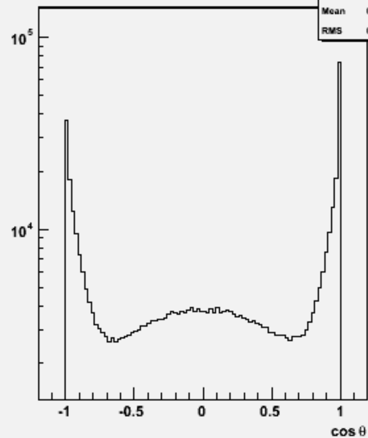
Jet cos \theta (All jets)w100773 e1e1udsc_o
