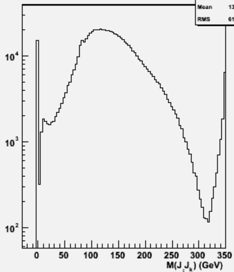
2jets mass(All comb)w100773 e1e1udsc_o
