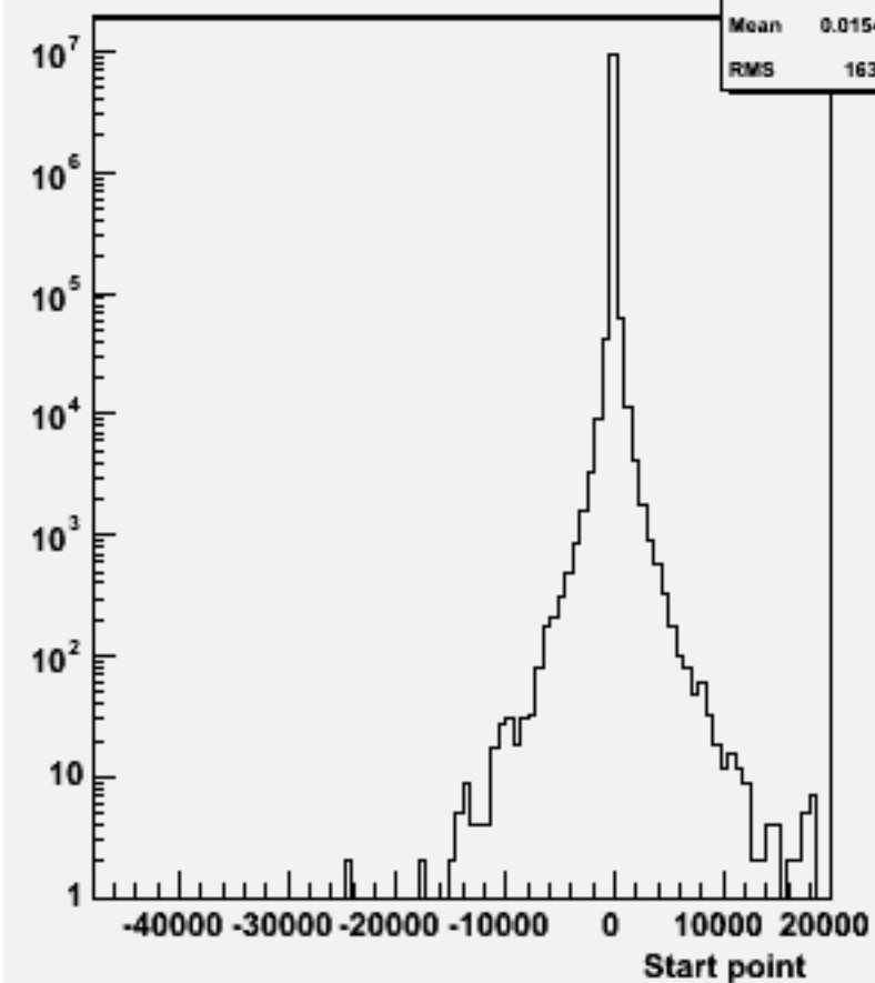
Start point Z : w100773 e1e1udsc_o
