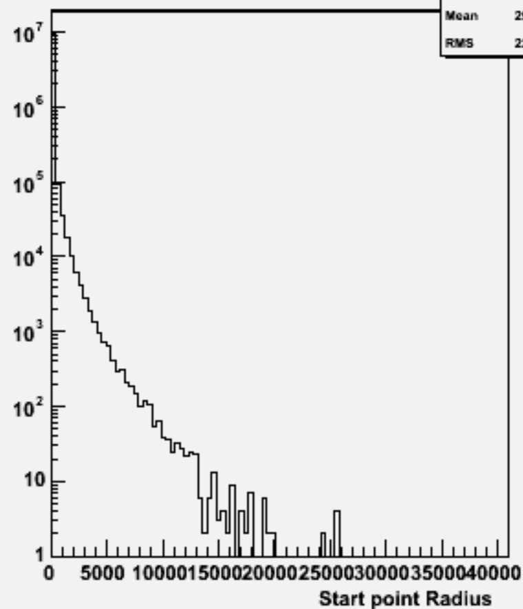
Start point R : w100773 e1e1udsc_o
