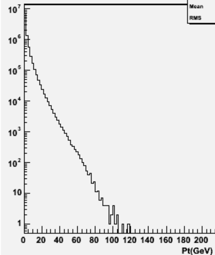
Particle Pt : w100773 e1e1udsc_o
