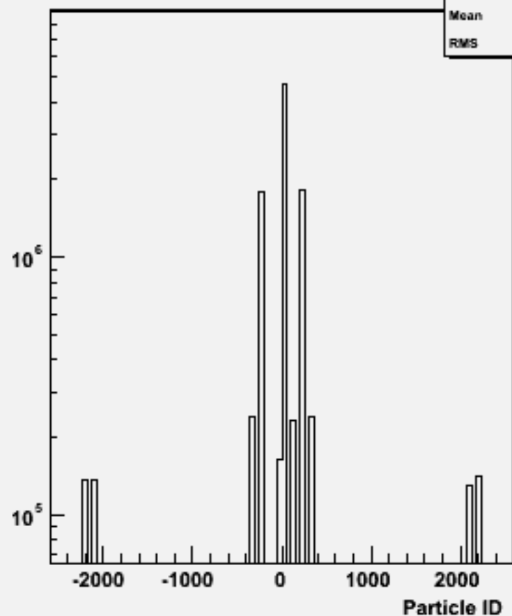
Particle ID : w100773 e1e1udsc_o
