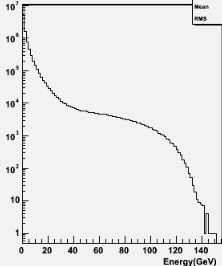
Particle Energy : w100773 e1e1udsc_o
