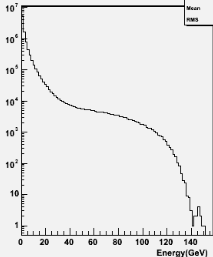
Particle Energy : w100772 e1e1udsc_o
