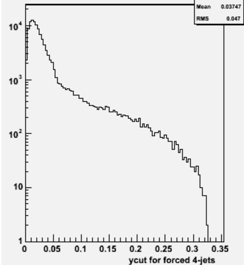
Ycut for 4-jets :w100772 e1e1udsc_o
