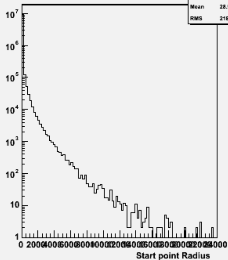
Start point R : w100772 e1e1udsc_o
