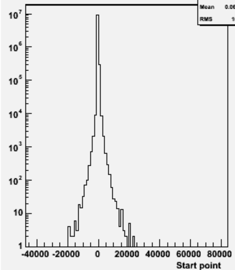
Start point Z : w100772 e1e1udsc_o
