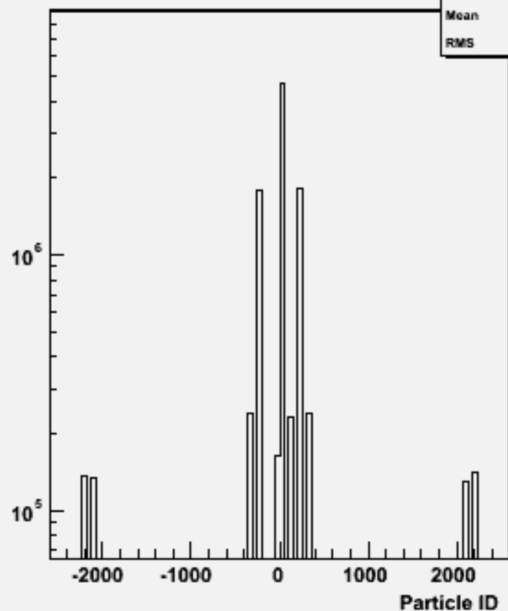
Particle ID : w100772 e1e1udsc_o
