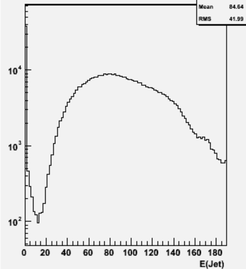
Jet energies(All jets)w100772 e1e1udsc_o
