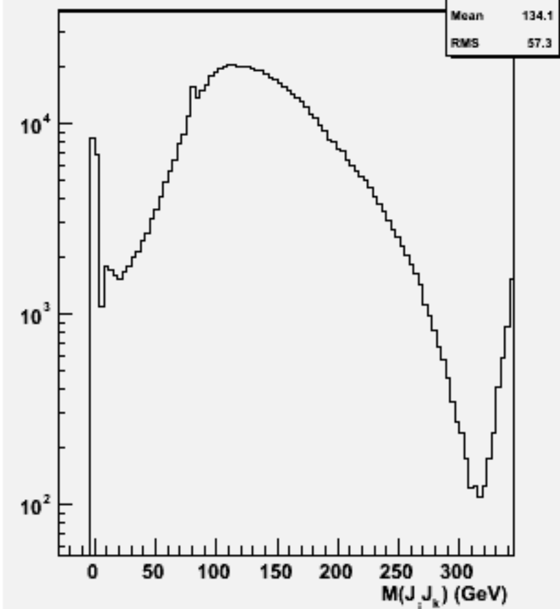
2jets mass(All comb)w100772 e1e1udsc_o
