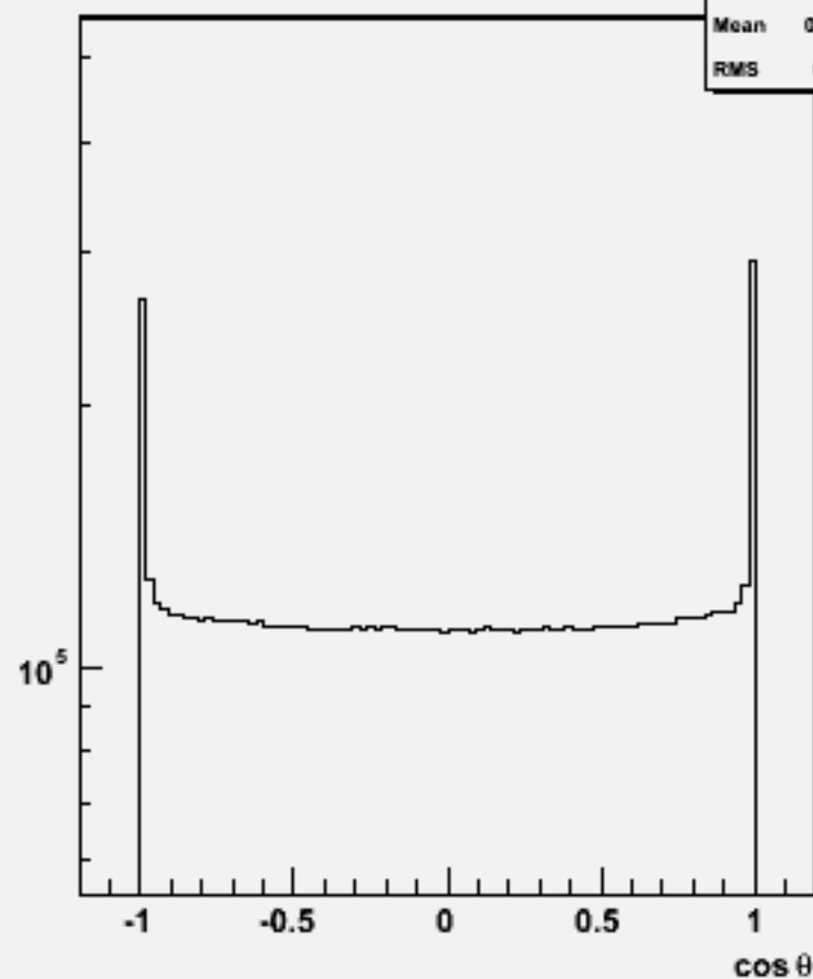
Particle cos \theta : w100772 e1e1udsc_o
