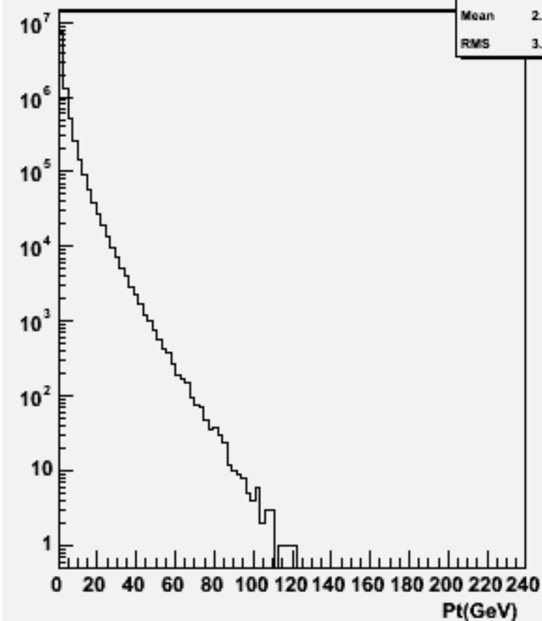
Particle Pt : w100772 e1e1udsc_o
