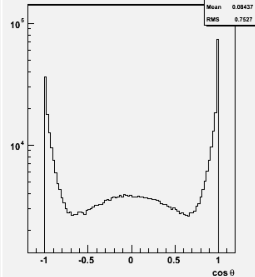
Jet cosθ (All jets)w100772 e1e1udsc_o
