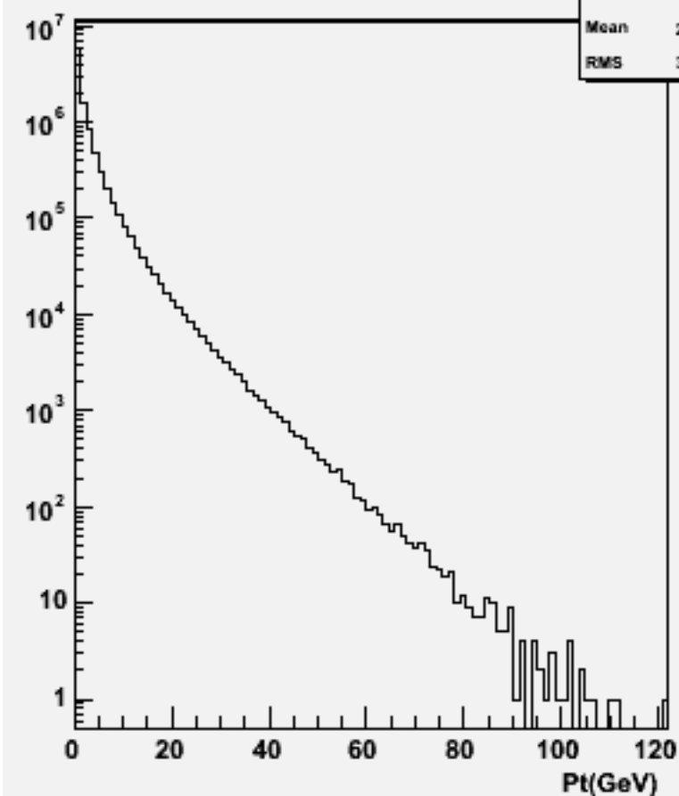
Particle Pt : w100771 e1e1udsc_o
