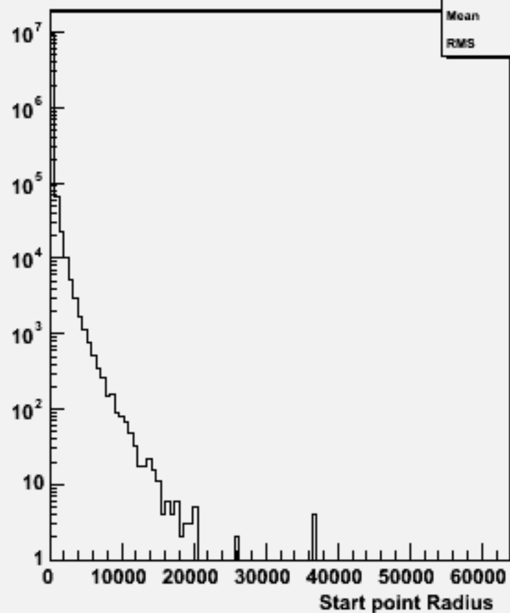
Start point R : w100771 e1e1udsc_o
