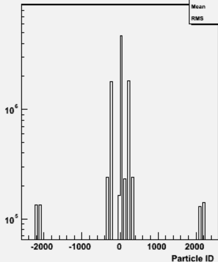
Particle ID : w100771 e1e1udsc_o
