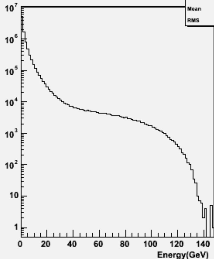
Particle Energy : w100771 e1e1udsc_o
