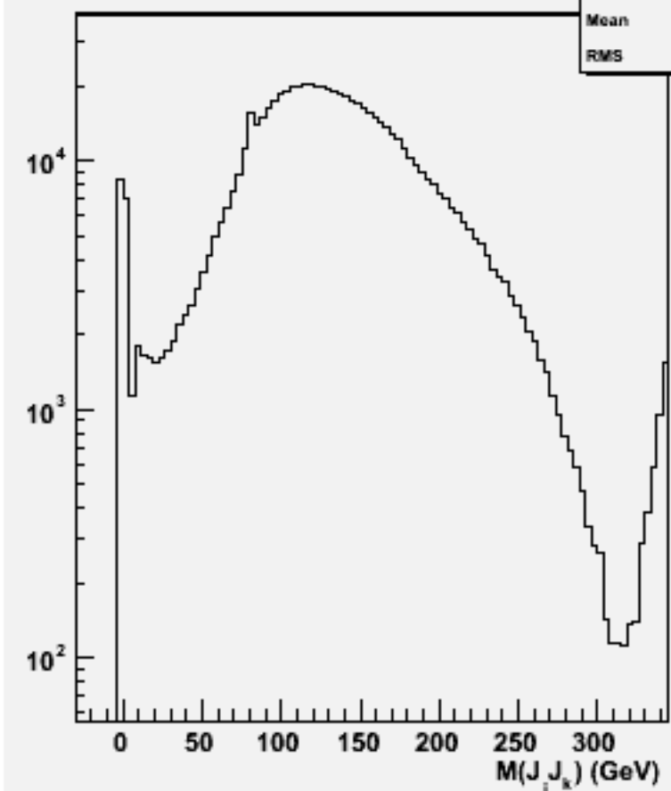
2jets mass(All comb)w100771 e1e1udsc_o
