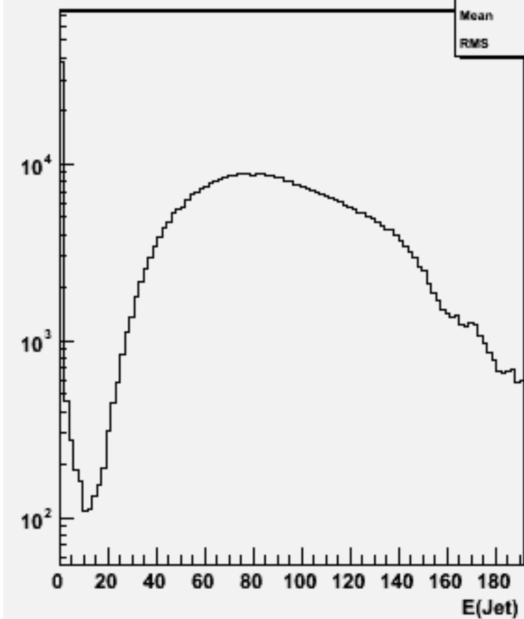
Jet energies(All jets)w100771 e1e1udsc_o
