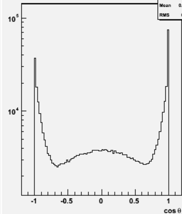
Jet cosθ (All jets)w100771 e1e1udsc_o
