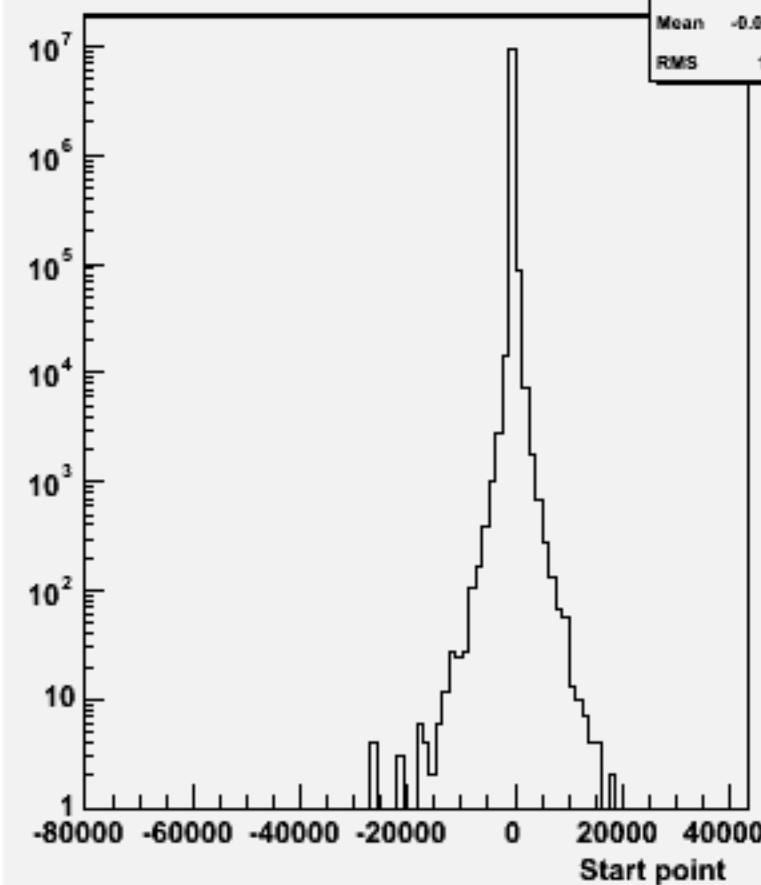
Start point Z : w100771 e1e1udsc_o
