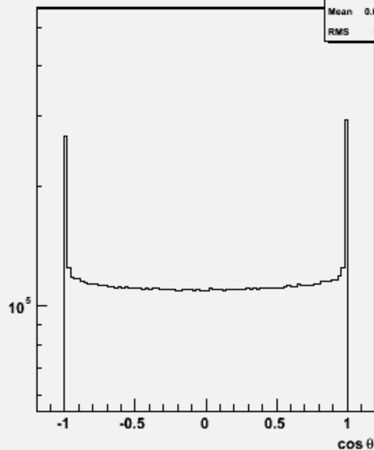
Particle cos \theta : w100771 e1e1udsc_o
