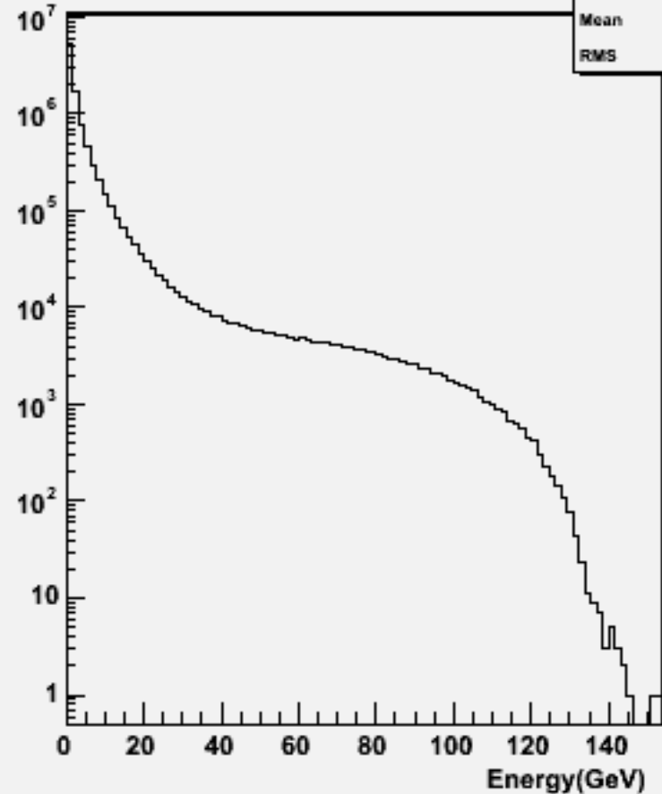
Particle Energy : w100770 e1e1uddu_o
