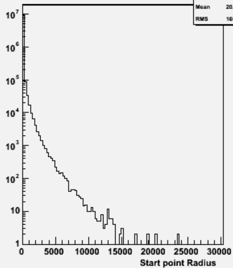
Start point R : w100770 e1e1uddu_o
