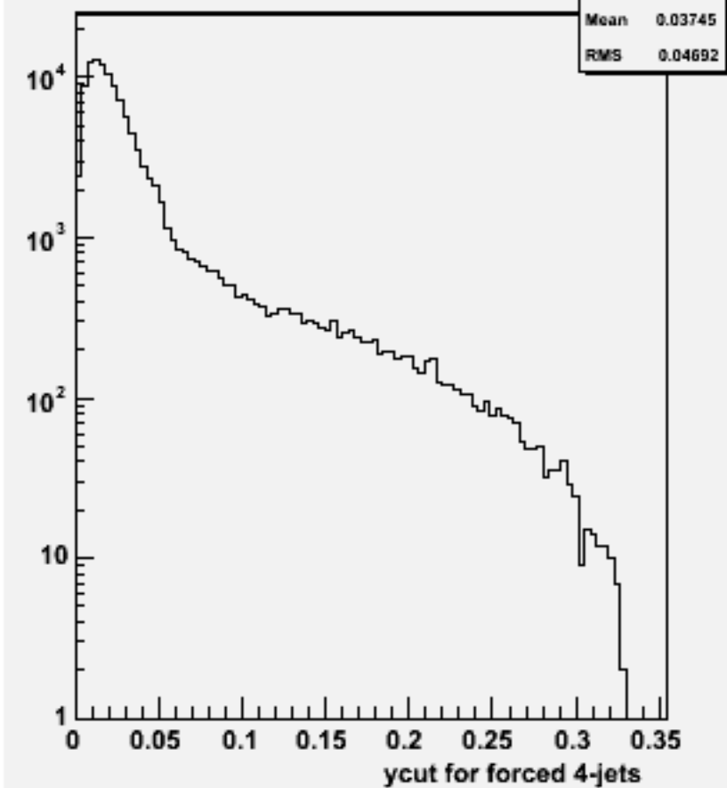
Ycut for 4-jets :w100770 e1e1uddu_o
