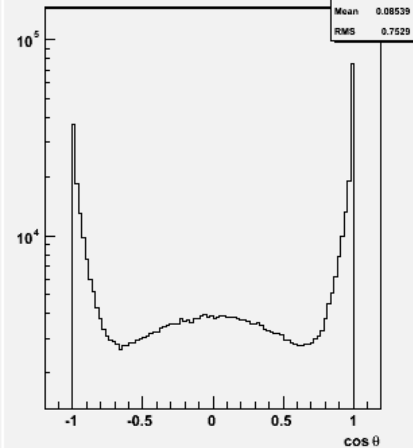
Jet cos \theta (All jets)w100770 e1e1uddu_o
