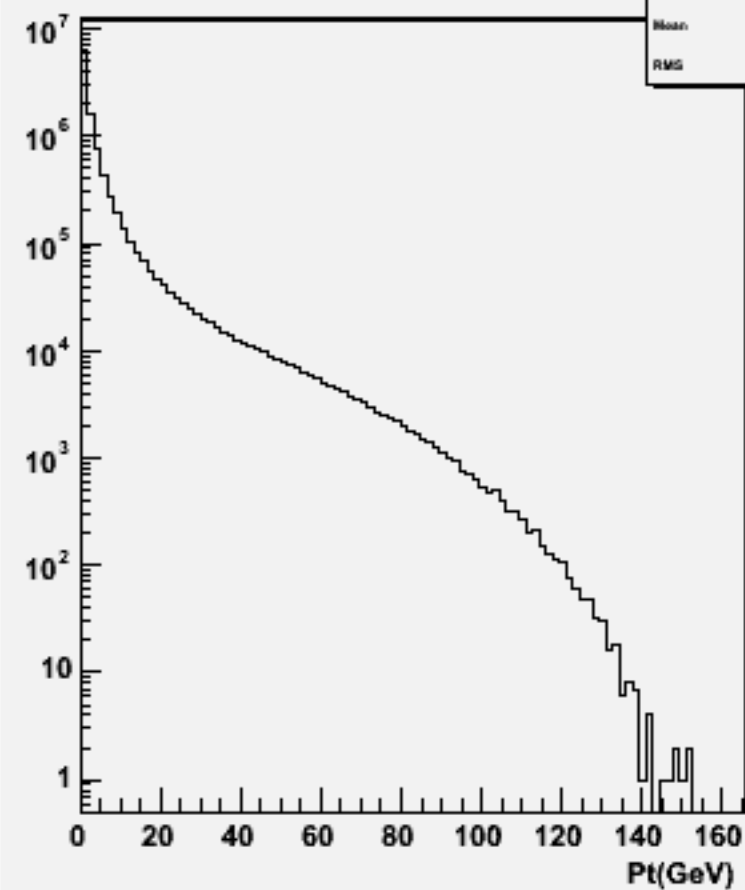
Particle Pt : w100766 e1e1ude3n3_o
