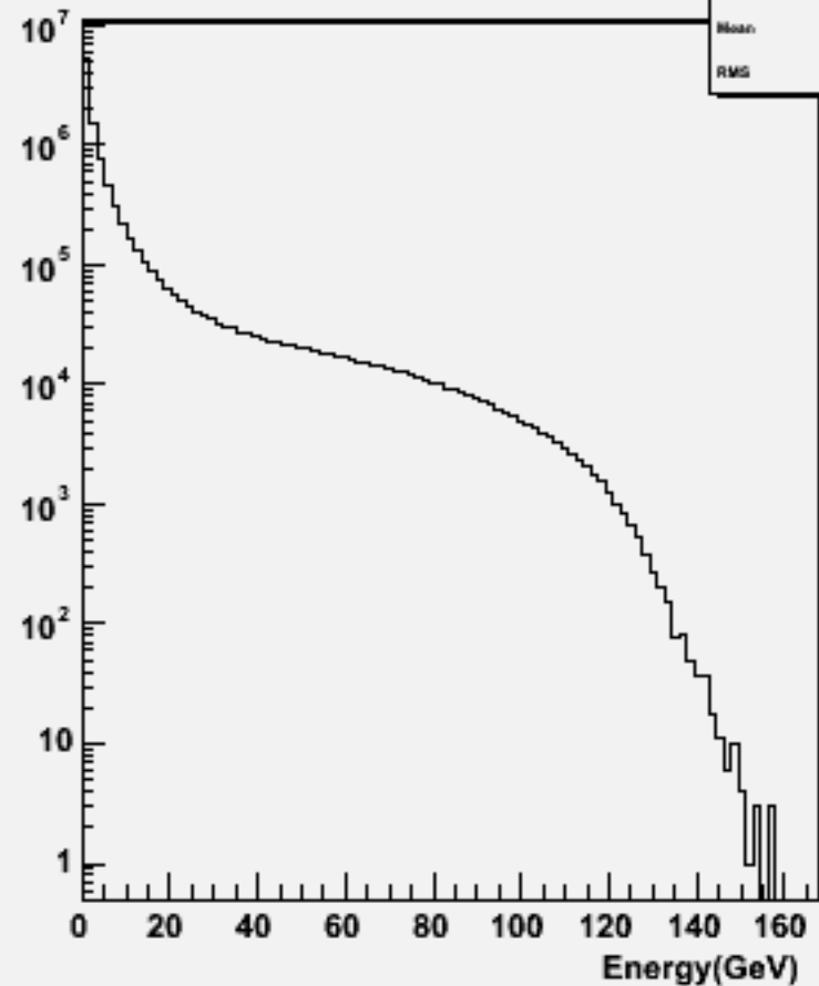
Particle Energy : w100766 e1e1ude3n3_o
