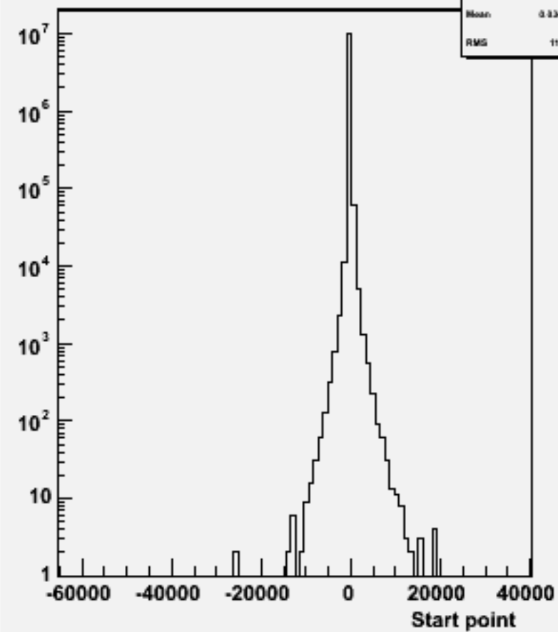
Start point Z : w100766 e1e1ude3n3_o
