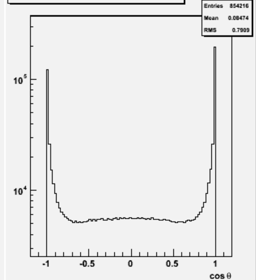
Jet cos \theta (All jets)w100766 e1e1ude3n3_o
