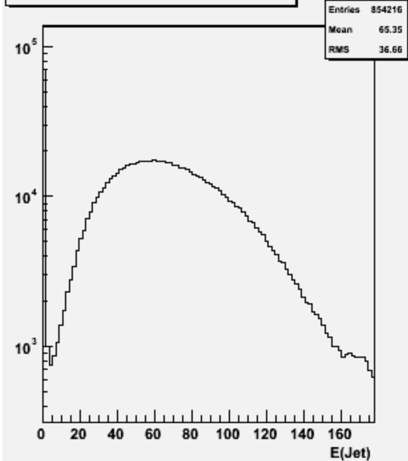
Jet energies(All jets)w100766 e1e1ude3n3_o
