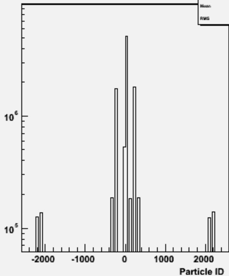
Particle ID : w100766 e1e1ude3n3_o
