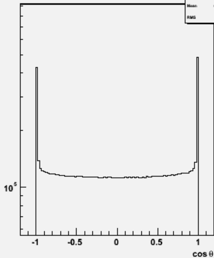
Particle \cos\theta : w100766 e1e1ude3n3_o
