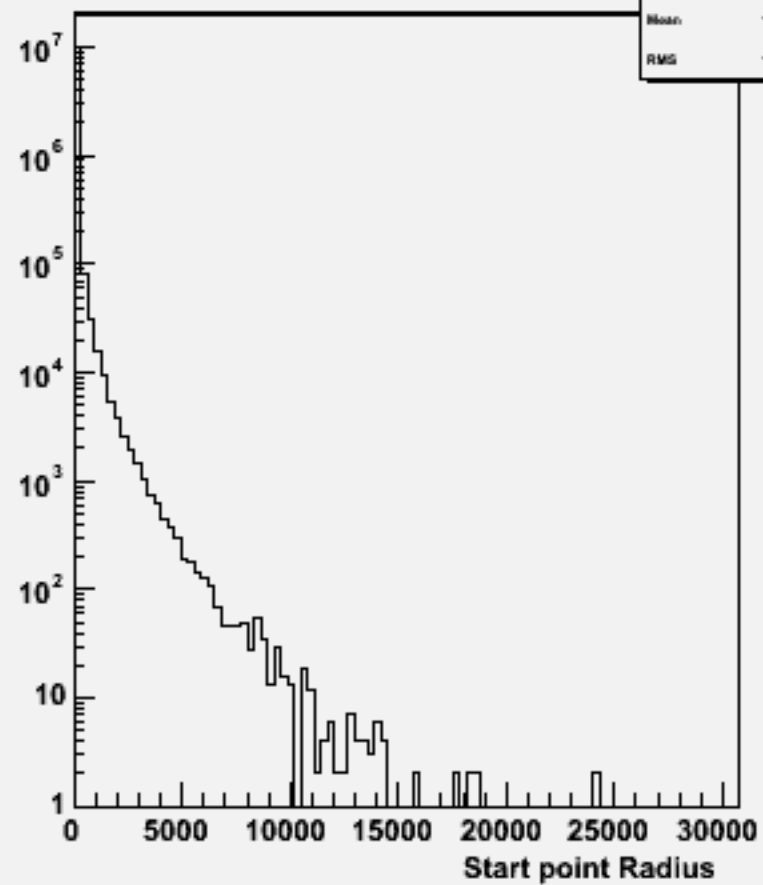
Start point R : w100766 e1e1ude3n3_o
