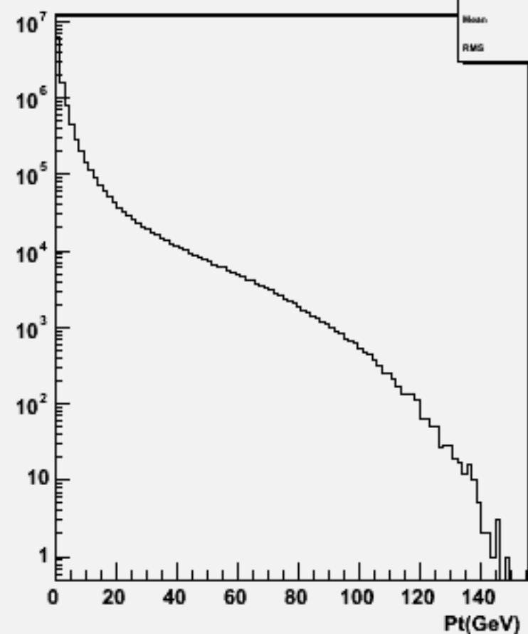
Particle Pt : w100765 e1e1ude3n3_o
