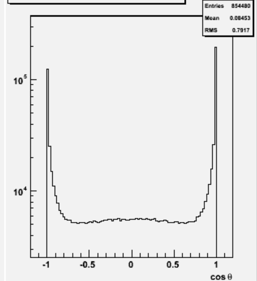
Jet cos \theta (All jets)w100765 e1e1ude3n3_o
