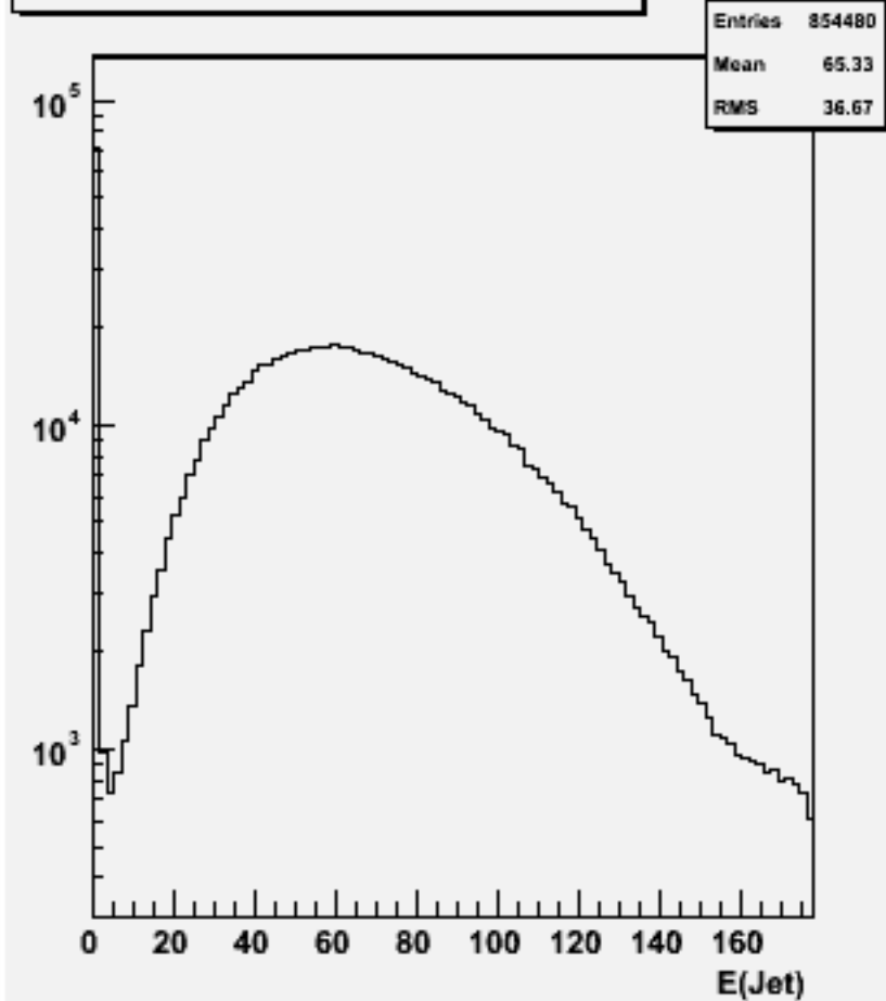
Jet energies(All jets)w100765 e1e1ude3n3_o
