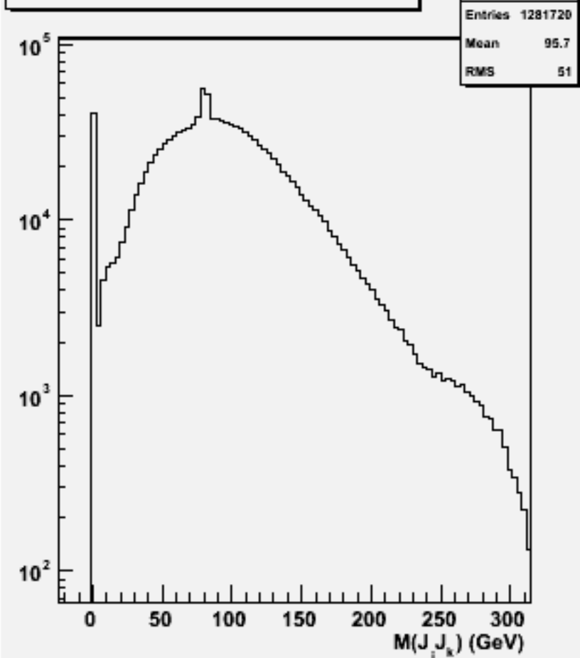
2jets mass(All comb)w100765 e1e1ude3n3_o
