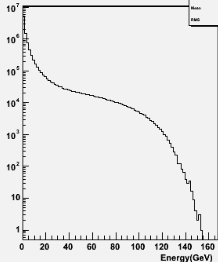
Particle Energy : w100765 e1e1ude3n3_o
