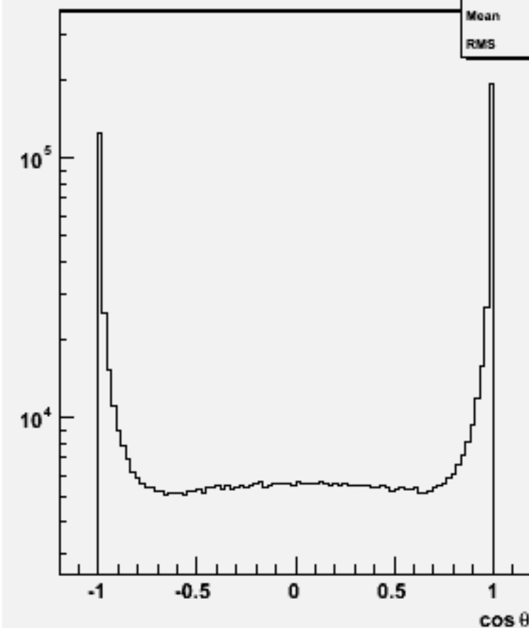
Jet cos \theta (All jets)w100763 e1e1ude3n3_o
