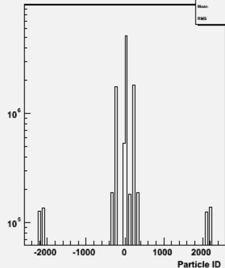
Particle ID : w100763 e1e1ude3n3_o
