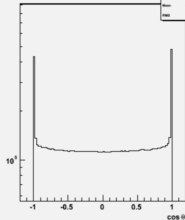
Particle cos \theta : w100763 e1e1ude3n3_o
