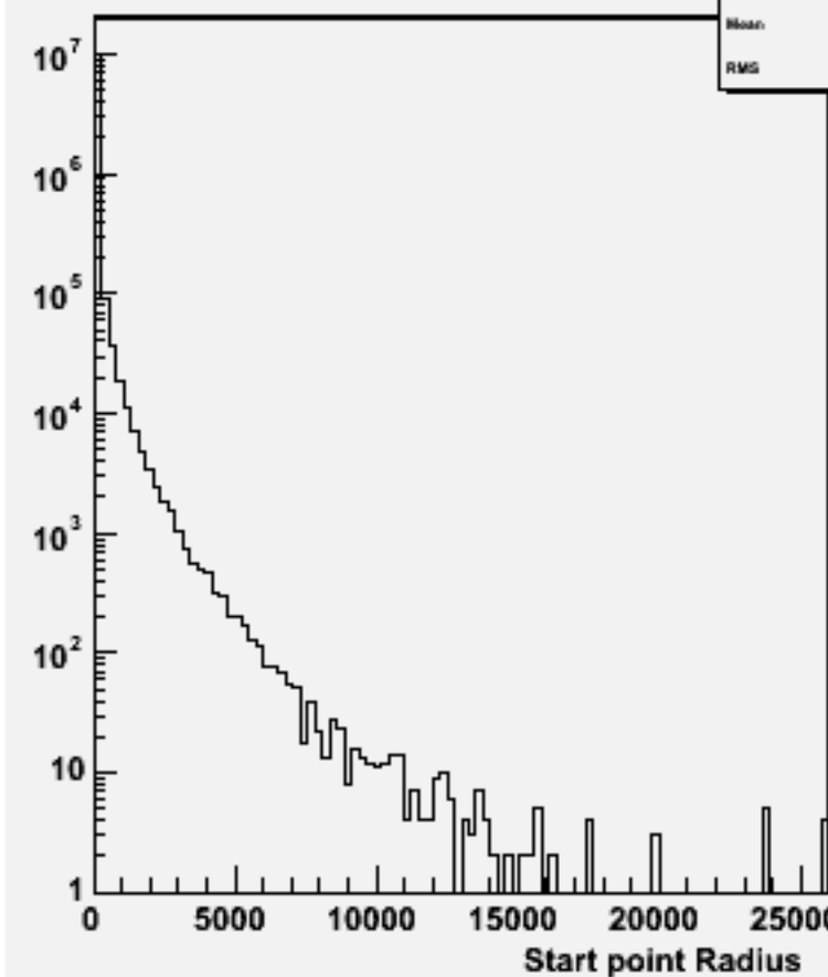
Start point R : w100763 e1e1ude3n3_o
