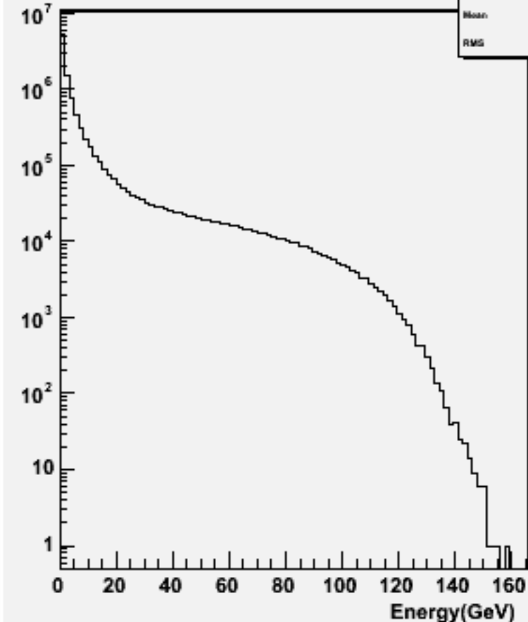
Particle Energy : w100763 e1e1ude3n3_o
