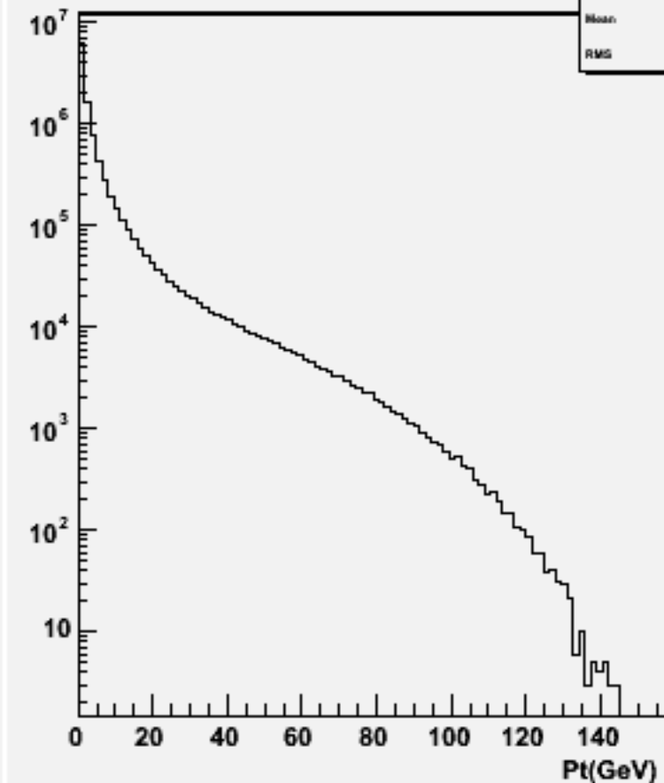
Particle Pt : w100763 e1e1ude3n3_o
