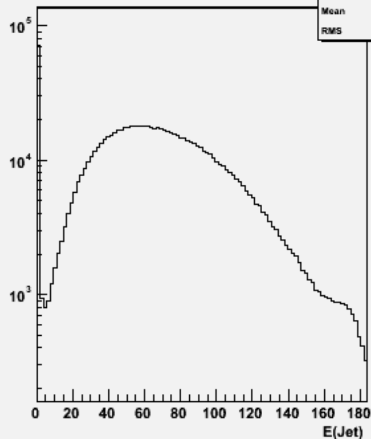
Jet energies(All jets)w100763 e1e1ude3n3_o
