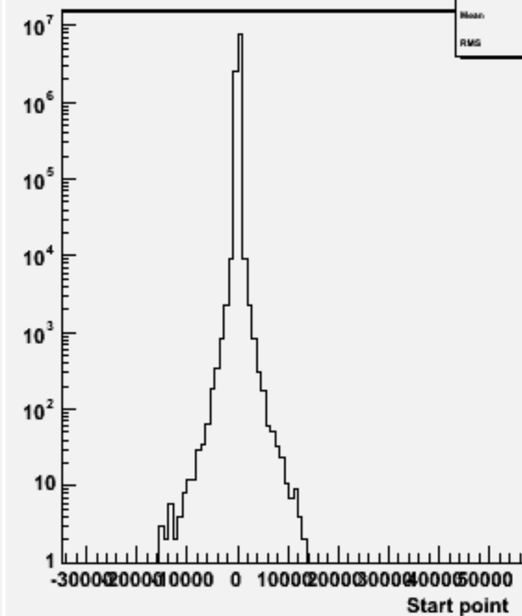
Start point Z : w100763 e1e1ude3n3_o
