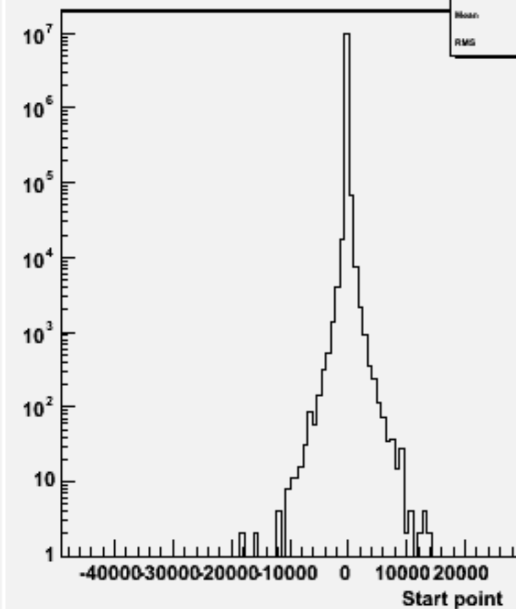
Start point Z : w100762 e1e1ude2n2_o
