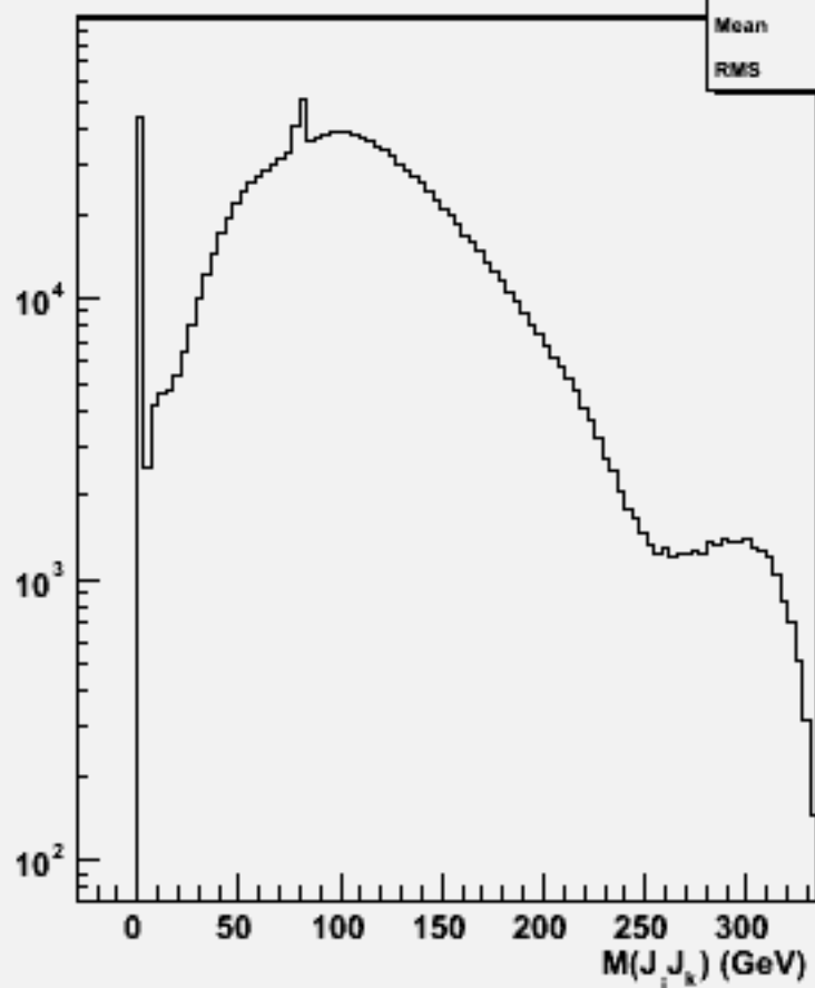
2jets mass(All comb)w100762 e1e1ude2n2_o
