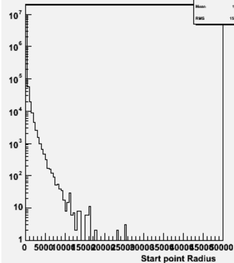
Start point R : w100762 e1e1ude2n2_o
