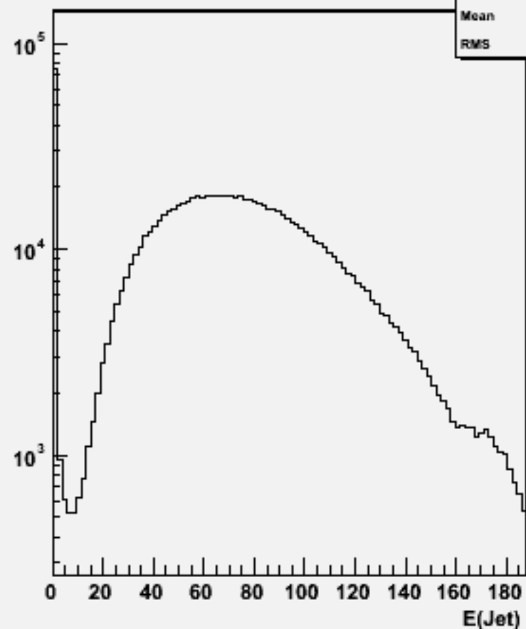
Jet energies(All jets)w100762 e1e1ude2n2_o
