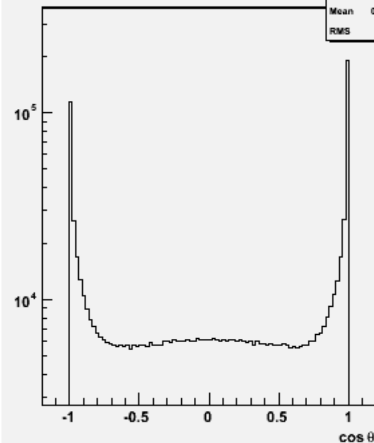
Jet cos \theta (All jets)w100762 e1e1ude2n2_o
