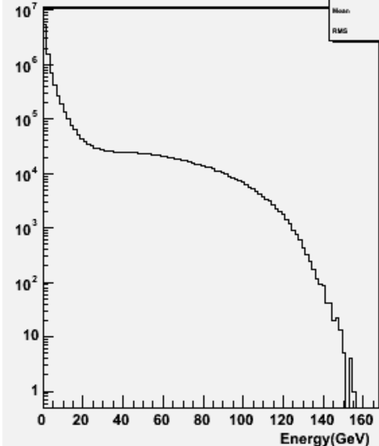
Particle Energy : w100762 e1e1ude2n2_o
