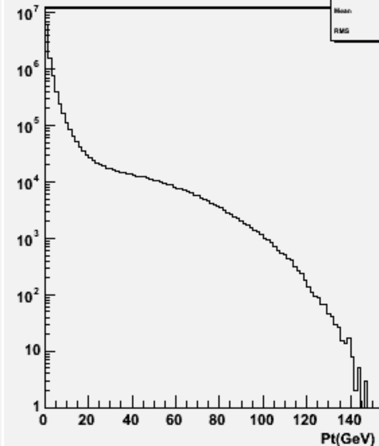
Particle Pt : w100762 e1e1ude2n2_o
