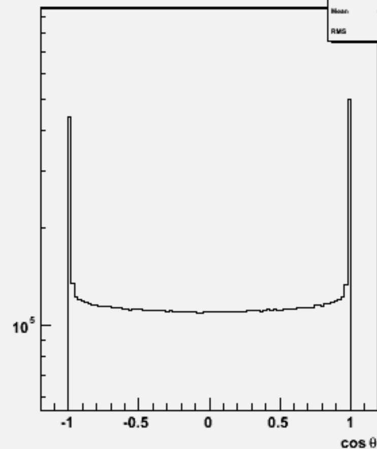
Particle \cos\theta : w100762 e1e1ude2n2_o
