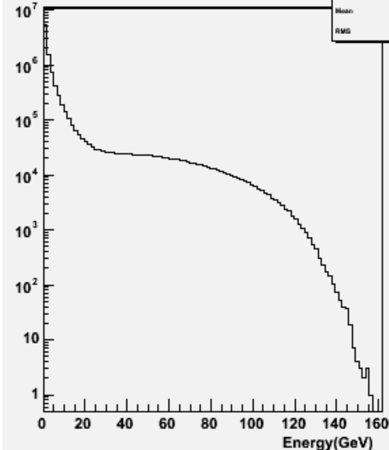
Particle Energy : w100761 e1e1ude2n2_o
