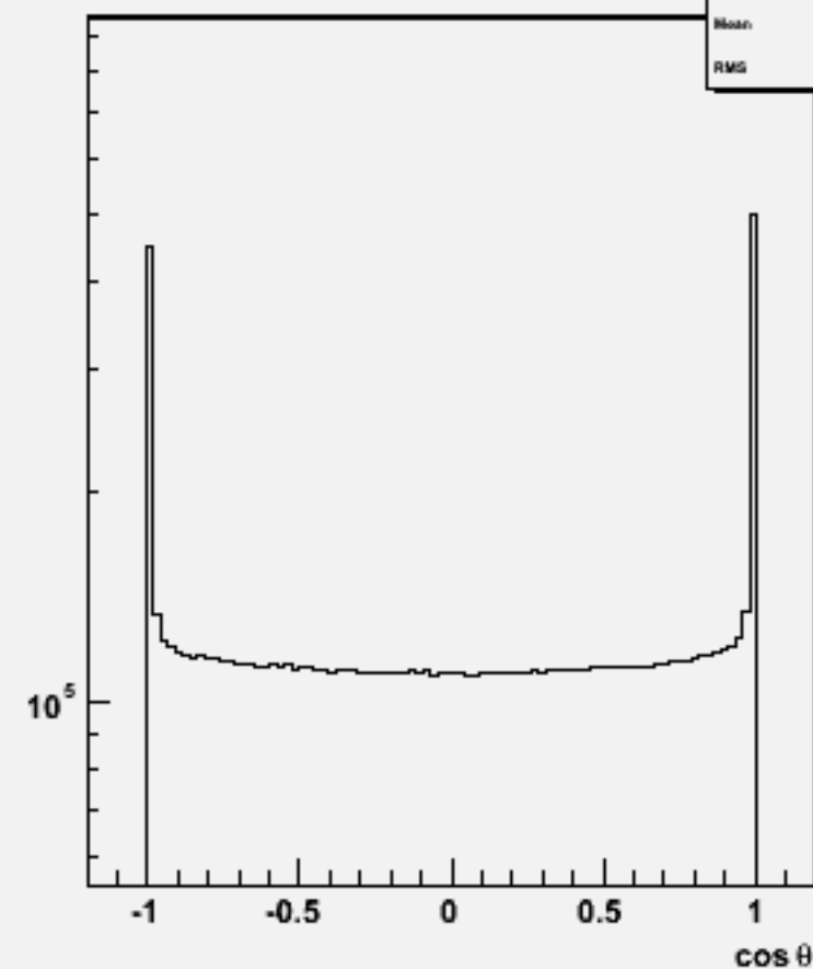
Particle \cos\theta : w100761 e1e1ude2n2_o
