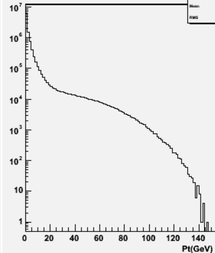
Particle Pt : w100761 e1e1ude2n2_o
