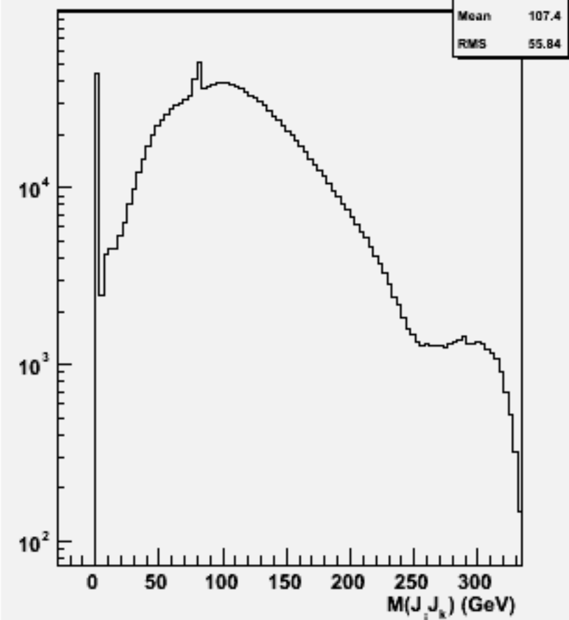
2jets mass(All comb)w100761 e1e1ude2n2_o
