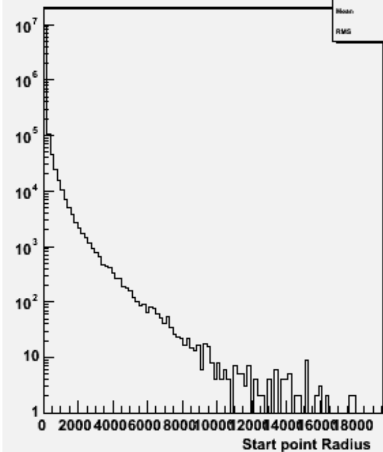
Start point R : w100761 e1e1ude2n2_o
