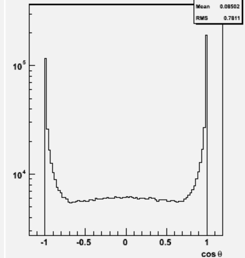
Jet cos \theta (All jets)w100761 e1e1ude2n2_o
