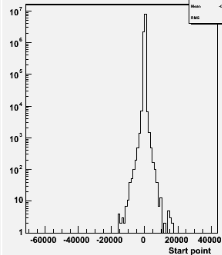
Start point Z : w100761 e1e1ude2n2_o
