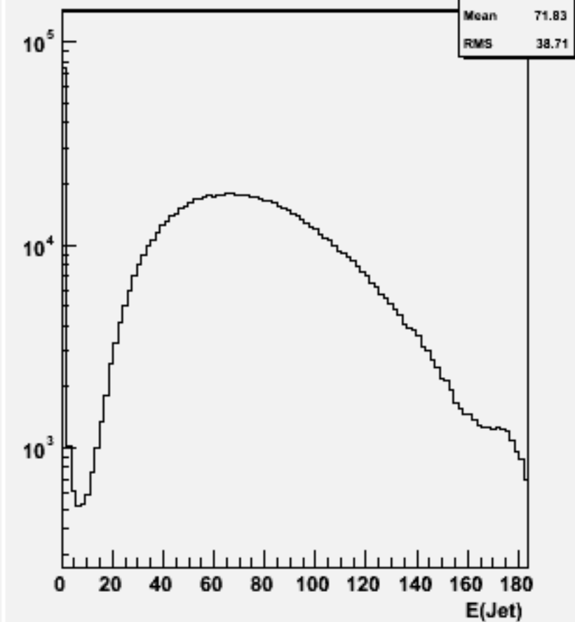
Jet energies(All jets)w100761 e1e1ude2n2_o
