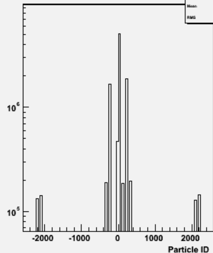
Particle ID : w100761 e1e1ude2n2_o
