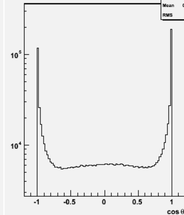
Jet cos \theta (All jets)w100759 e1e1ude2n2_o
