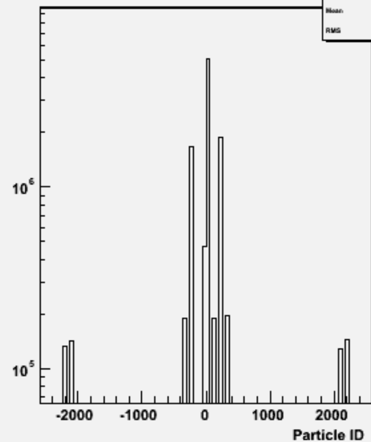
Particle ID : w100759 e1e1ude2n2_o
