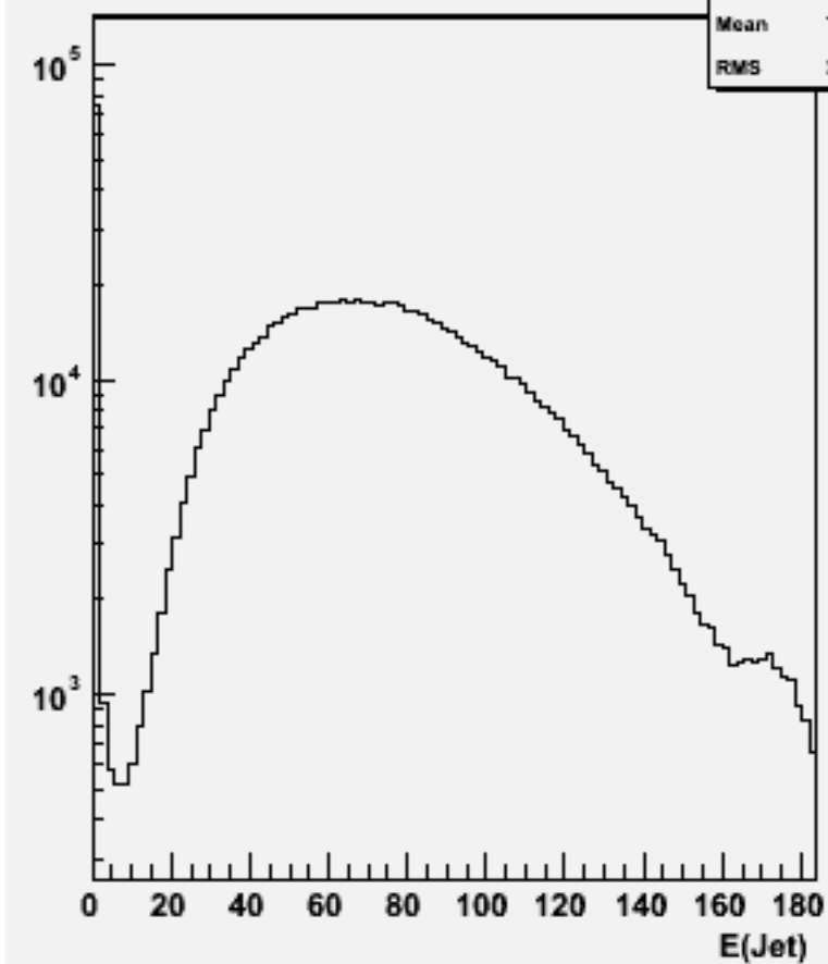
Jet energies(All jets)w100759 e1e1ude2n2_o
