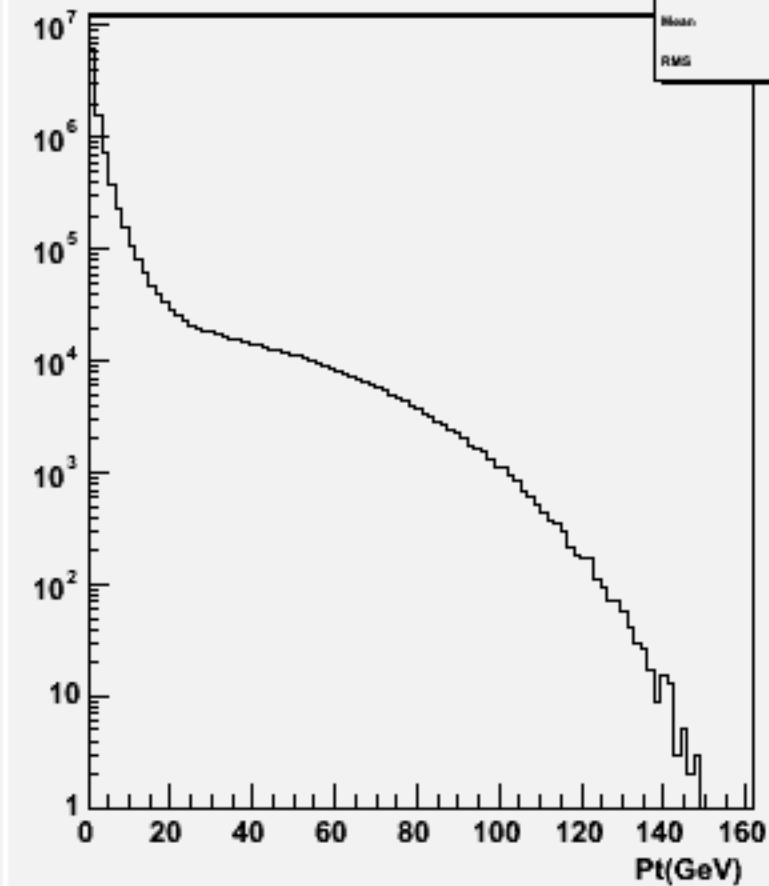
Particle Pt : w100759 e1e1ude2n2_o
