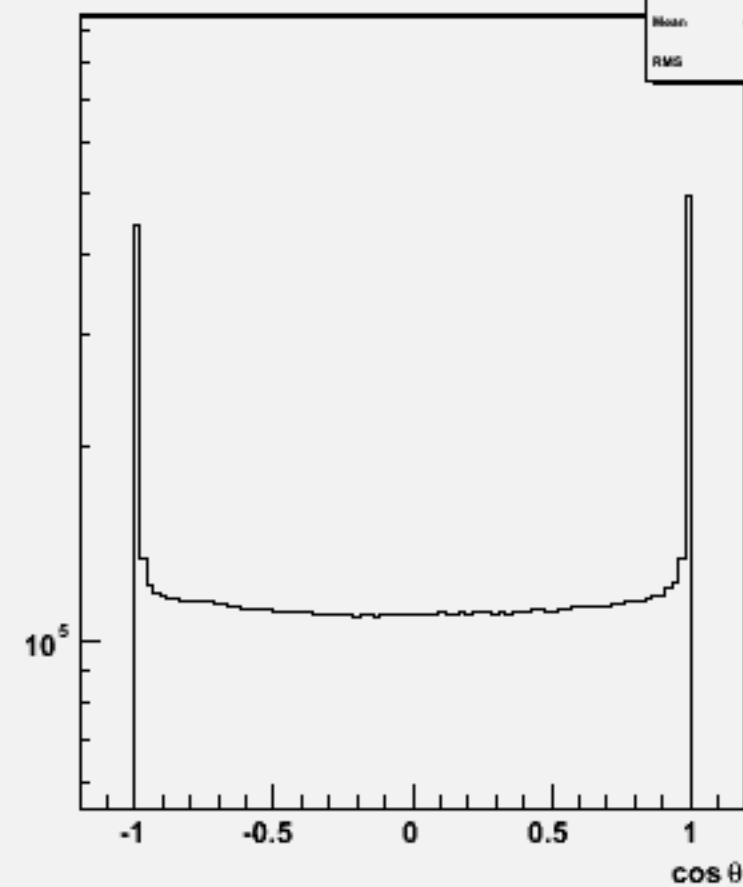
Particle \cos\theta : w100759 e1e1ude2n2_o
