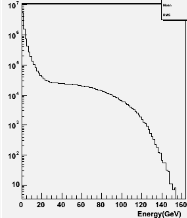
Particle Energy : w100759 e1e1ude2n2_o
