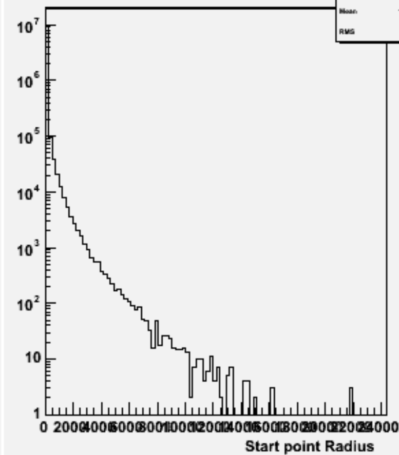
Start point R : w100759 e1e1ude2n2_o
