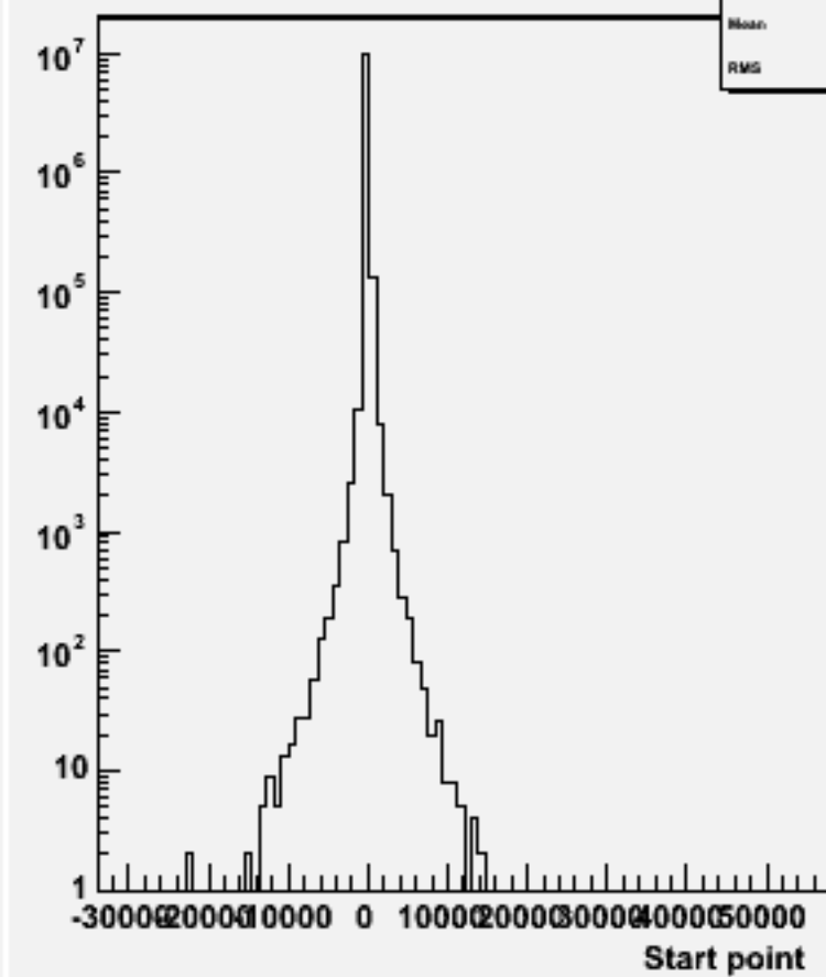
Start point Z : w100759 e1e1ude2n2_o
