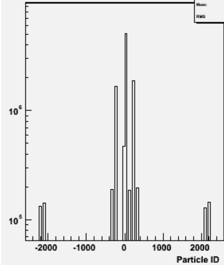
Particle ID : w100758 e1e1ude1n1_o
