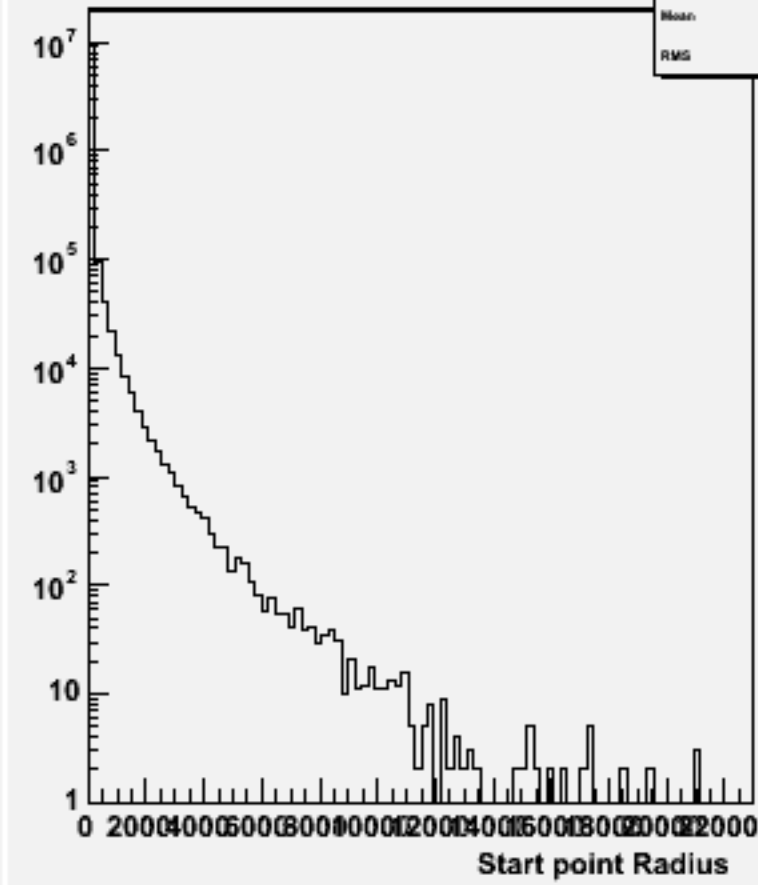
Start point R : w100758 e1e1ude1n1_o
