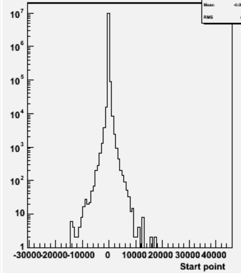
Start point Z : w100758 e1e1ude1n1_o
