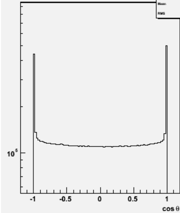
Particle cosθ : w100758 e1e1ude1n1_o
