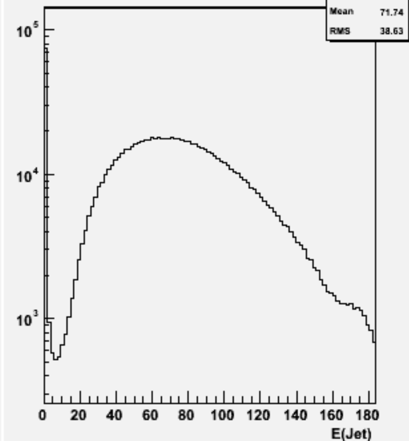
Jet energies(All jets)w100758 e1e1ude1n1_o
