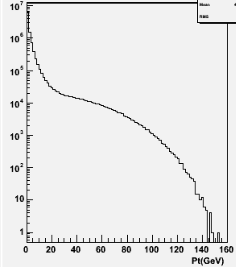
Particle Pt : w100758 e1e1ude1n1_o
