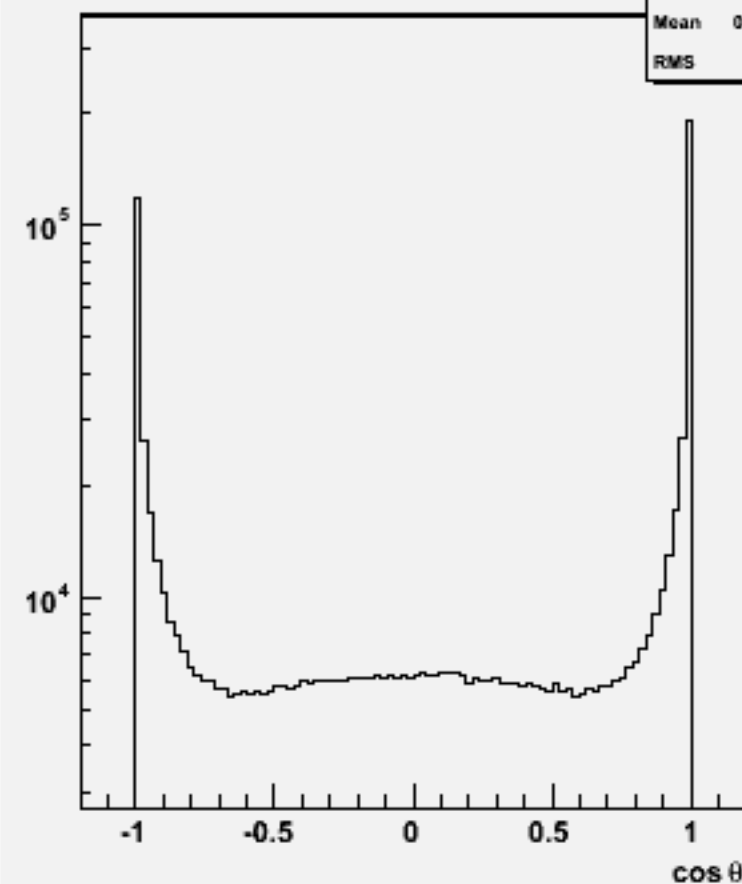
Jet cos \theta (All jets)w100757 e1e1ude1n1_o
