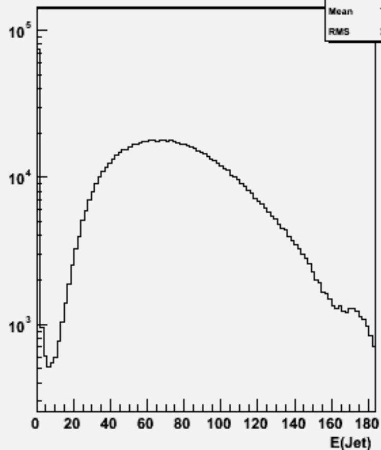
Jet energies(All jets)w100757 e1e1ude1n1_o
