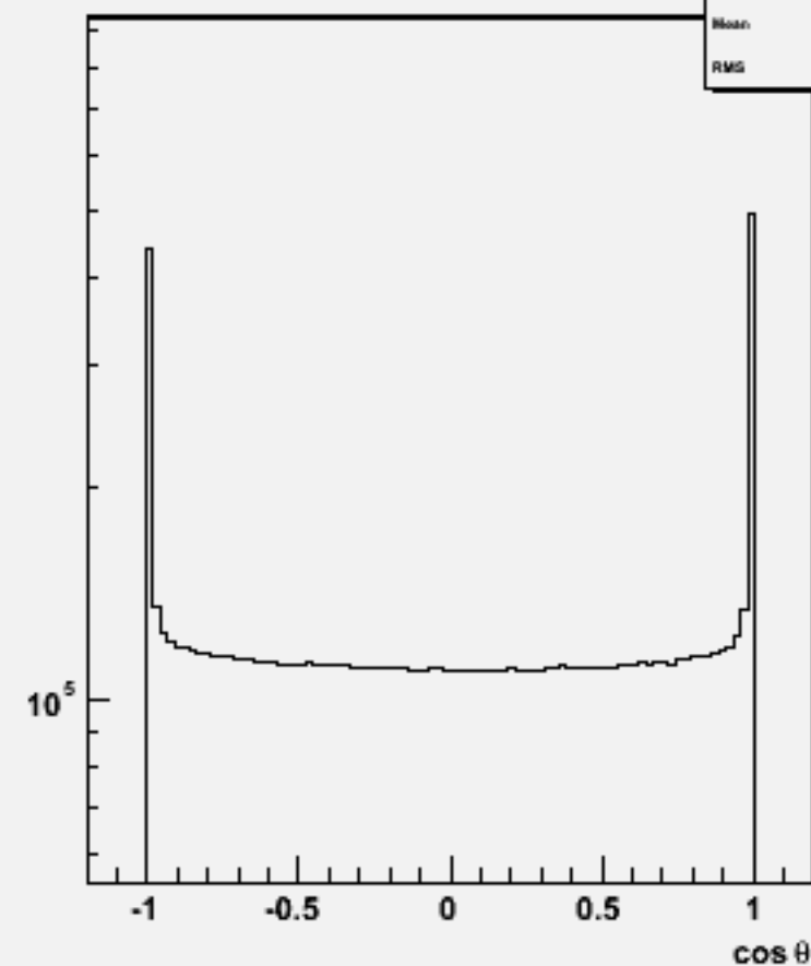
Particle \cos\theta : w100756 e1e1ude1n1_o
