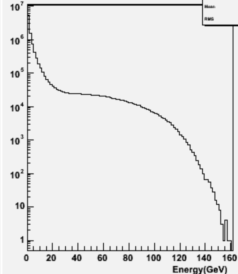
Particle Energy : w100756 e1e1ude1n1_o
