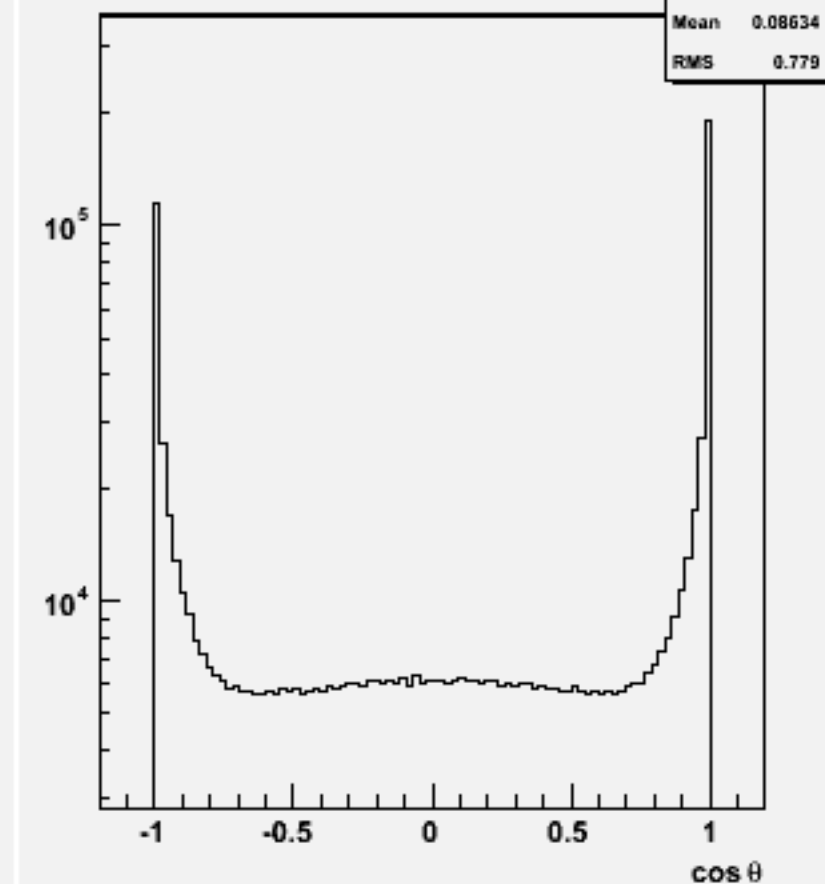
Jet cos \theta (All jets)w100756 e1e1ude1n1_o
