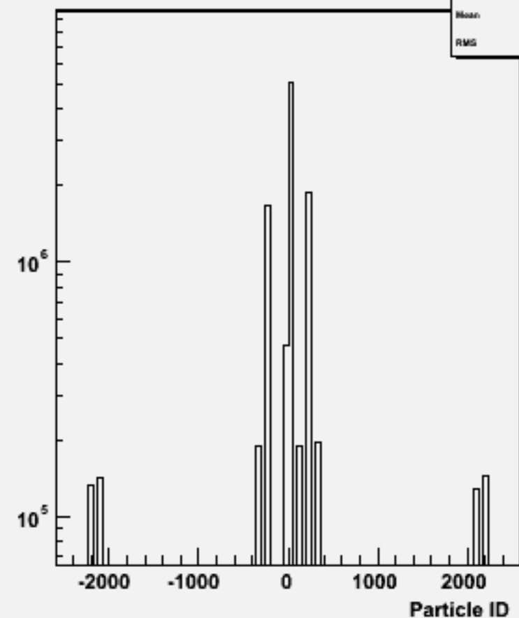
Particle ID : w100756 e1e1ude1n1_o
