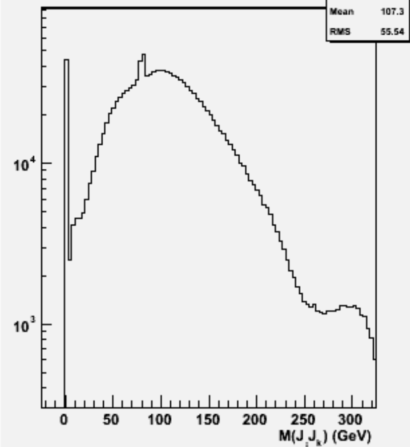
2jets mass(All comb)w100756 e1e1ude1n1_o
