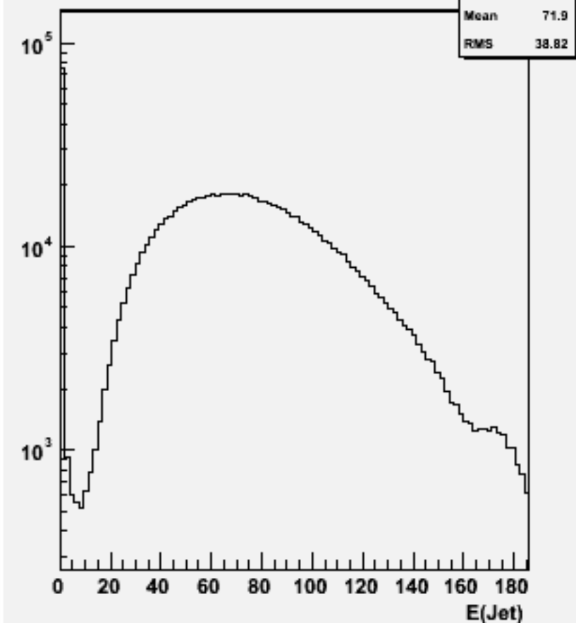
Jet energies(All jets)w100756 e1e1ude1n1_o
