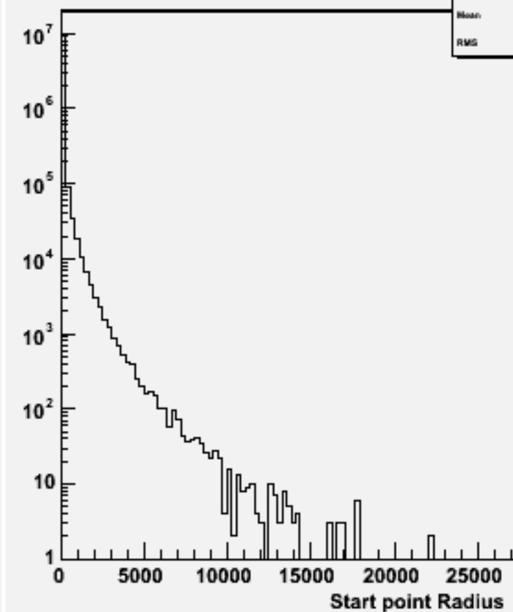
Start point R : w100756 e1e1ude1n1_o
