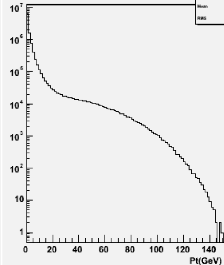
Particle Pt : w100756 e1e1ude1n1_o
