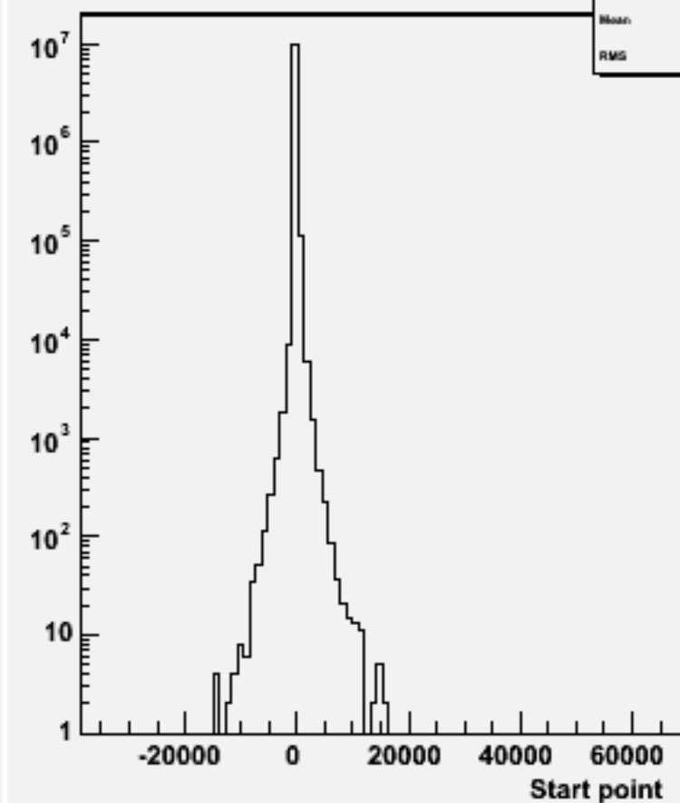
Start point Z : w100756 e1e1ude1n1_o
