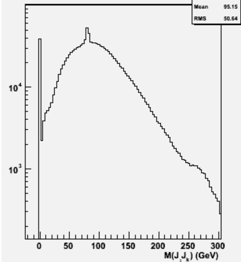
2jets mass(All comb)w100754 e1e1n3e3sc_o
