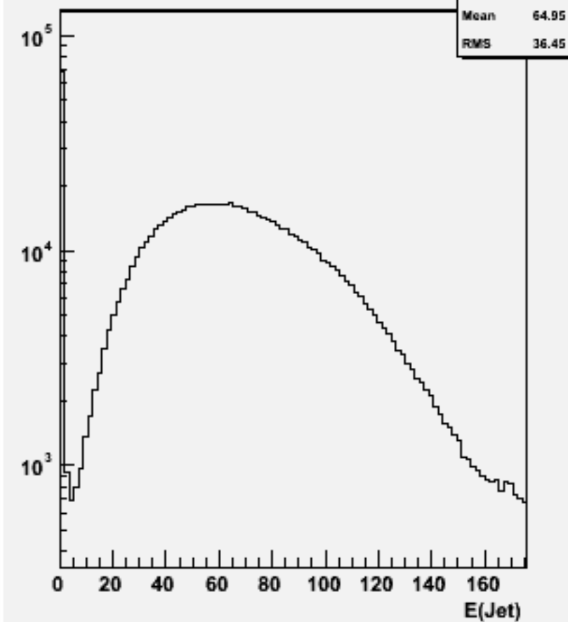
Jet energies(All jets)w100754 e1e1n3e3sc_o
