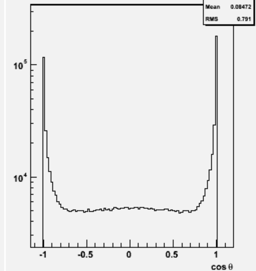
Jet cos \theta (All jets)w100754 e1e1n3e3sc_o
