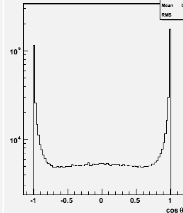
Jet cos \theta (All jets)w100752 e1e1n3e3sc_o
