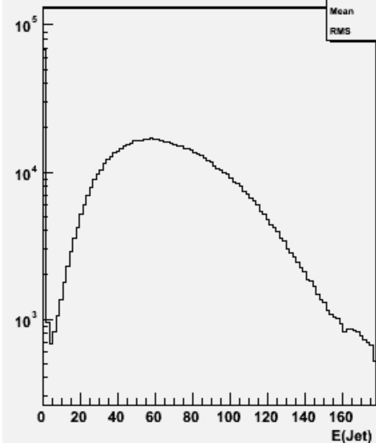
Jet energies(All jets)w100752 e1e1n3e3sc_o
