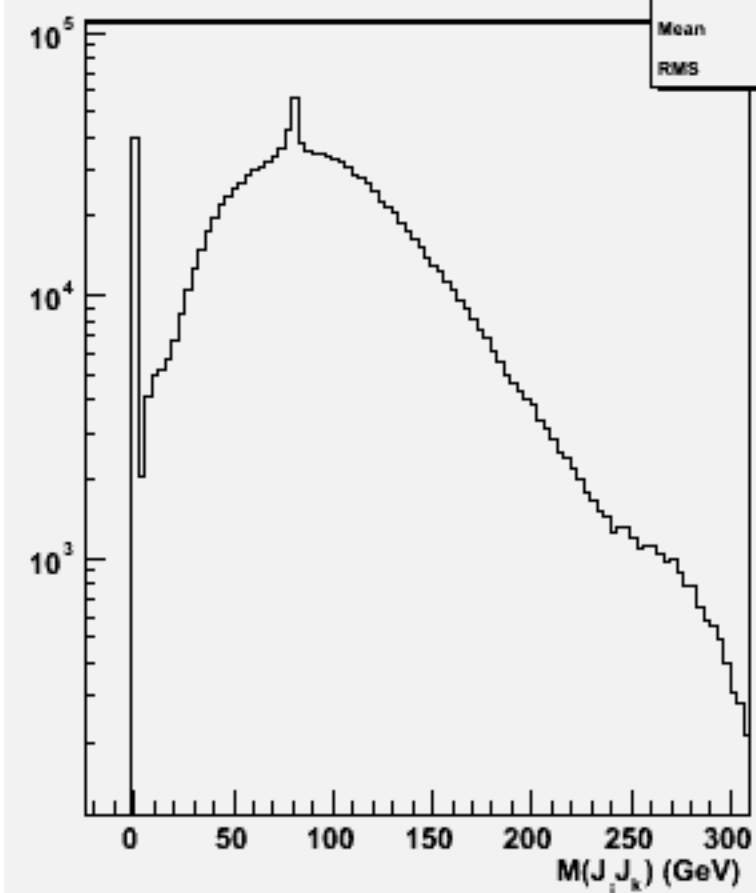
2jets mass(All comb)w100752 e1e1n3e3sc_o
