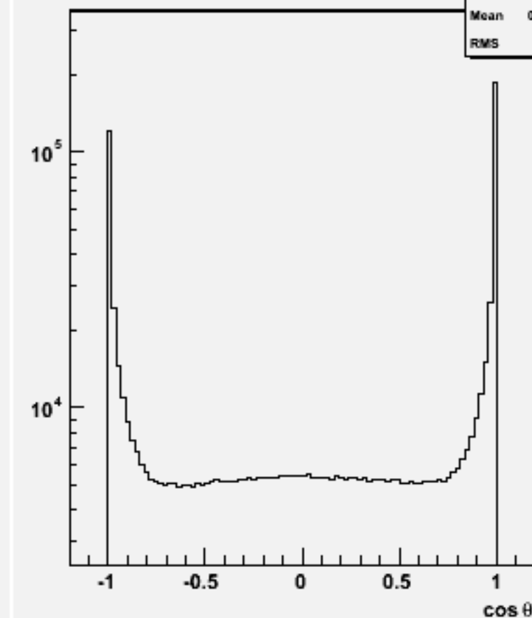
Jet cos \theta (All jets)w100751 e1e1n3e3sc_o
