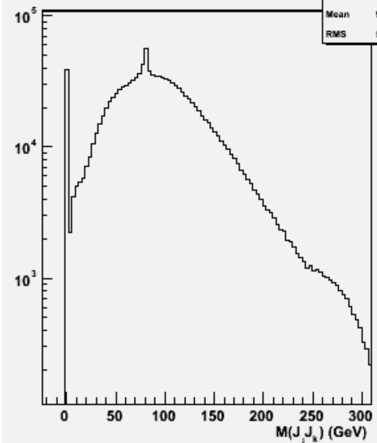
2jets mass(All comb)w100751 e1e1n3e3sc_o
