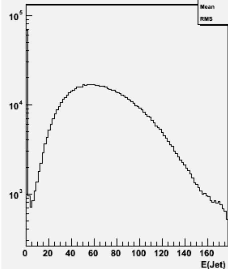
Jet energies(All jets)w100751 e1e1n3e3sc_o
