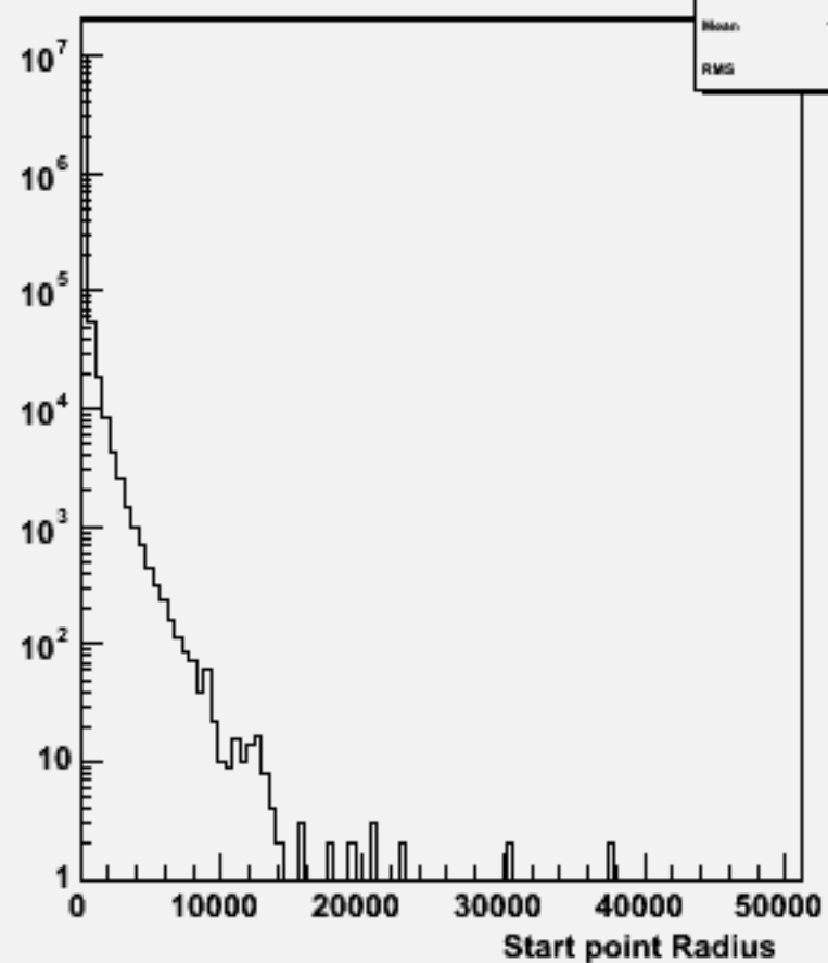
Start point R : w100750 e1e1n3e3du_o
