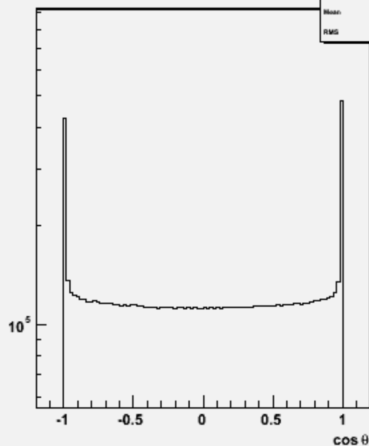
Particle cosθ : w100750 e1e1n3e3du_o
