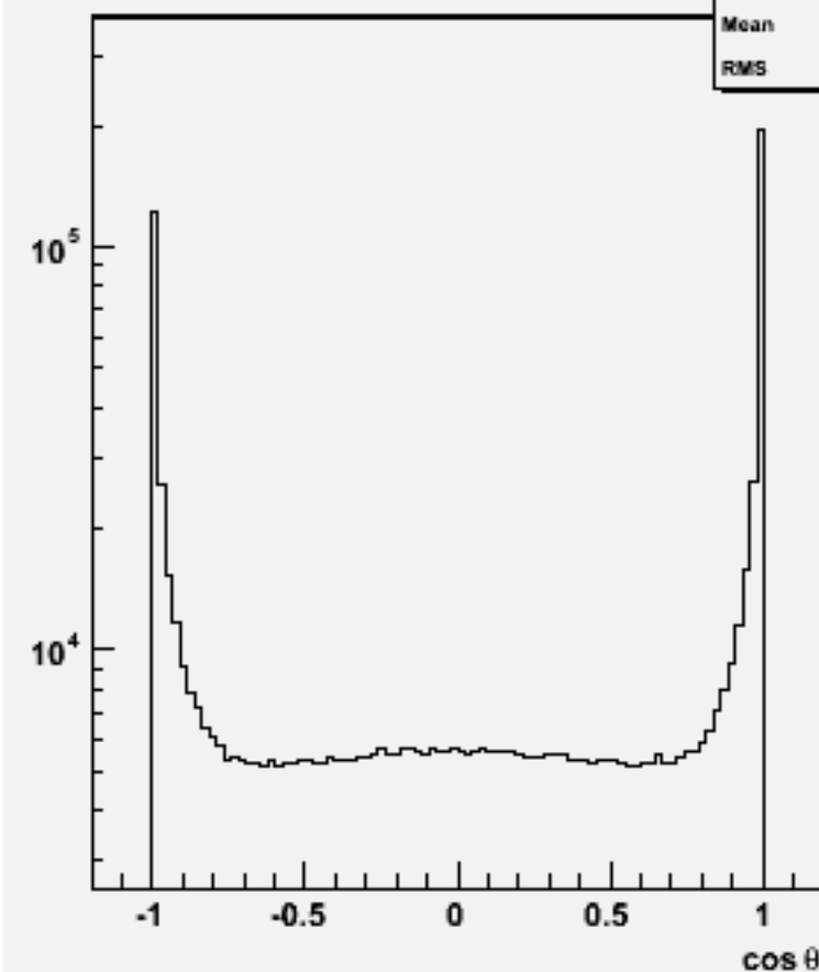
Jet cos \theta (All jets)w100750 e1e1n3e3du_o
