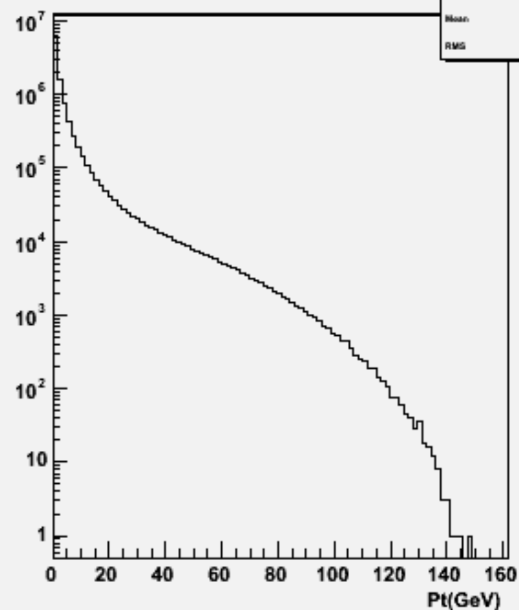
Particle Pt : w100750 e1e1n3e3du_o
