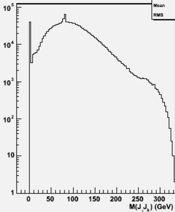
2jets mass(All comb)w100750 e1e1n3e3du_o
