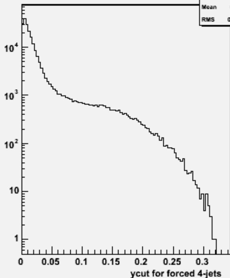
Ycut for 4-jets :w100750 e1e1n3e3du_o
