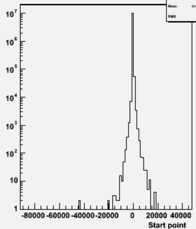
Start point Z : w100750 e1e1n3e3du_o
