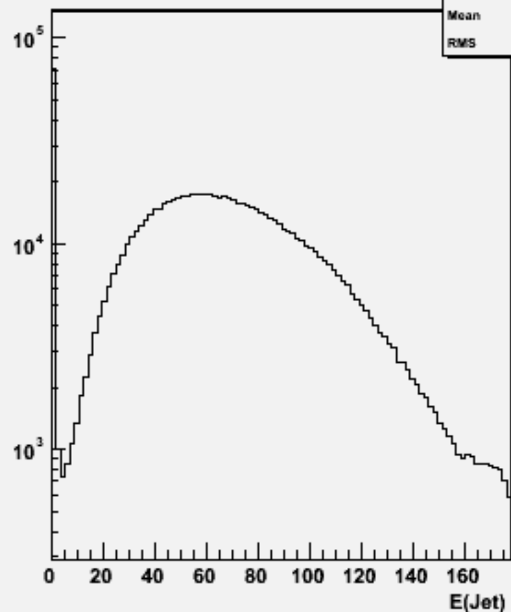
Jet energies(All jets)w100750 e1e1n3e3du_o
