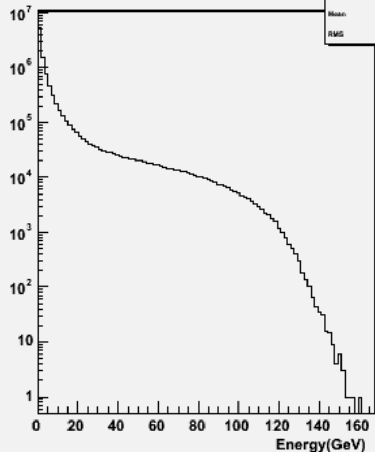
Particle Energy : w100750 e1e1n3e3du_o
