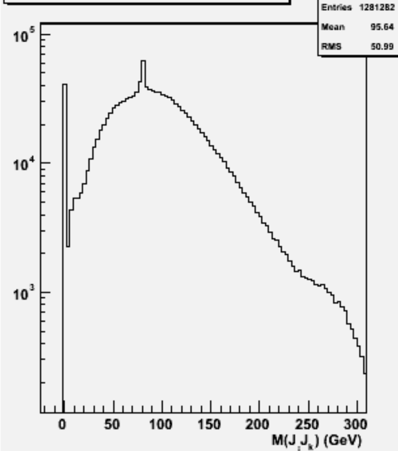
2jets mass(All comb)w100748 e1e1n3e3du_o
