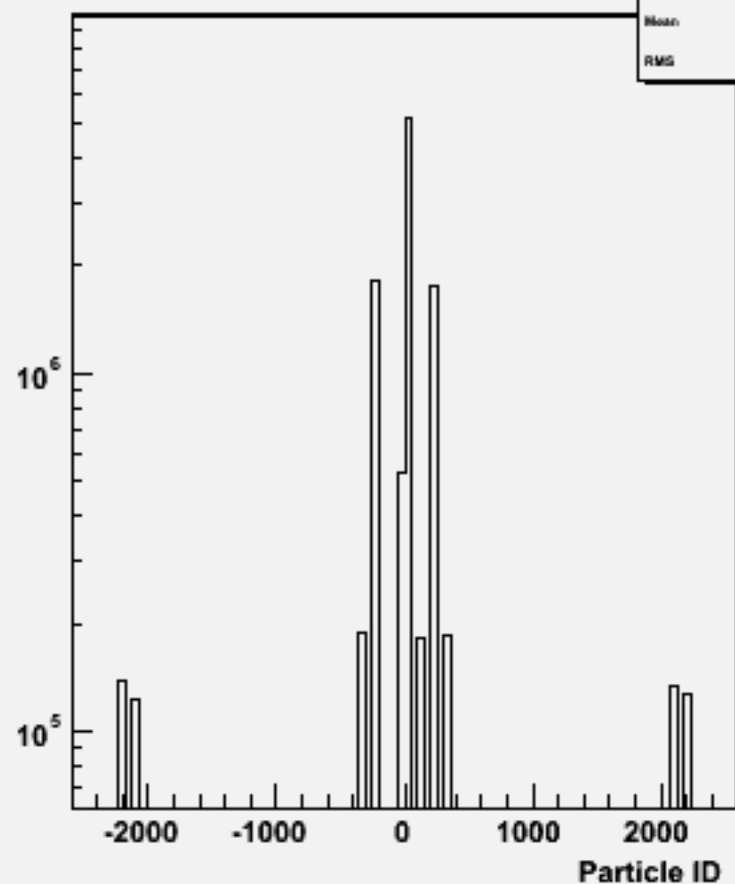
Particle ID : w100748 e1e1n3e3du_o
