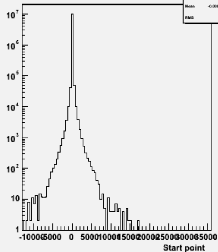
Start point Z : w100748 e1e1n3e3du_o
