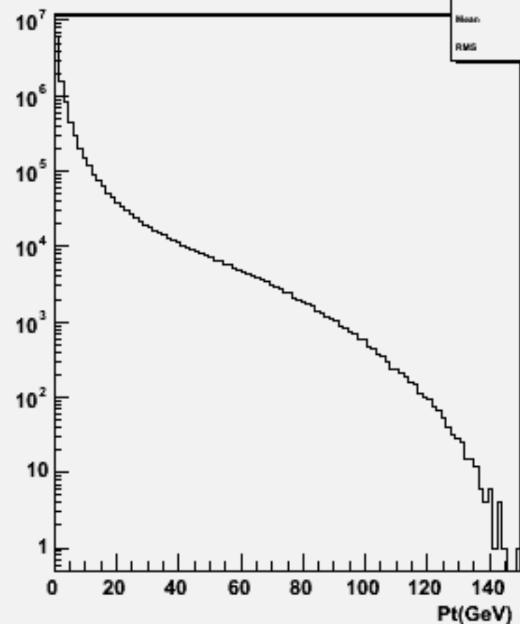
Particle Pt : w100748 e1e1n3e3du_o
