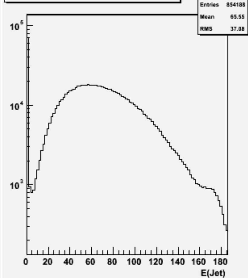
Jet energies(All jets)w100748 e1e1n3e3du_o
