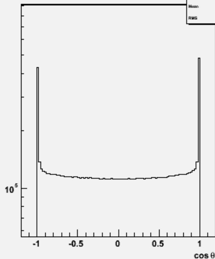
Particle \cos\theta : w100748 e1e1n3e3du_o
