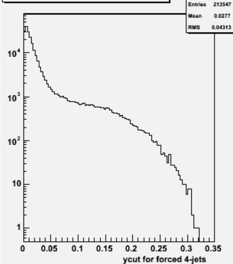
Ycut for 4-jets :w100748 e1e1n3e3du_o
