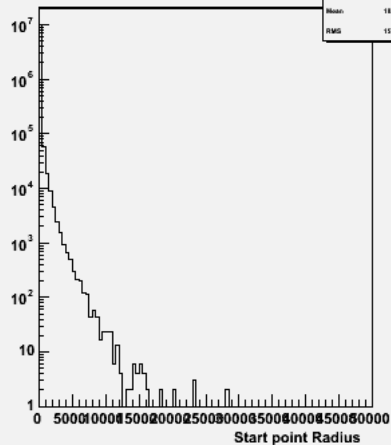
Start point R : w100748 e1e1n3e3du_o
