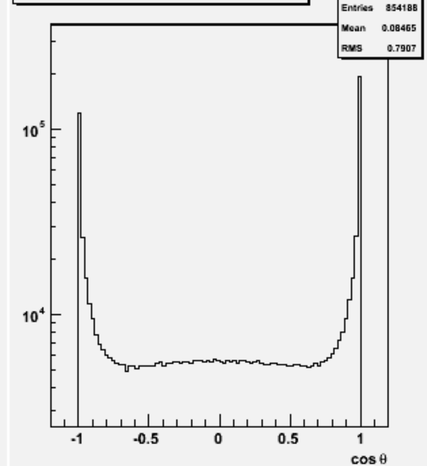
Jet cos \theta (All jets)w100748 e1e1n3e3du_o
