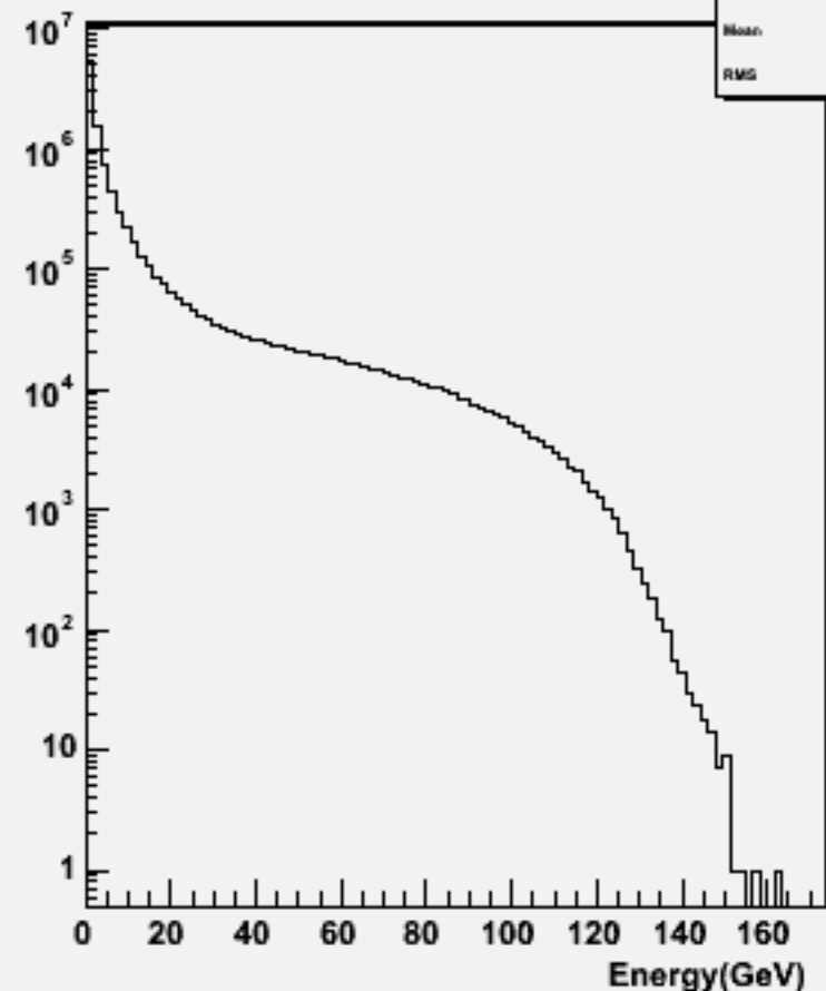
Particle Energy : w100748 e1e1n3e3du_o
