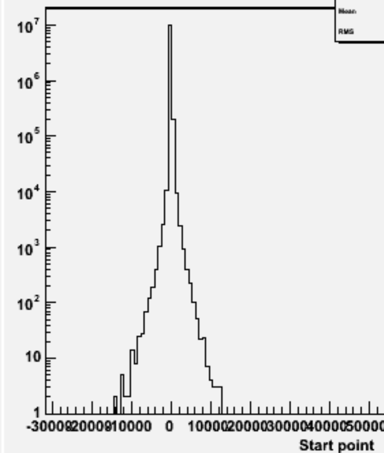
Start point Z : w100747 e1e1n3e3du_o
