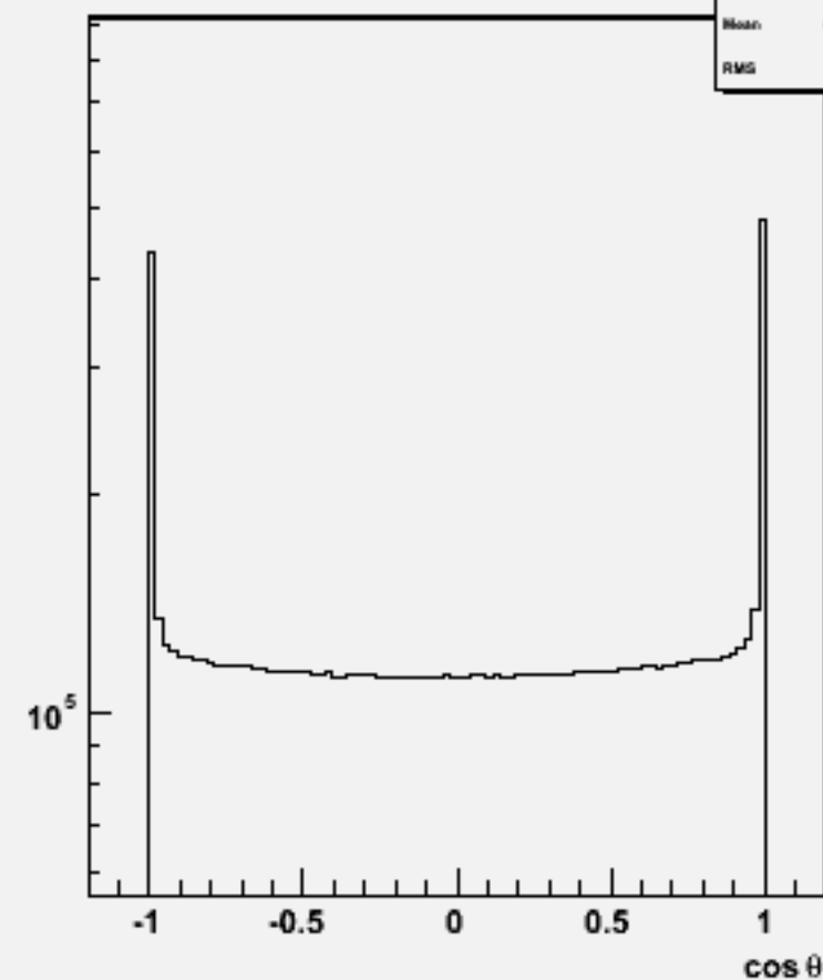
Particle \cos\theta : w100747 e1e1n3e3du_o
