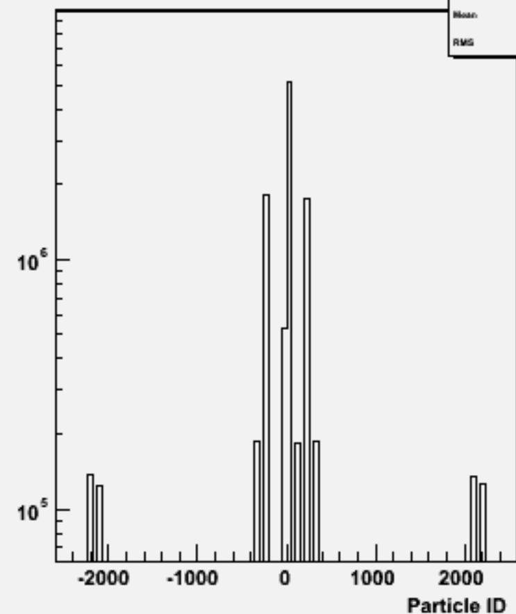
Particle ID : w100747 e1e1n3e3du_o
