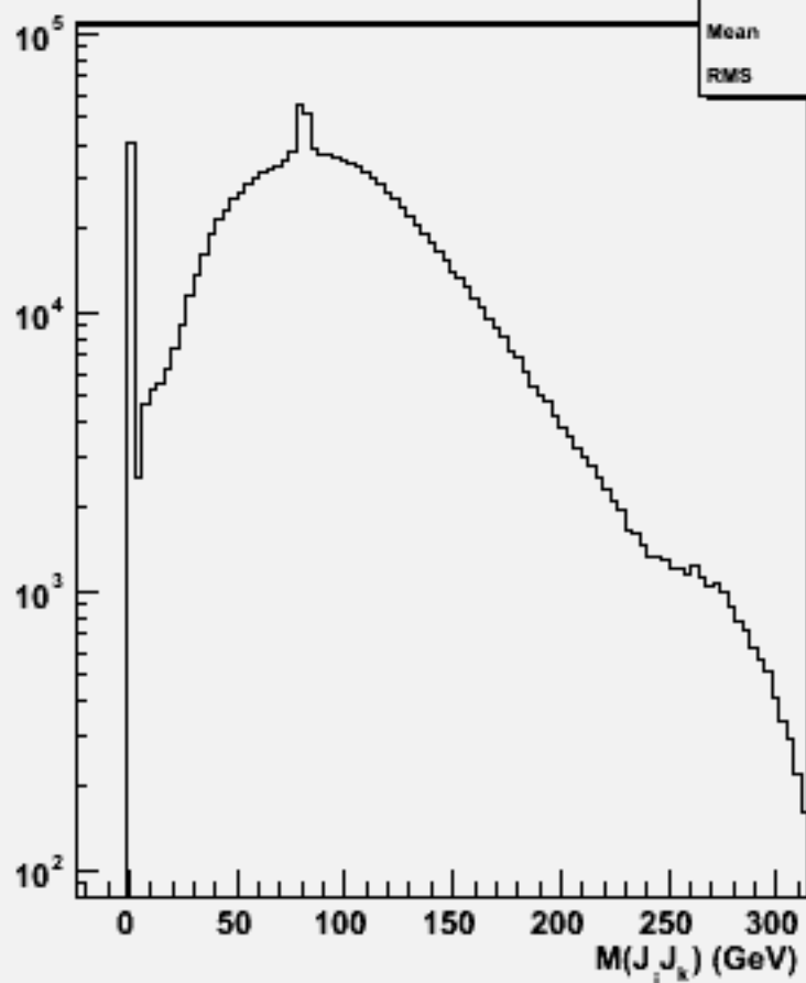
2jets mass(All comb)w100747 e1e1n3e3du_o
