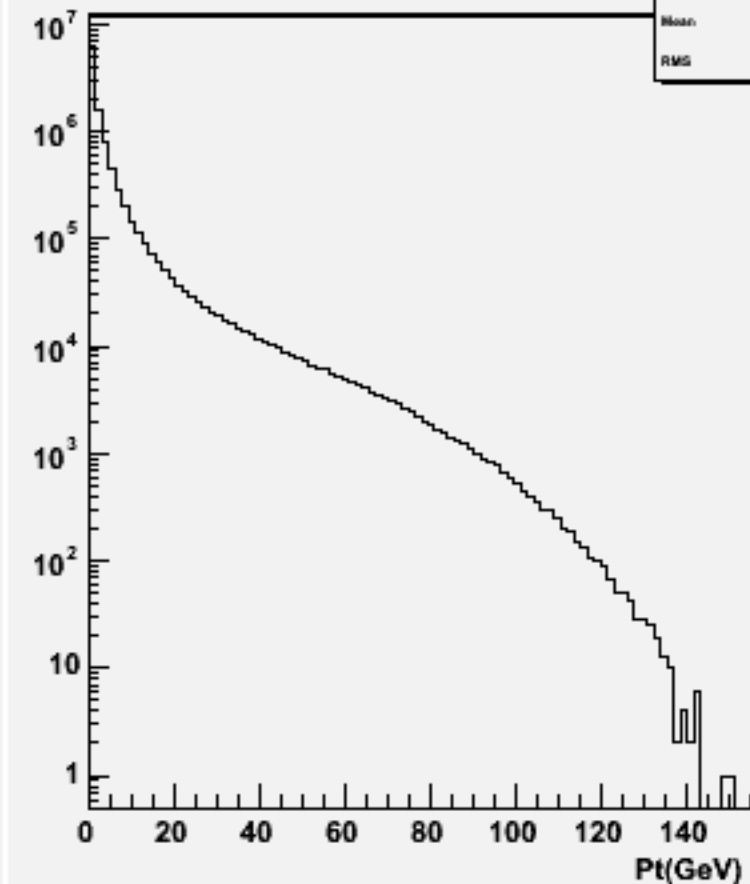
Particle Pt : w100747 e1e1n3e3du_o
