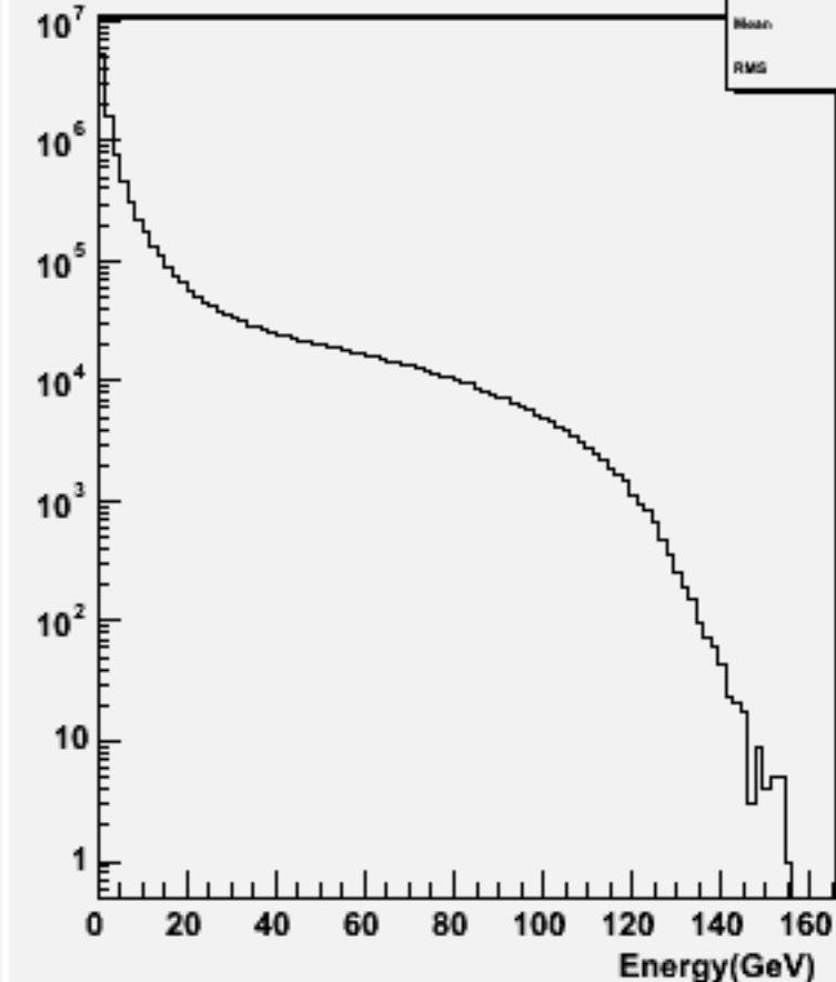
Particle Energy : w100747 e1e1n3e3du_o
