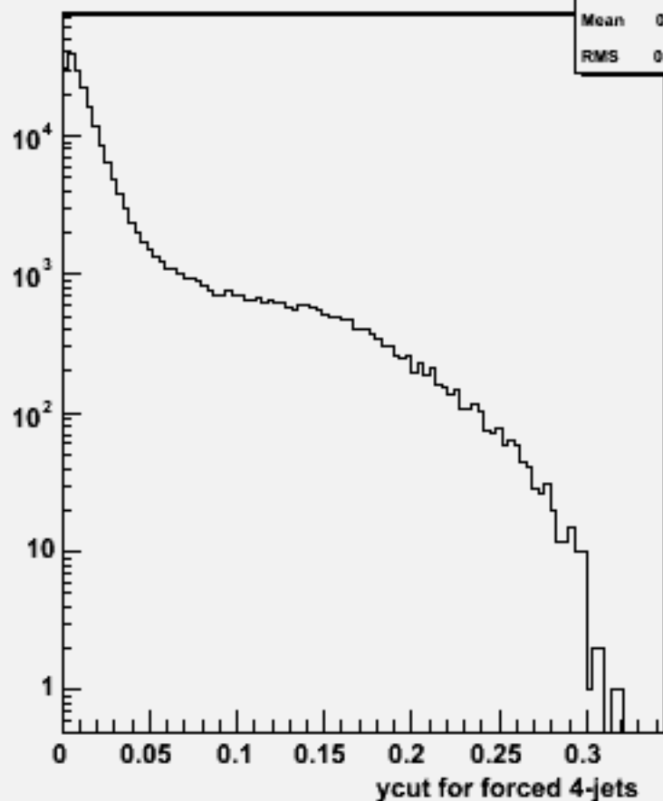
Ycut for 4-jets :w100747 e1e1n3e3du_o
