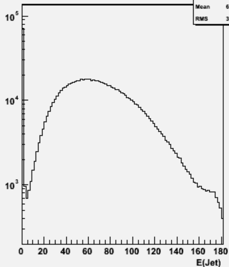
Jet energies(All jets)w100747 e1e1n3e3du_o
