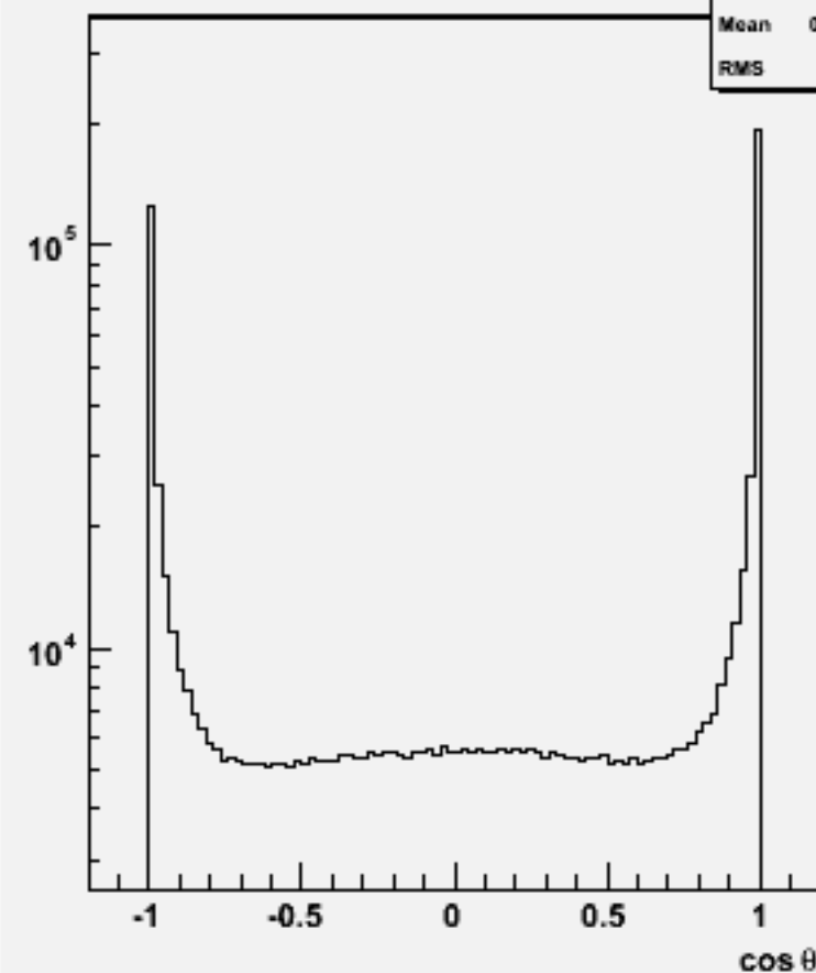
Jet cos \theta (All jets)w100747 e1e1n3e3du_o
