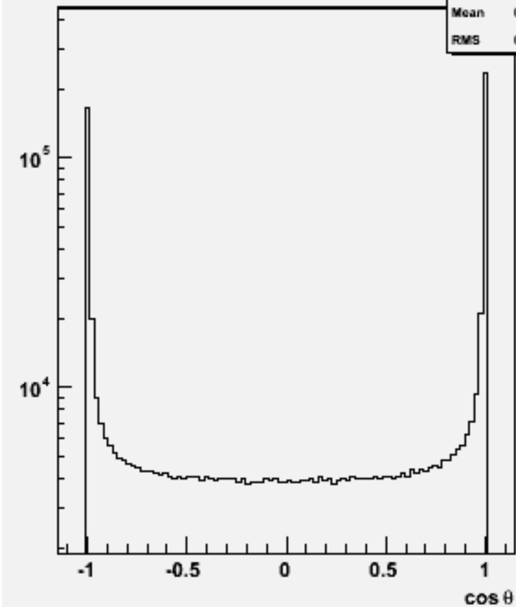
Jet cos \theta (All jets)w100745 e1e1n3e3e3n3_o
