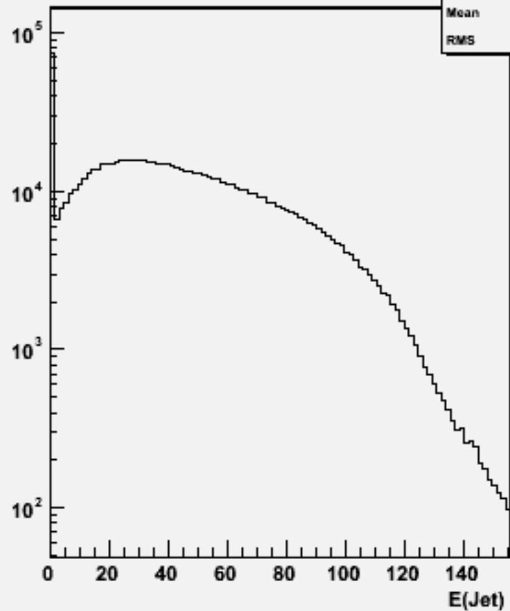
Jet energies(All jets)w100745 e1e1n3e3e3n3_o
