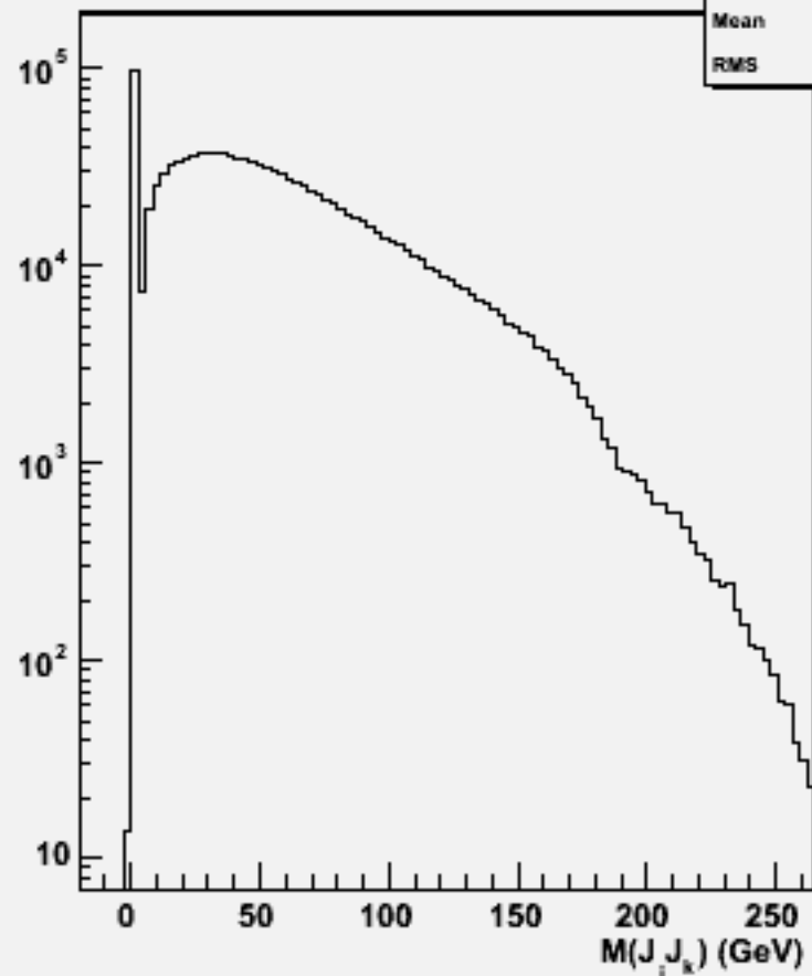
2jets mass(All comb)w100745 e1e1n3e3e3n3_o
