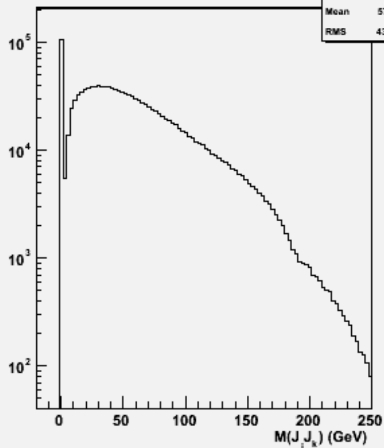
2jets mass(All comb)w100744 e1e1n3e3e3n3_o
