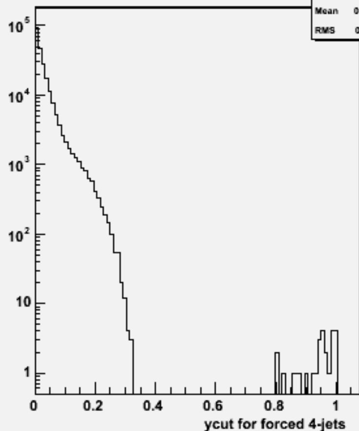
Ycut for 4-jets :w100744 e1e1n3e3e3n3_o
