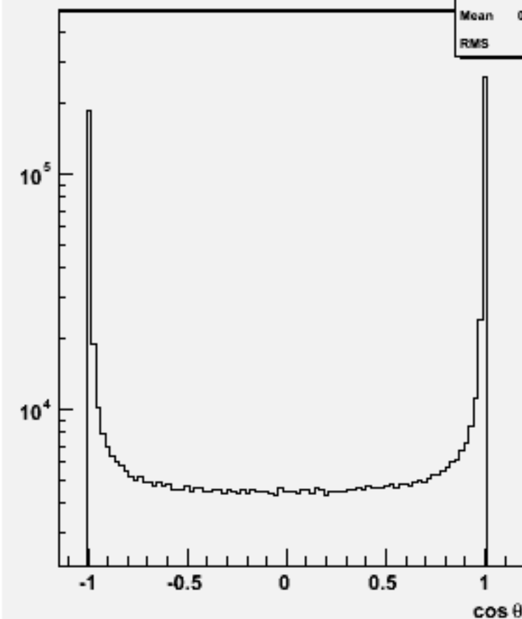
Jet cos \theta (All jets)w100744 e1e1n3e3e3n3_o
