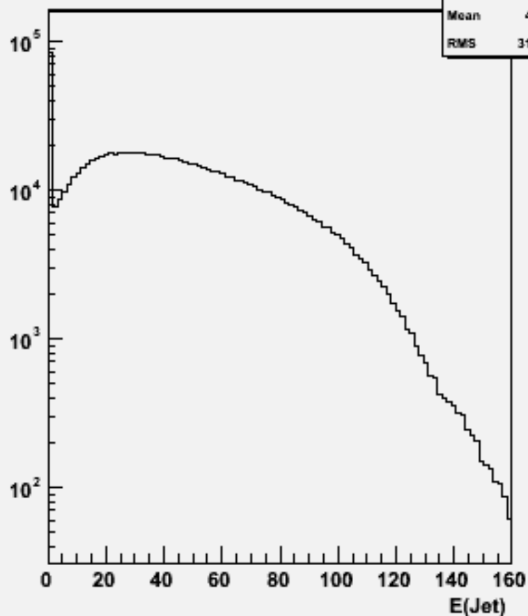
Jet energies(All jets)w100744 e1e1n3e3e3n3_o
