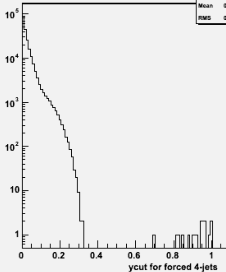
Ycut for 4-jets :w100743 e1e1n3e3e3n3_o
