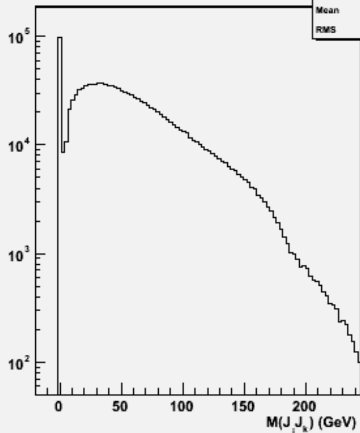
2jets mass(All comb)w100743 e1e1n3e3e3n3_o
