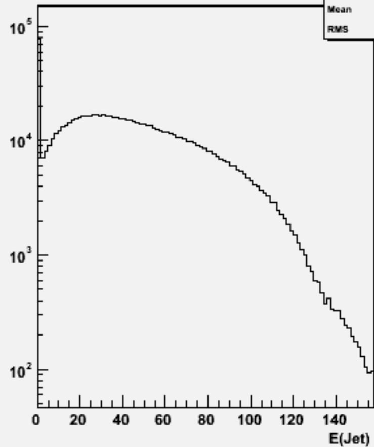
Jet energies(All jets)w100743 e1e1n3e3e3n3_o
