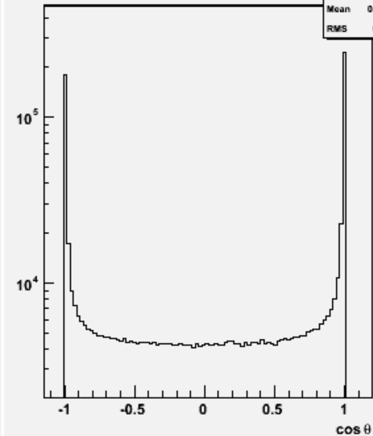
Jet cos \theta (All jets)w100743 e1e1n3e3e3n3_o
