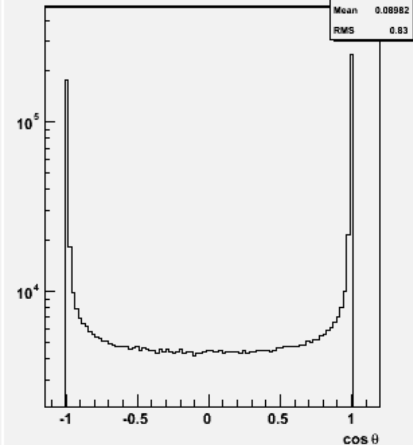
Jet cos theta (All jets)w100742 e1e1n3e3e2n2_o
