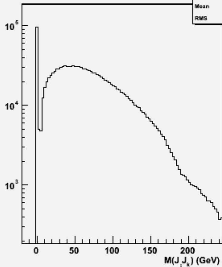
2jets mass(All comb)w100742 e1e1n3e3e2n2_o
