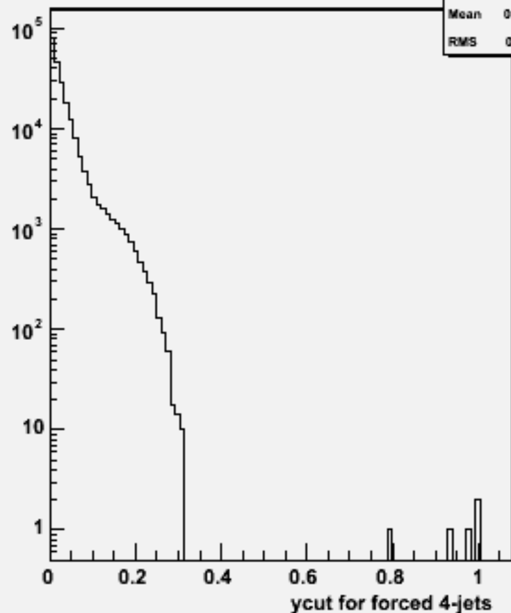
Ycut for 4-jets :w100742 e1e1n3e3e2n2_o
