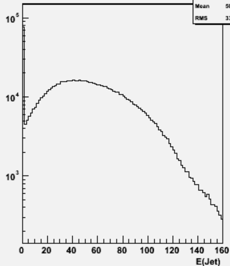
Jet energies(All jets)w100742 e1e1n3e3e2n2_o
