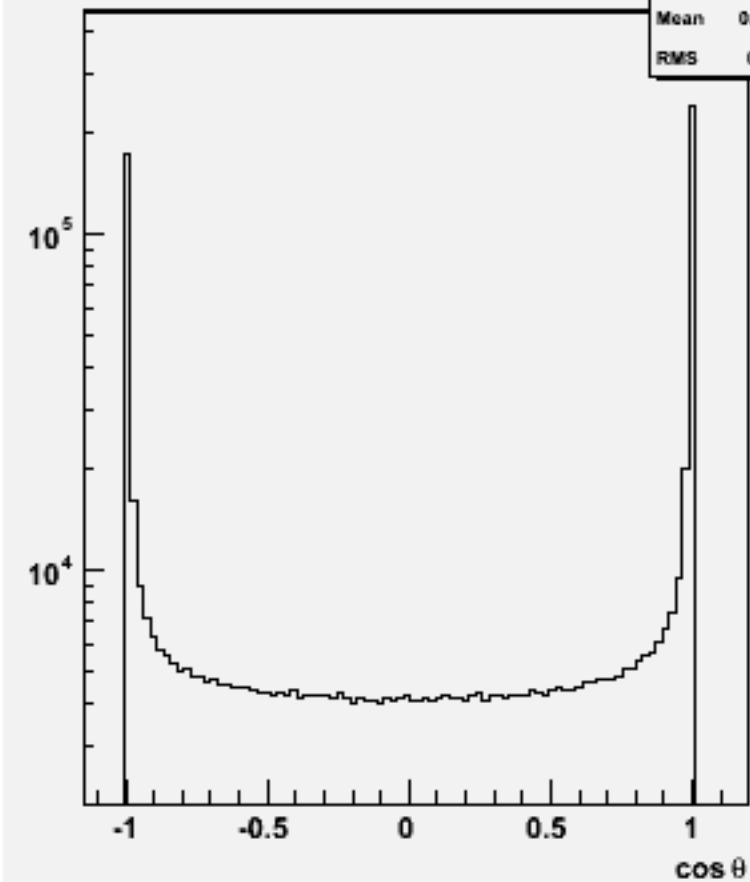
Jet cos \theta (All jets)w100741 e1e1n3e3e2n2_o
