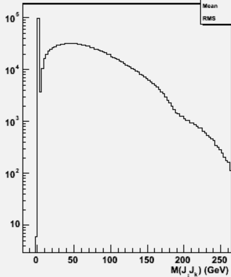
2jets mass(All comb)w100741 e1e1n3e3e2n2_o
