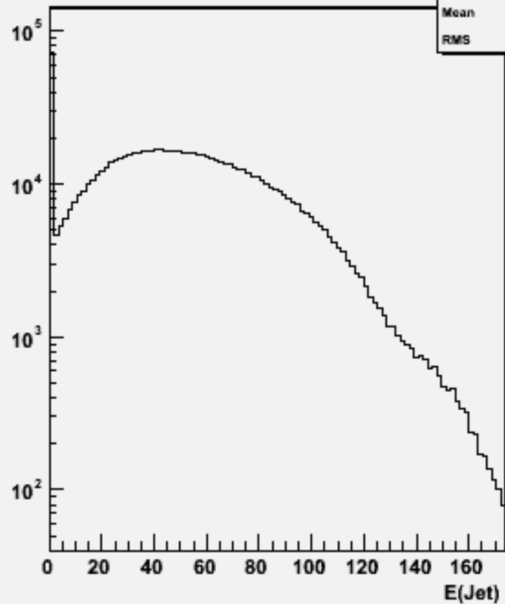
Jet energies(All jets)w100741 e1e1n3e3e2n2_o
