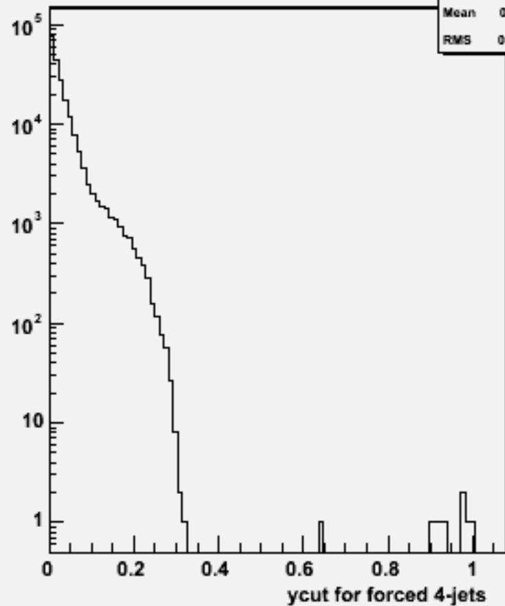
Ycut for 4-jets :w100741 e1e1n3e3e2n2_o
