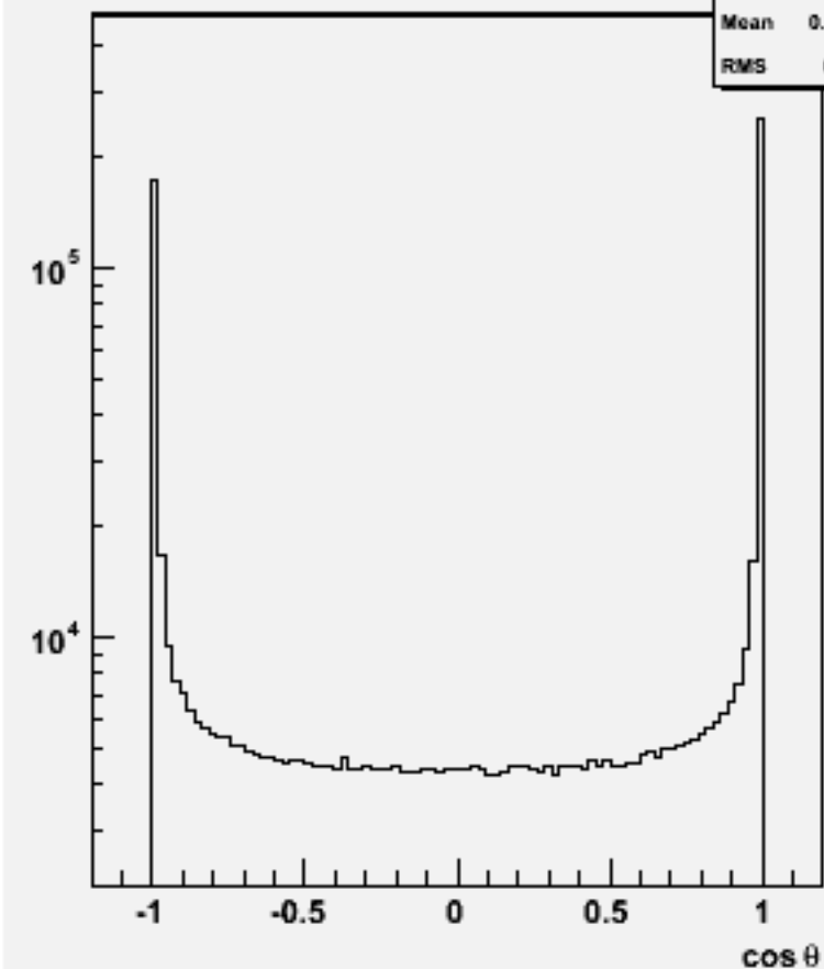
Jet cos \theta (All jets)w100738 e1e1n3e3e1n1_o
