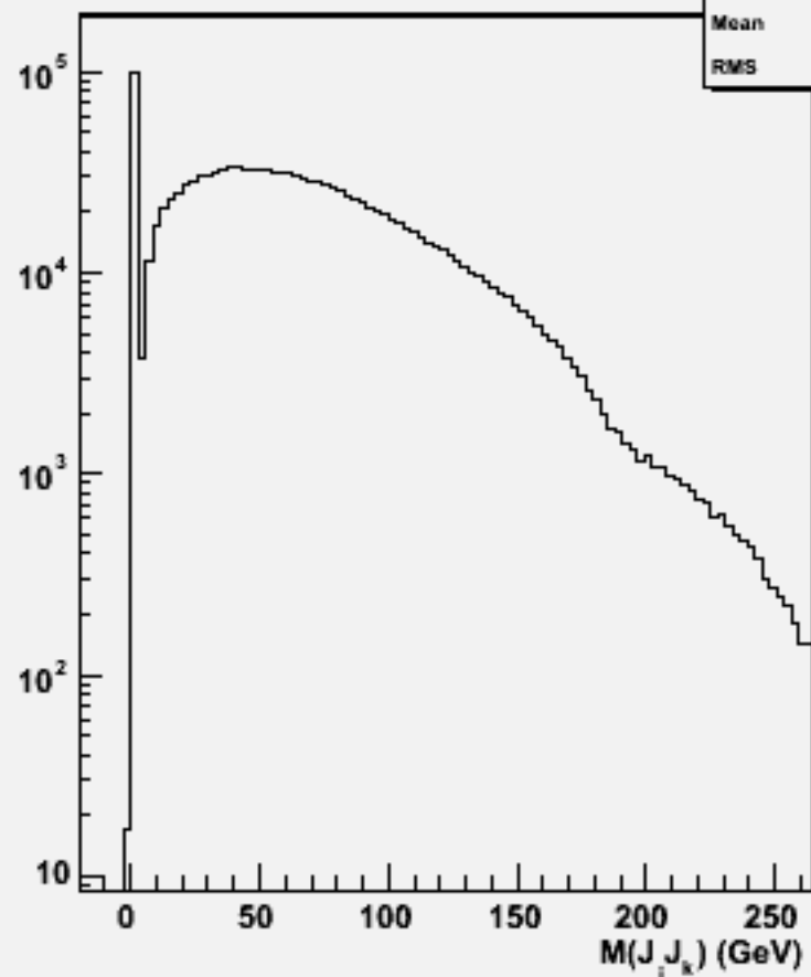
2jets mass(All comb)w100738 e1e1n3e3e1n1_o
