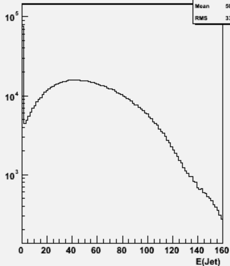
Jet energies(All jets)w100738 e1e1n3e3e1n1_o
