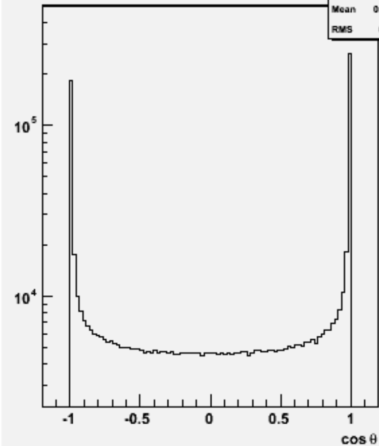
Jet cos \theta (All jets)w100736 e1e1n3e3e1n1_o
