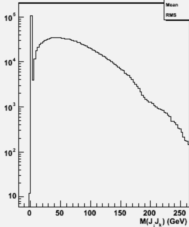
2jets mass(All comb)w100736 e1e1n3e3e1n1_o
