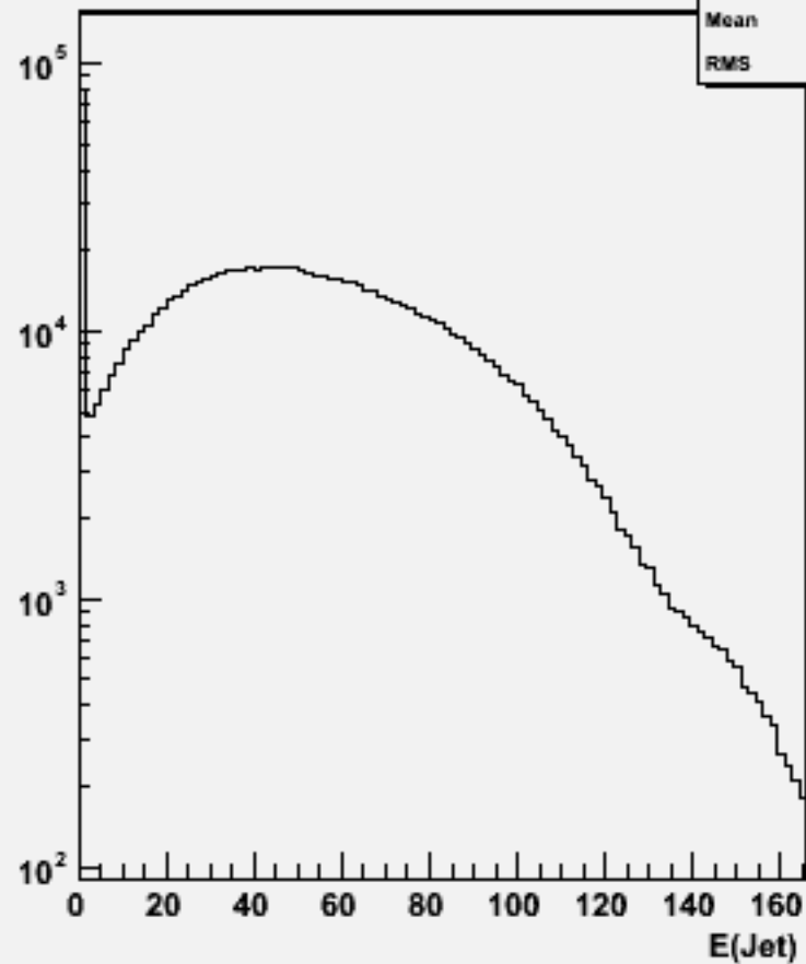
Jet energies(All jets)w100736 e1e1n3e3e1n1_o
