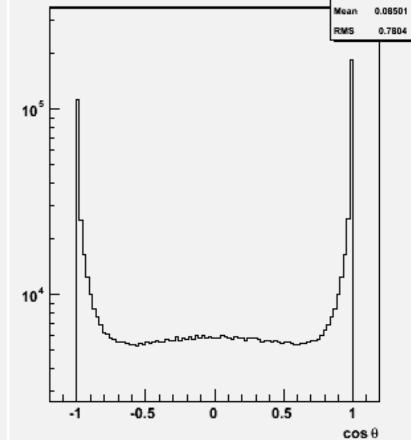
Jet cos \theta (All jets)w100734 e1e1n2e2sc_o
