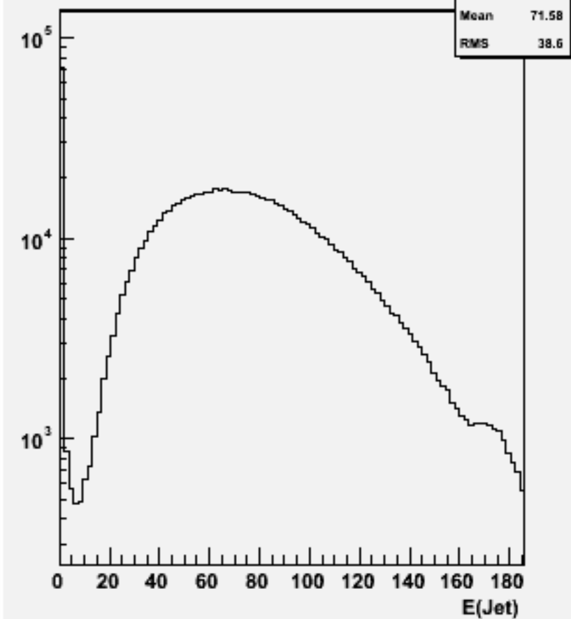
Jet energies(All jets)w100734 e1e1n2e2sc_o
