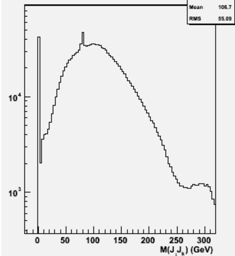
2jets mass(All comb)w100734 e1e1n2e2sc_o
