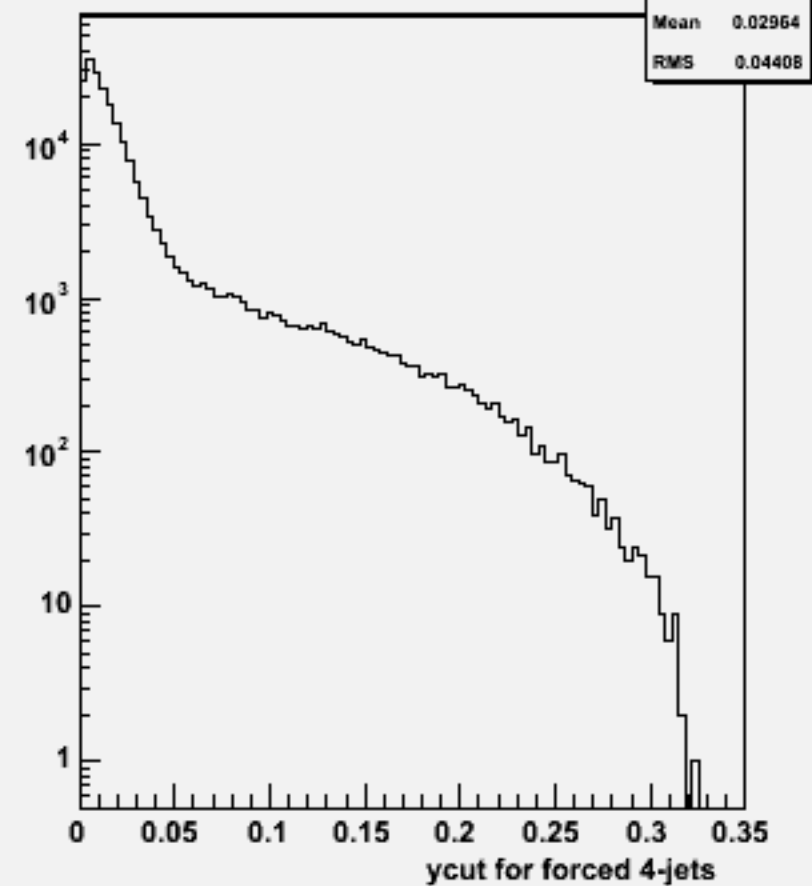
Ycut for 4-jets :w100734 e1e1n2e2sc_o
