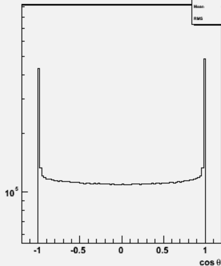
Particle \cos\theta : w100733 e1e1n2e2sc_o
