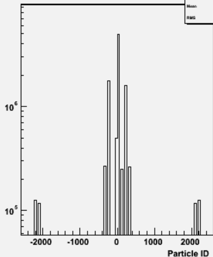
Particle ID : w100733 e1e1n2e2sc_o
