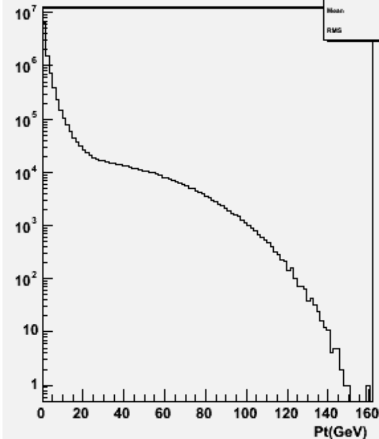
Particle Pt : w100733 e1e1n2e2sc_o
