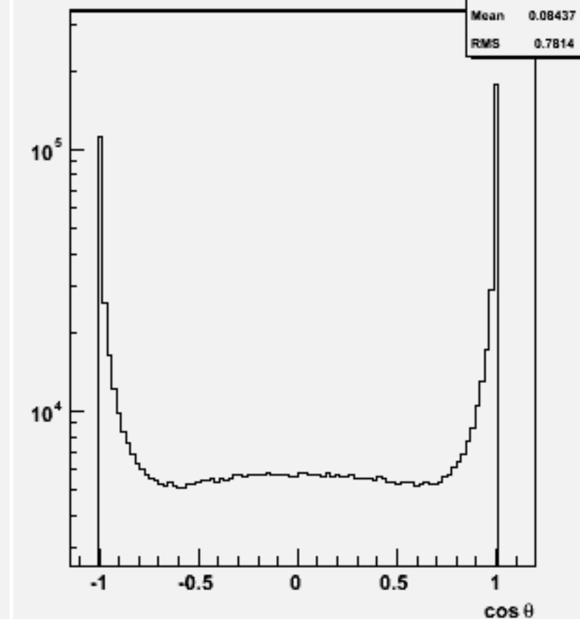
Jet cos \theta (All jets)w100733 e1e1n2e2sc_o
