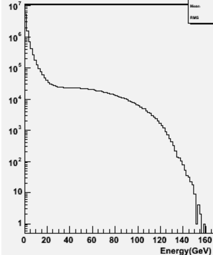
Particle Energy : w100733 e1e1n2e2sc_o
