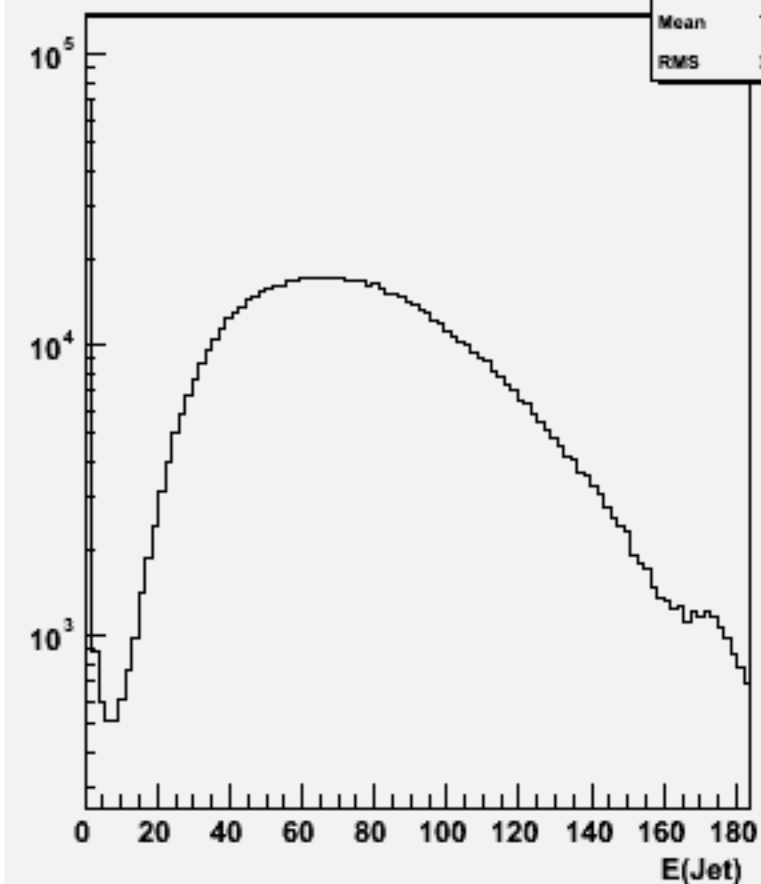
Jet energies(All jets)w100733 e1e1n2e2sc_o
