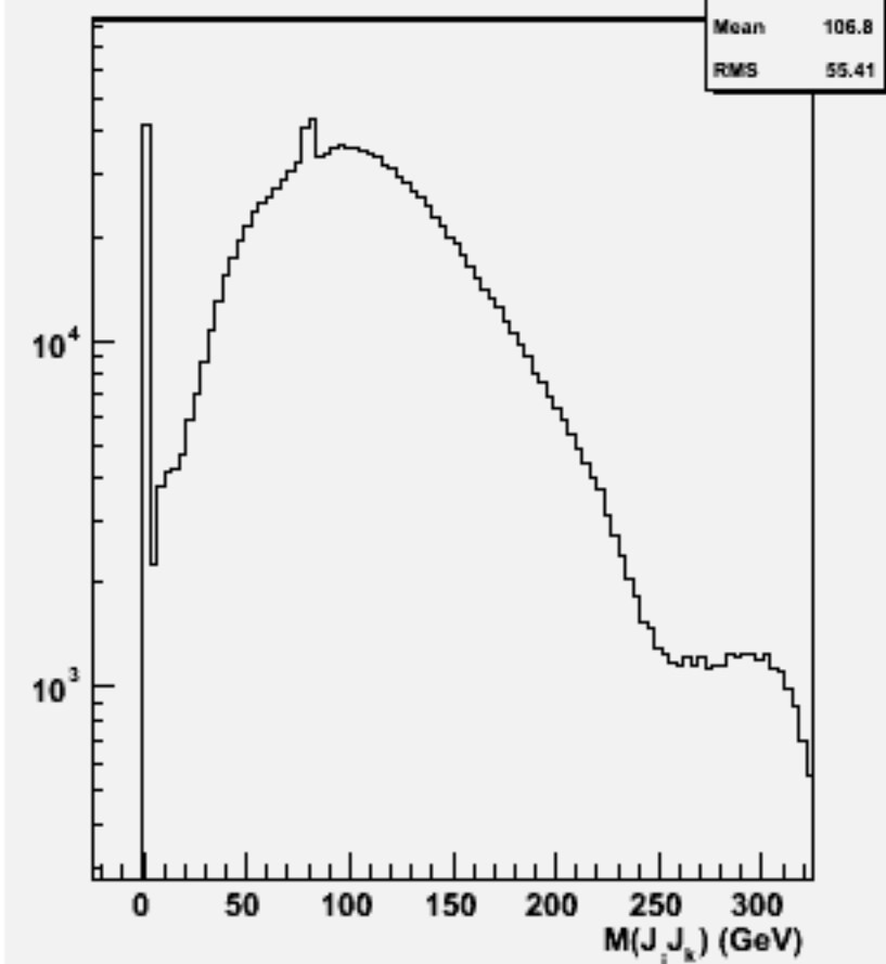
2jets mass(All comb)w100733 e1e1n2e2sc_o
