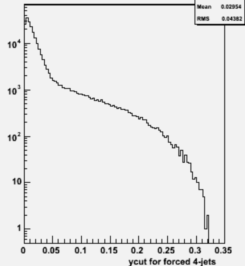
Ycut for 4-jets :w100733 e1e1n2e2sc_o
