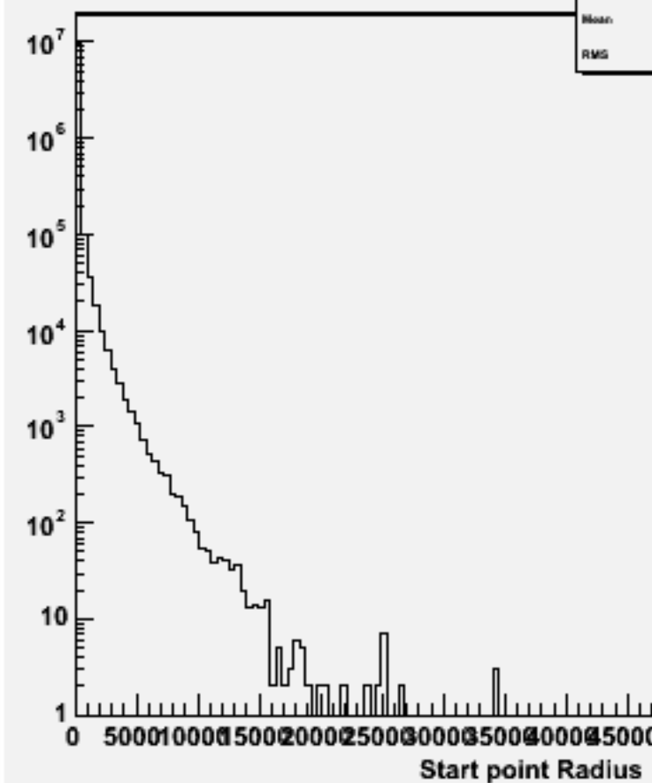
Start point R : w100733 e1e1n2e2sc_o
