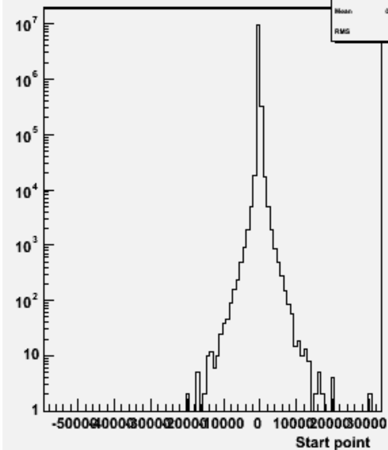
Start point Z : w100733 e1e1n2e2sc_o
