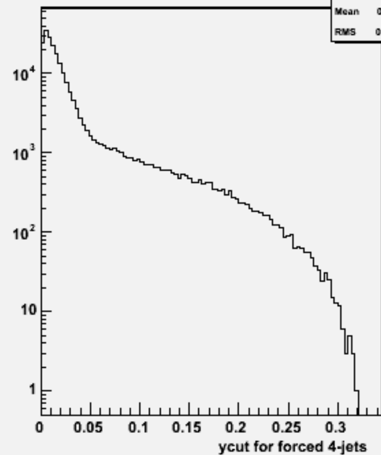
Ycut for 4-jets :w100732 e1e1n2e2sc_o
