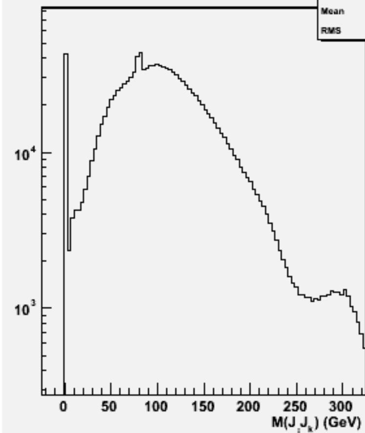
2jets mass(All comb)w100732 e1e1n2e2sc_o
