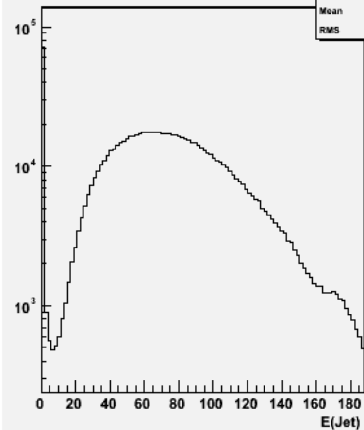
Jet energies(All jets)w100732 e1e1n2e2sc_o
