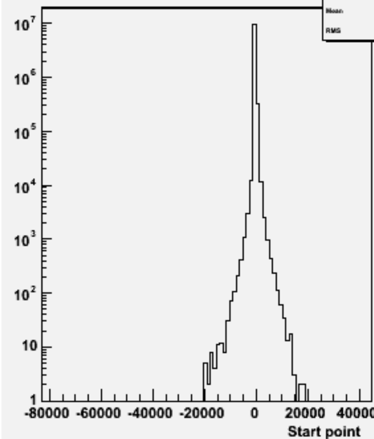
Start point Z : w100732 e1e1n2e2sc_o
