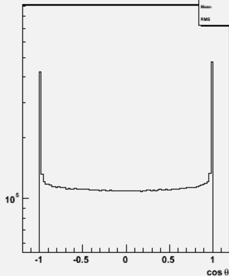
Particle \cos\theta : w100732 e1e1n2e2sc_o
