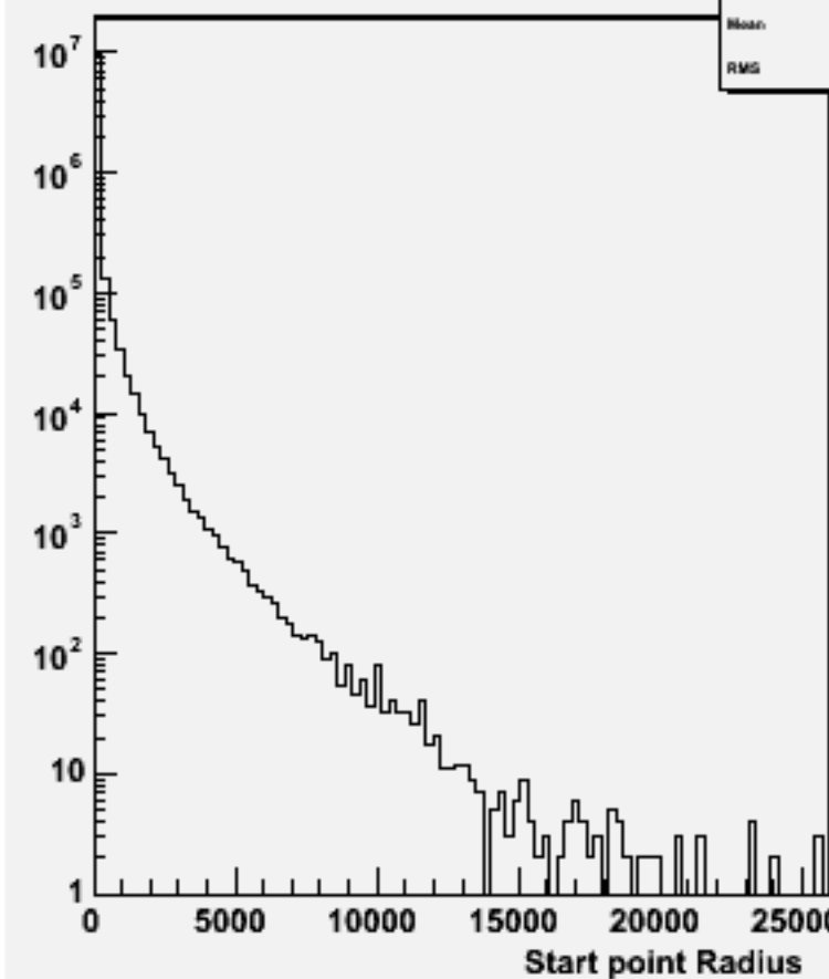
Start point R : w100732 e1e1n2e2sc_o
