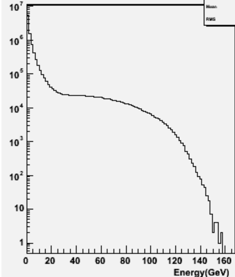
Particle Energy : w100732 e1e1n2e2sc_o
