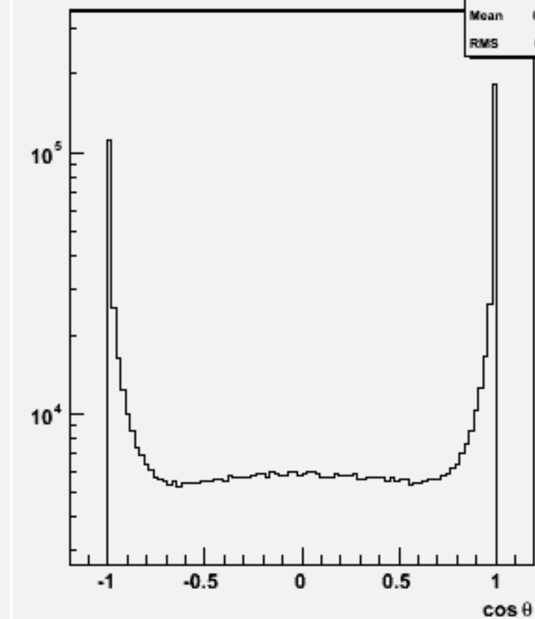
Jet cos \theta (All jets)w100732 e1e1n2e2sc_o
