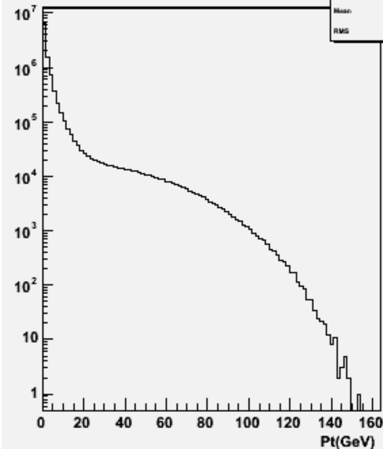
Particle Pt : w100732 e1e1n2e2sc_o
