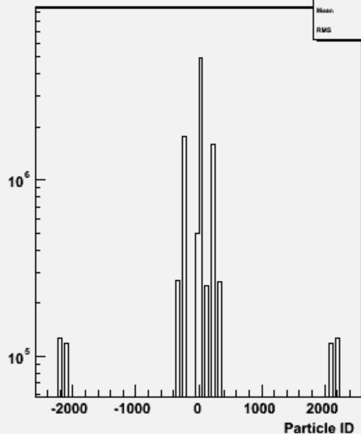
Particle ID : w100732 e1e1n2e2sc_o
