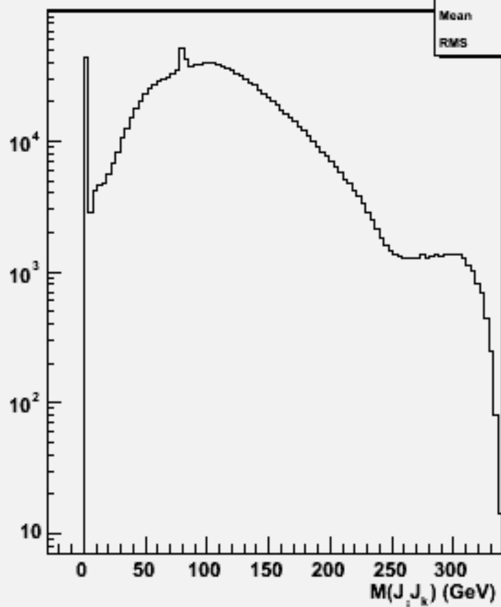
2jets mass(All comb)w100730 e1e1n2e2du_o
