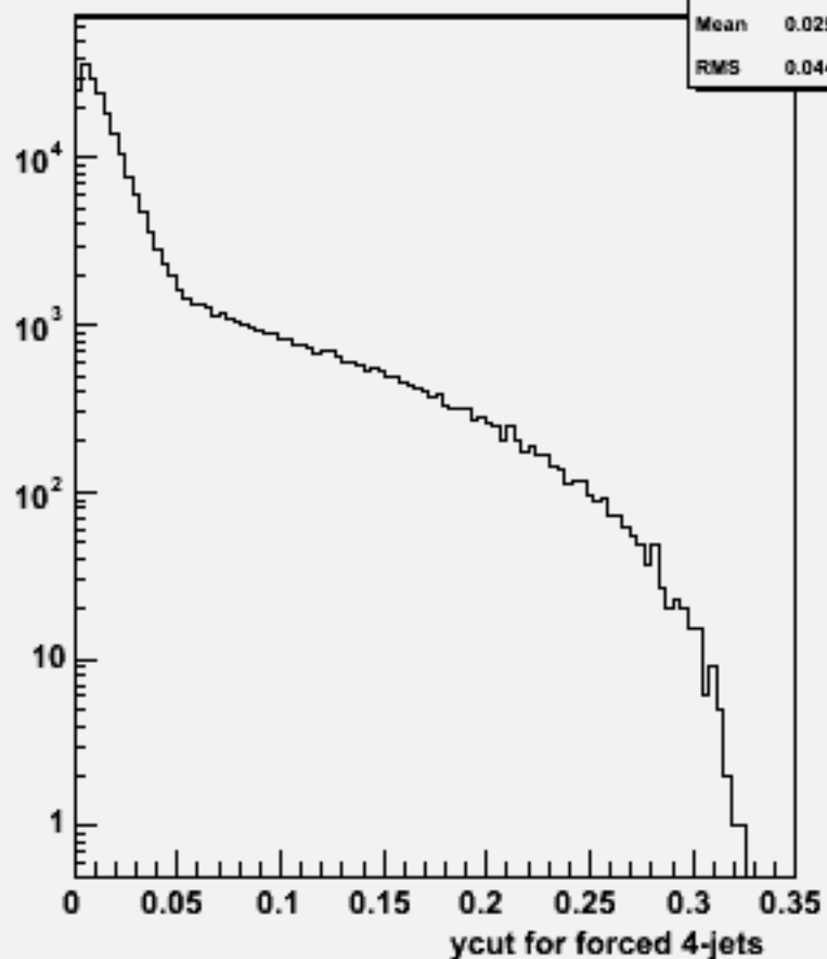
Ycut for 4-jets :w100730 e1e1n2e2du_o
