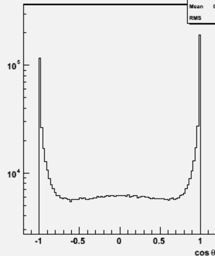
Jet cos \theta (All jets)w100730 e1e1n2e2du_o
