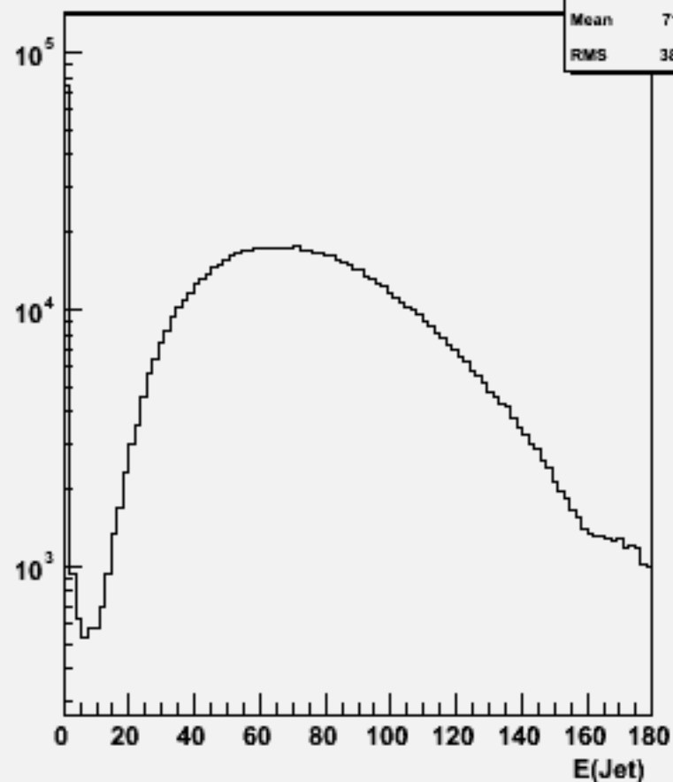
Jet energies(All jets)w100730 e1e1n2e2du_o
