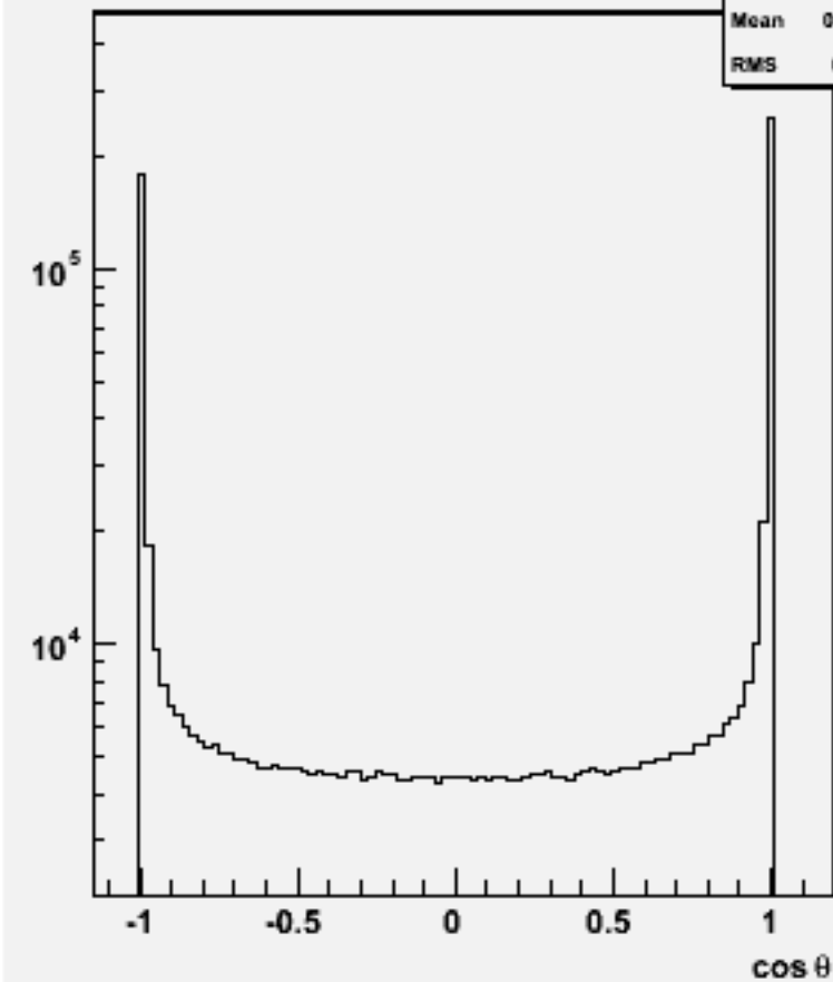
Jet cos \theta (All jets)w100726 e1e1n2e2e3n3_o
