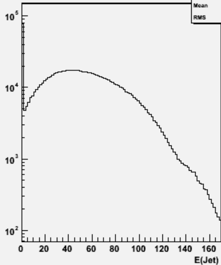
Jet energies(All jets)w100726 e1e1n2e2e3n3_o
