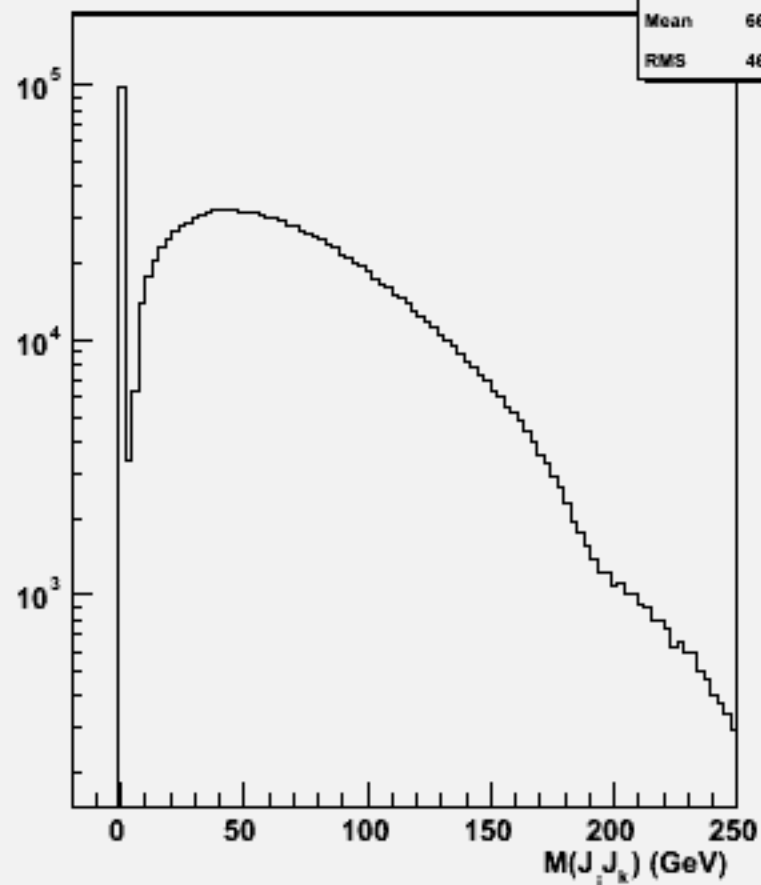
2jets mass(All comb)w100726 e1e1n2e2e3n3_o
