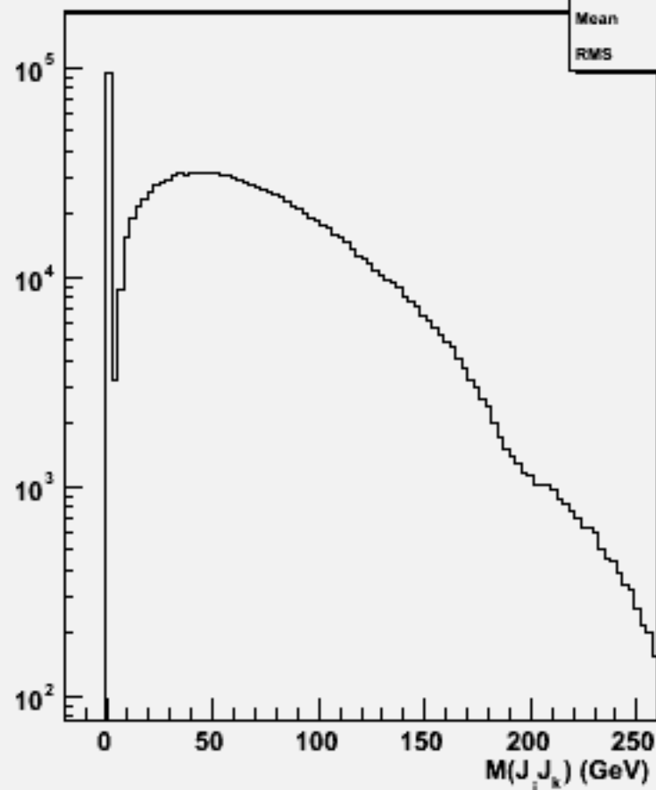
2jets mass(All comb)w100725 e1e1n2e2e3n3_o
