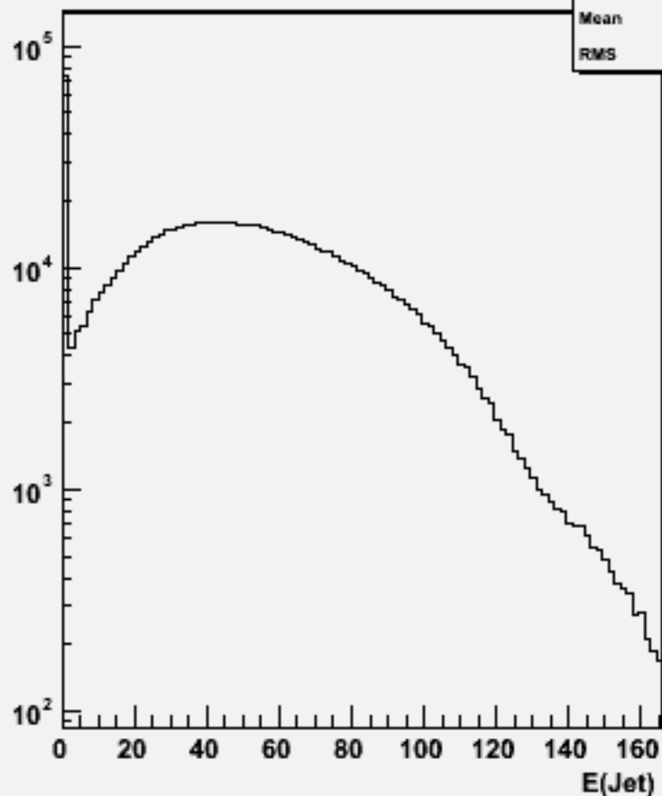
Jet energies(All jets)w100725 e1e1n2e2e3n3_o
