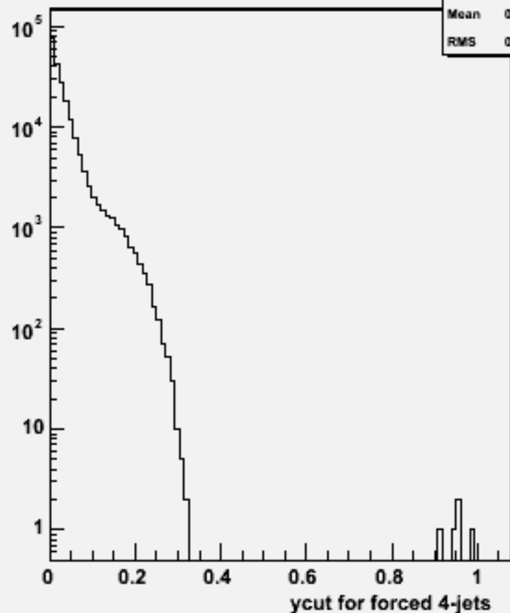
Ycut for 4-jets :w100725 e1e1n2e2e3n3_o
