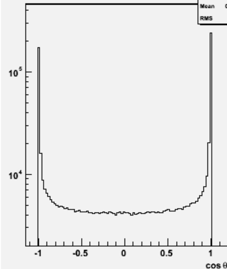
Jet cos \theta (All jets)w100725 e1e1n2e2e3n3_o
