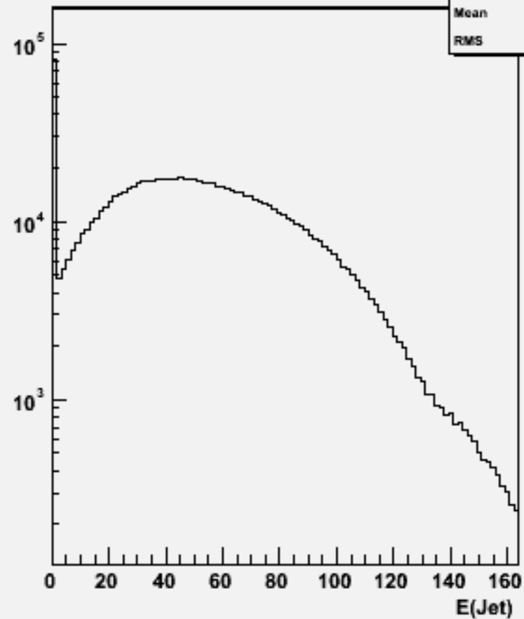
Jet energies(All jets)w100724 e1e1n2e2e3n3_o
