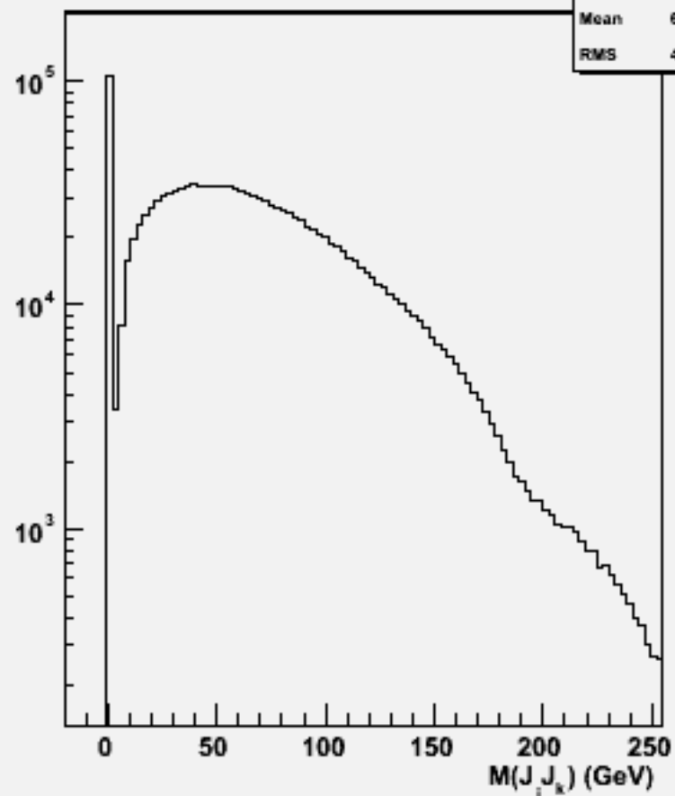
2jets mass(All comb)w100724 e1e1n2e2e3n3_o
