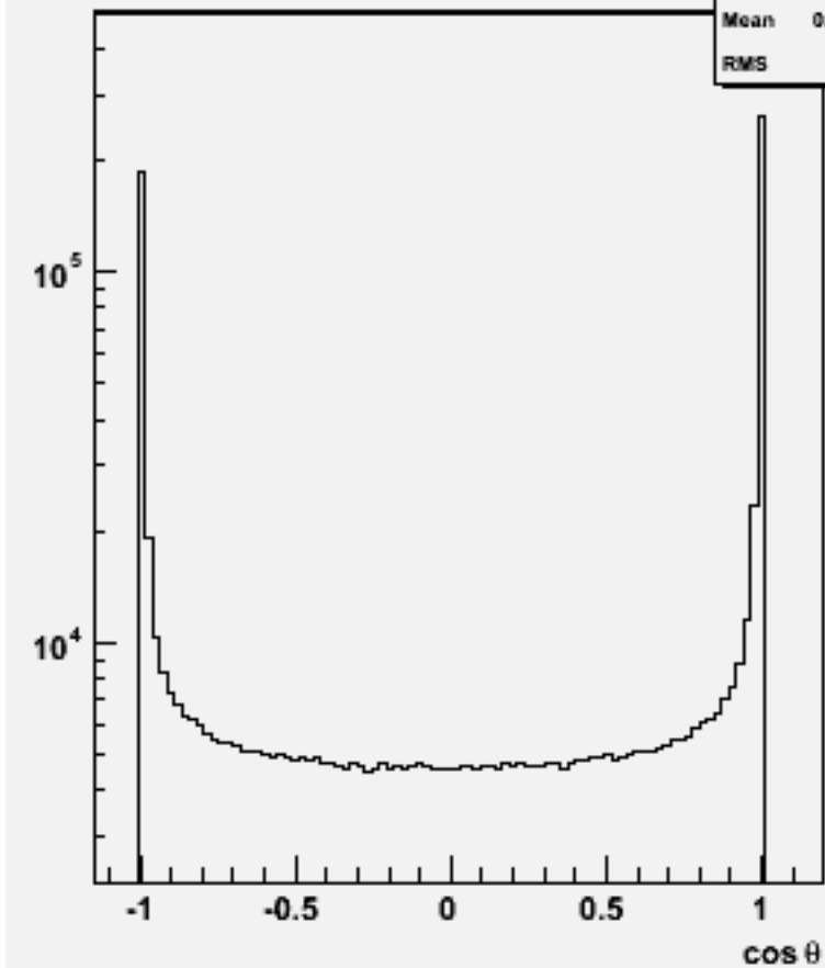
Jet cos \theta (All jets)w100724 e1e1n2e2e3n3_o
