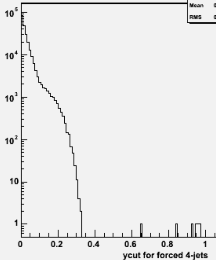
Ycut for 4-jets :w100724 e1e1n2e2e3n3_o
